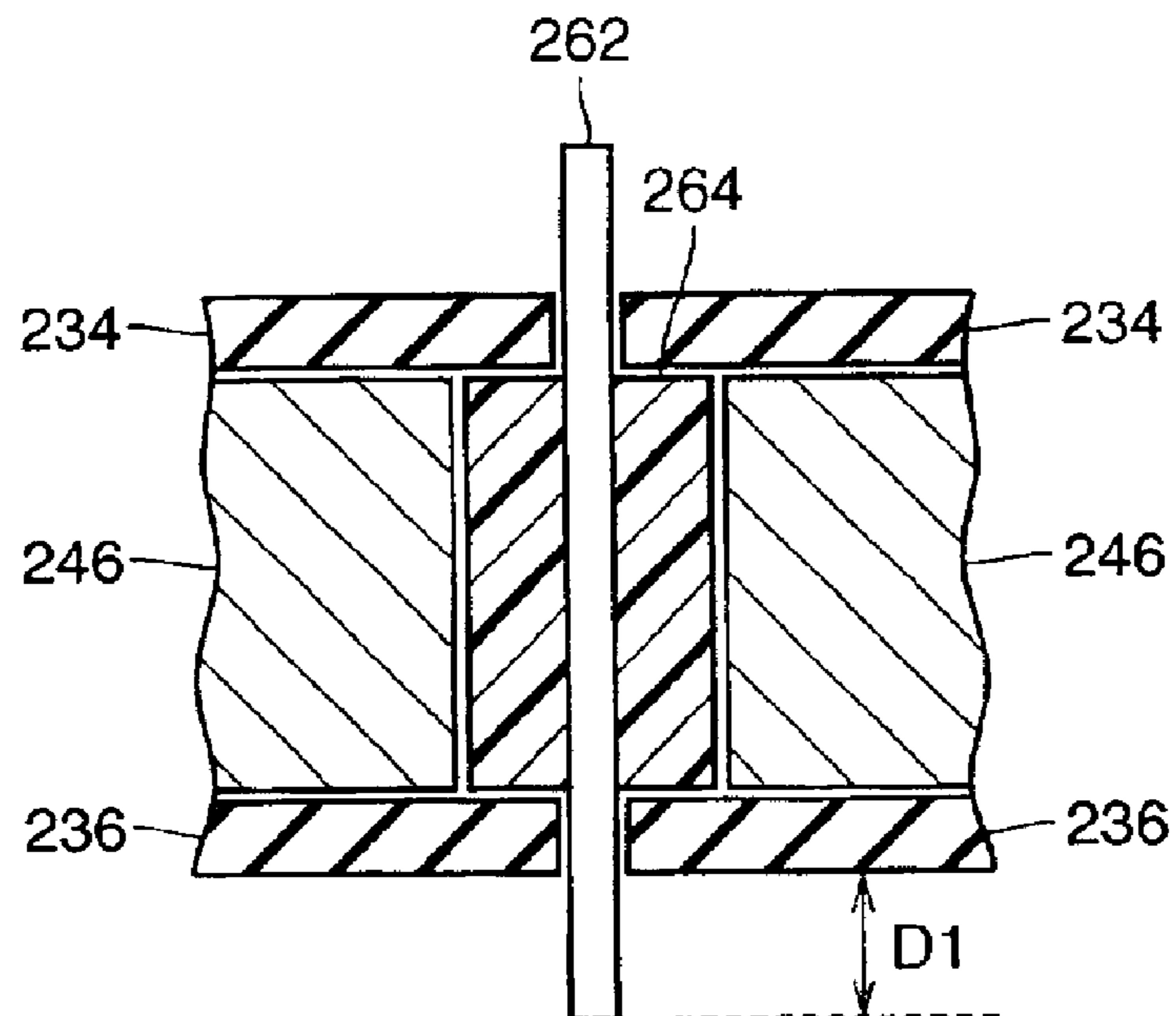
FIG. 13 PROR ART
