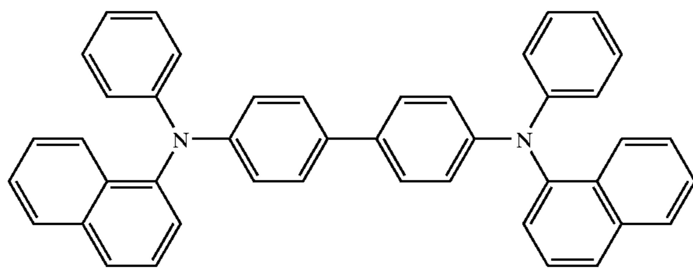
\alpha -NPD
