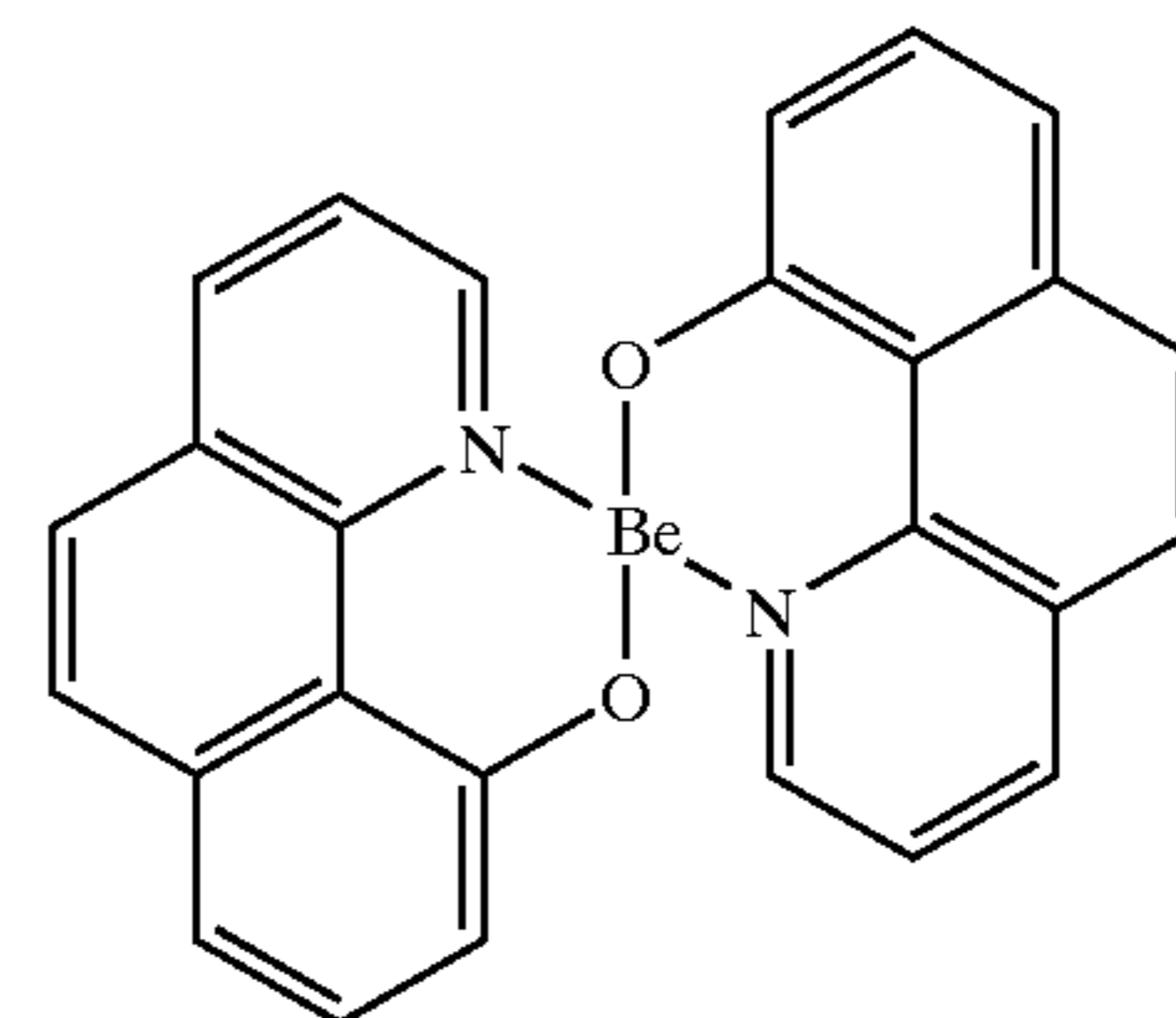
Bebq
