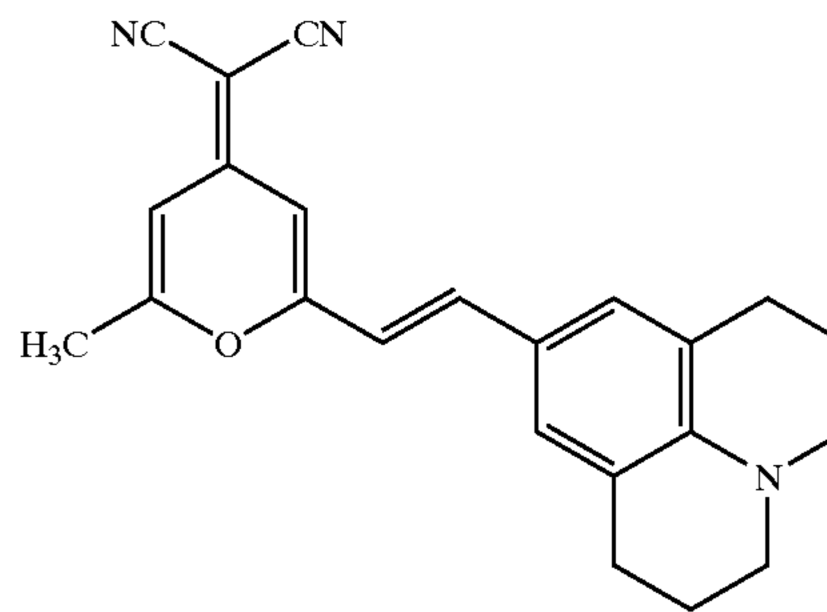
DCM-II
