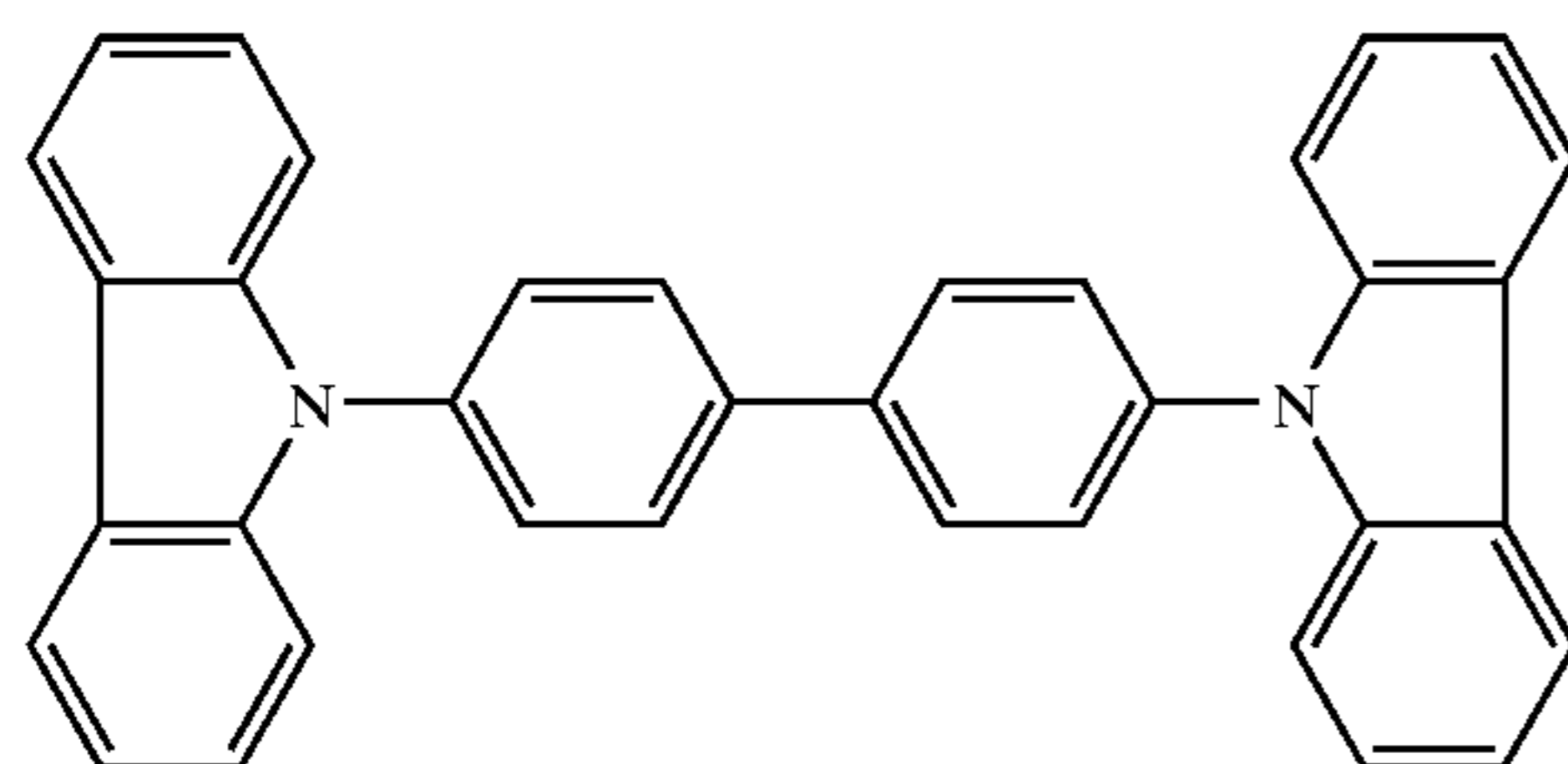
CBP
