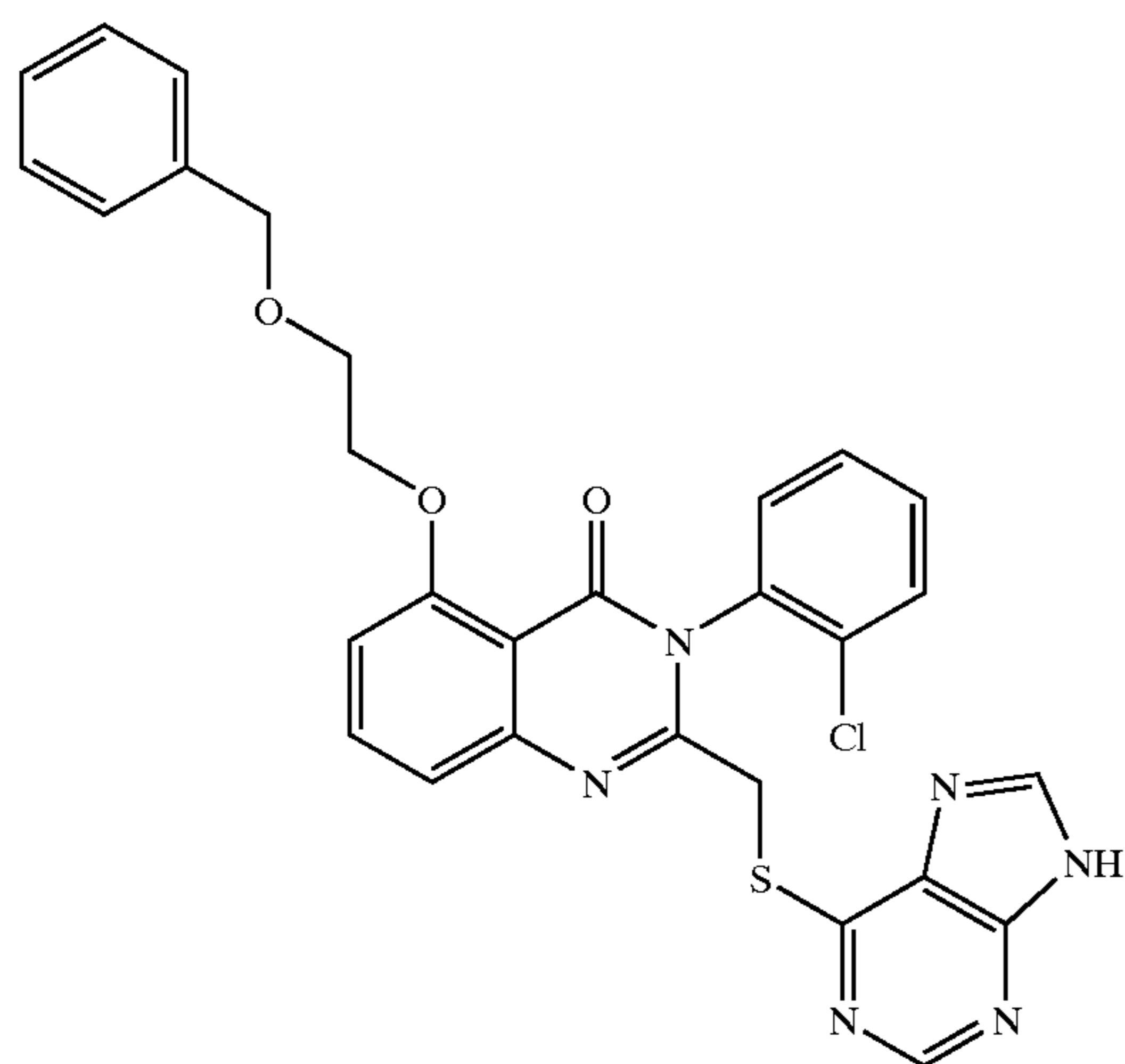
5-(2-Benzyloxyethoxy)-3-(2-chlorophenyl)-2-(9H-purin-6-ylsulfanylmethyl)-3H-quinazolin-4-one (D-078)
