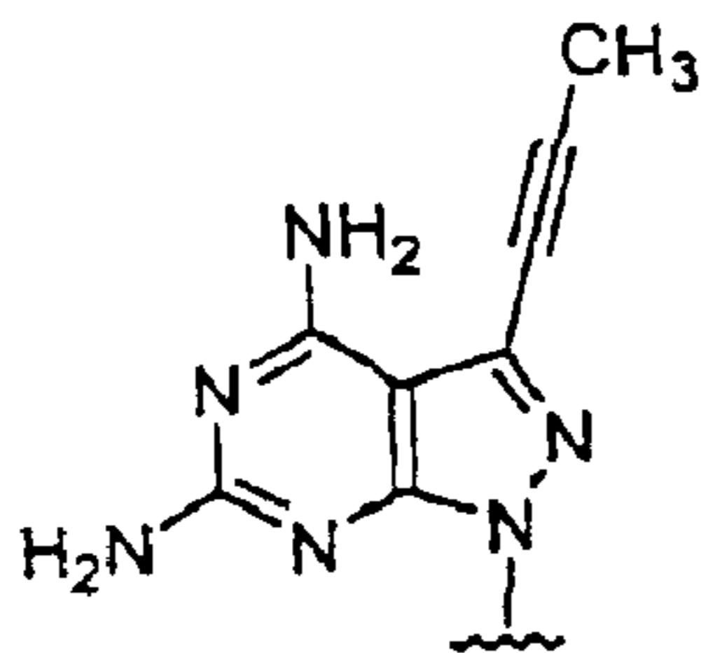
(NH 2 ) 2 PPPA
