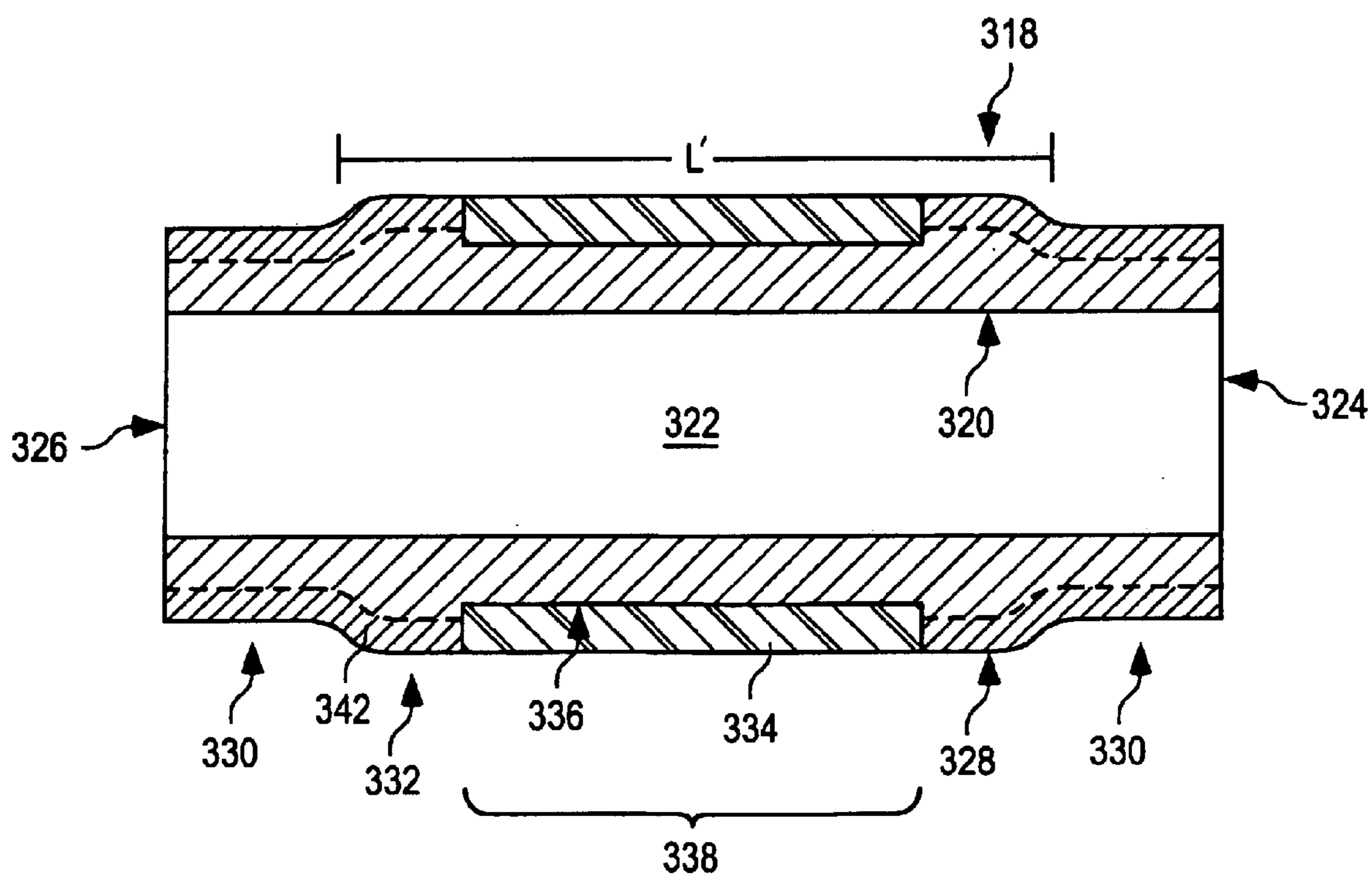
FIG. 3B
