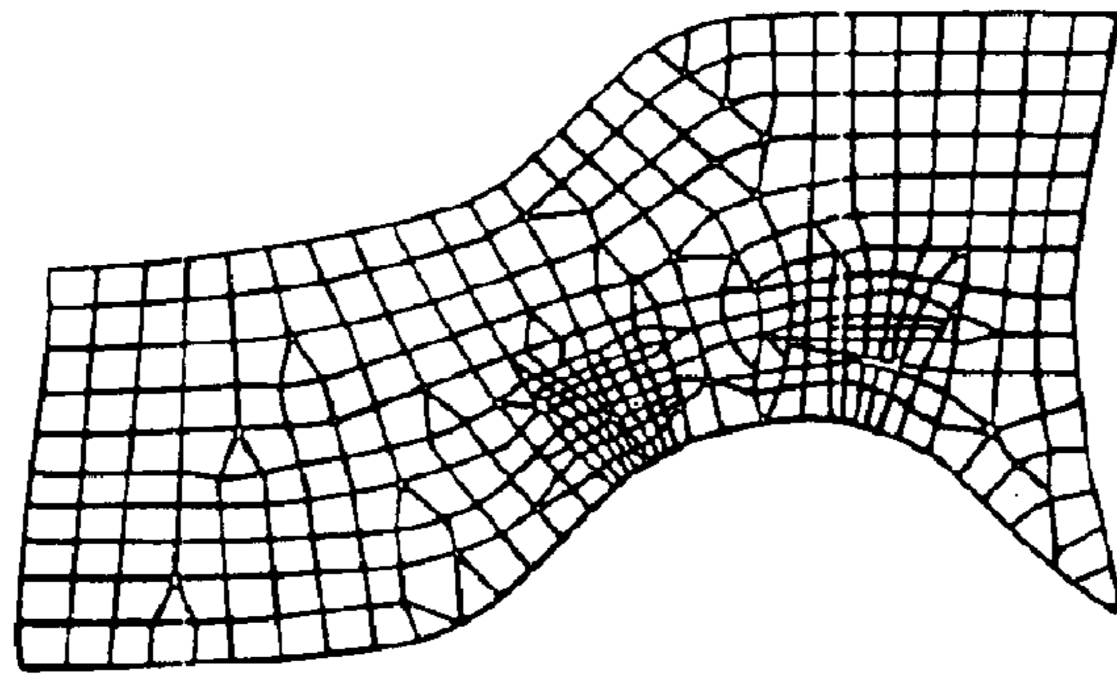
TEMPLATE MESH FIG. 12b
