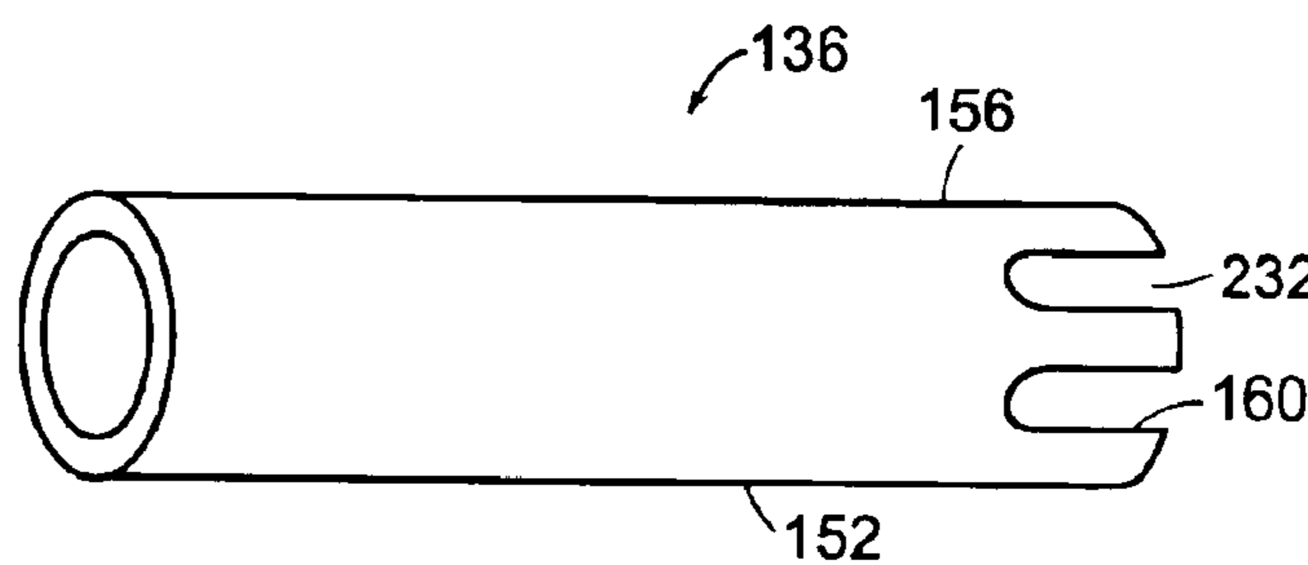
FIG. 5A
