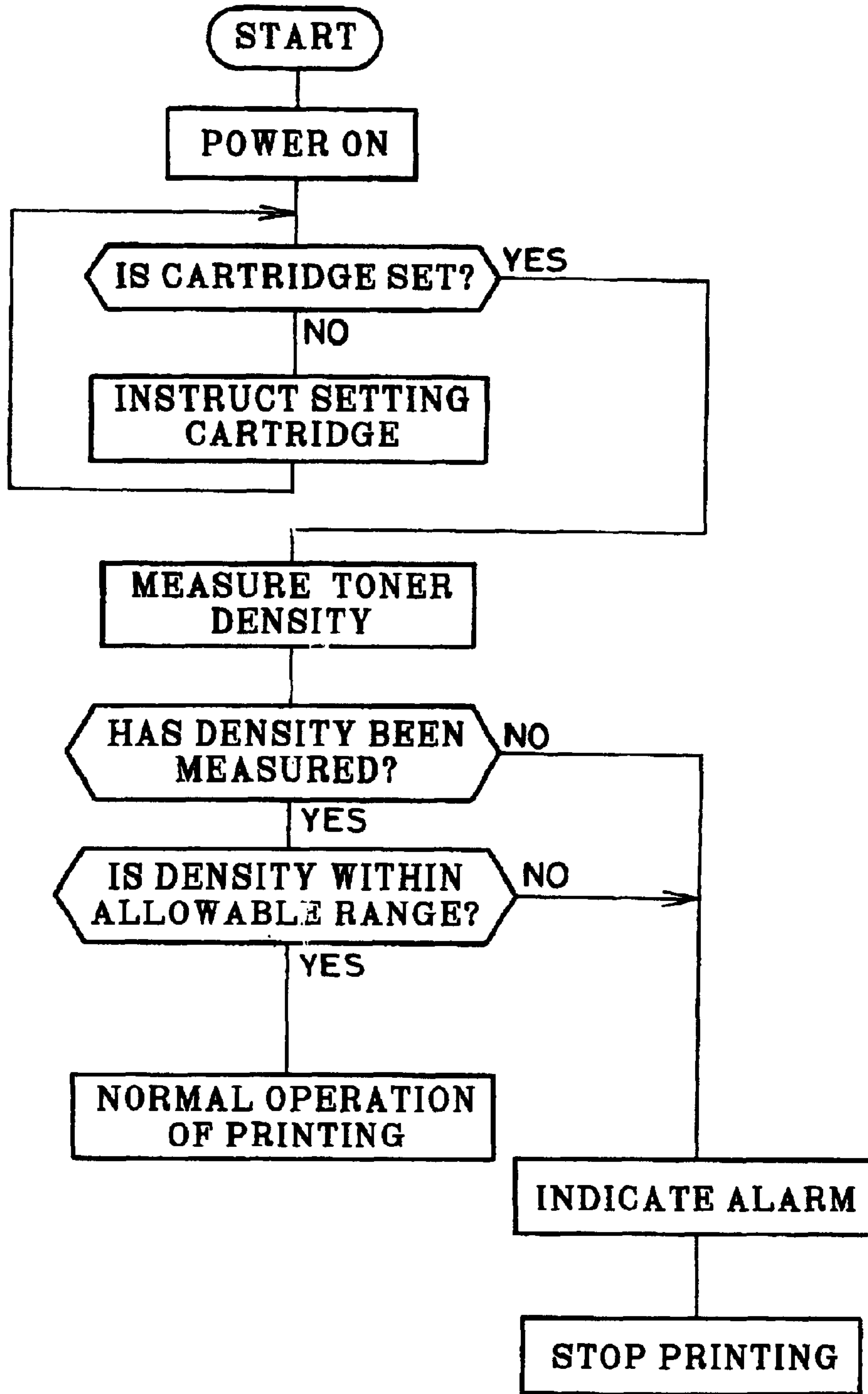
FIG. 20
