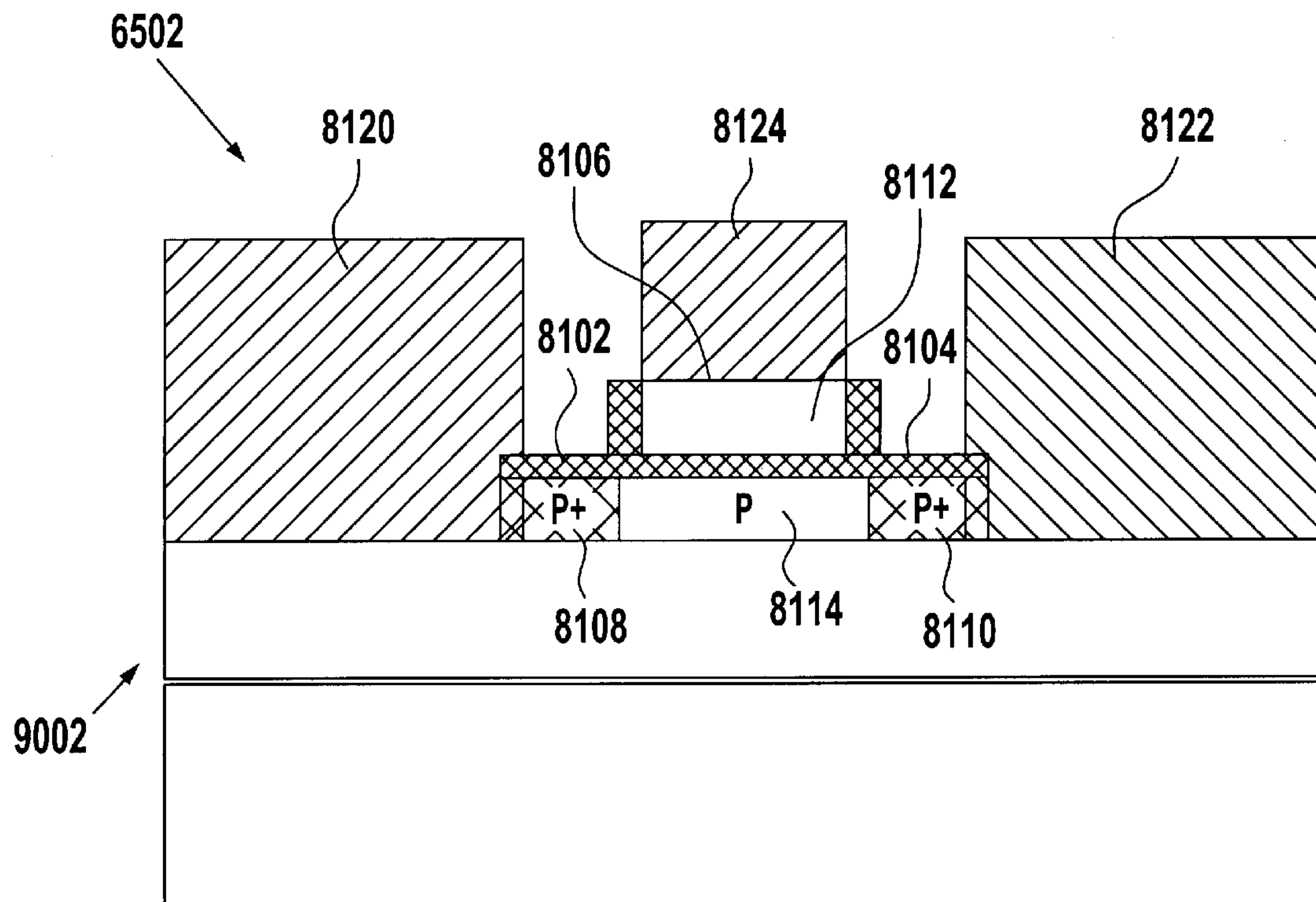
FIG. 91
