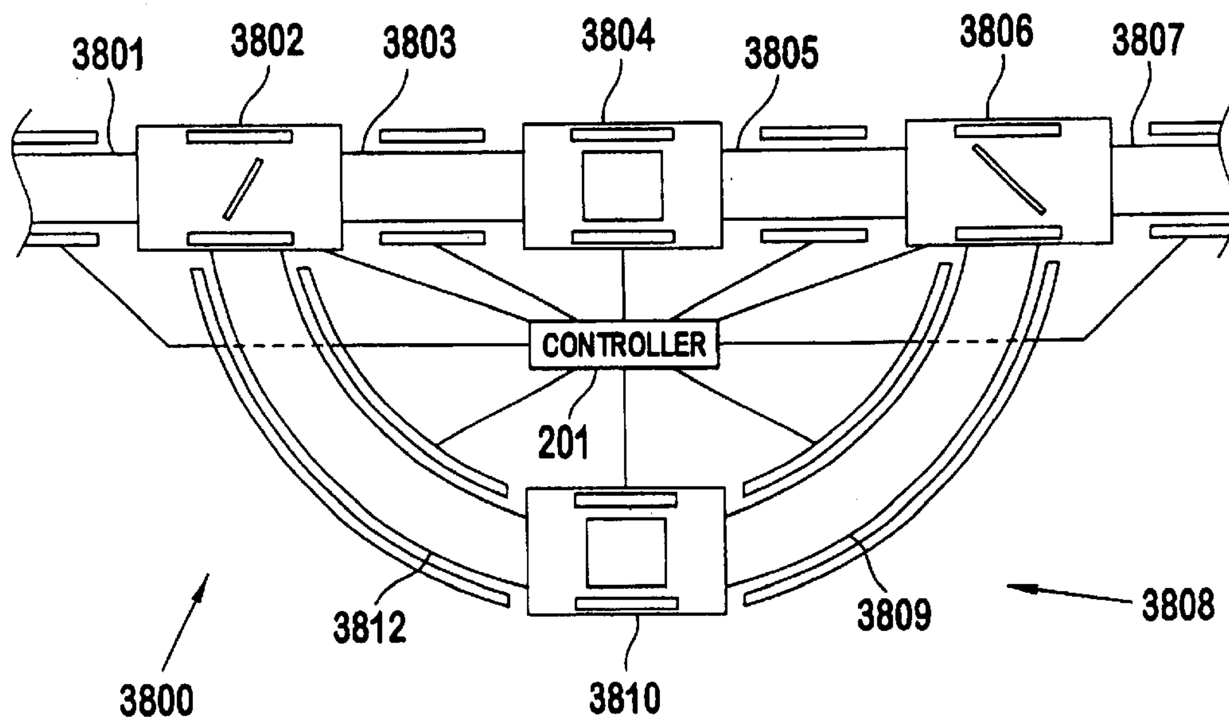
FIG. 38
