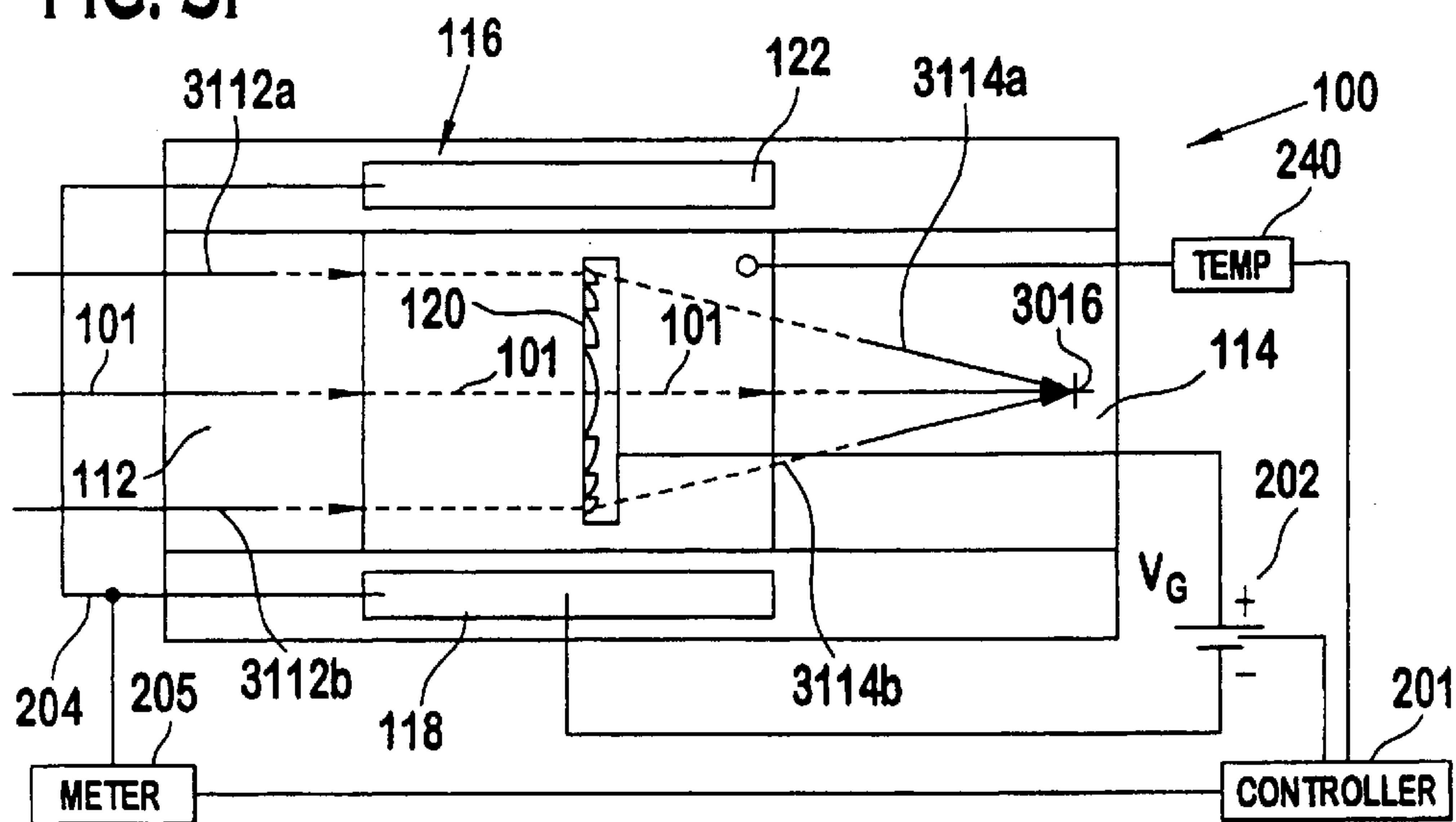
FIG. 31
