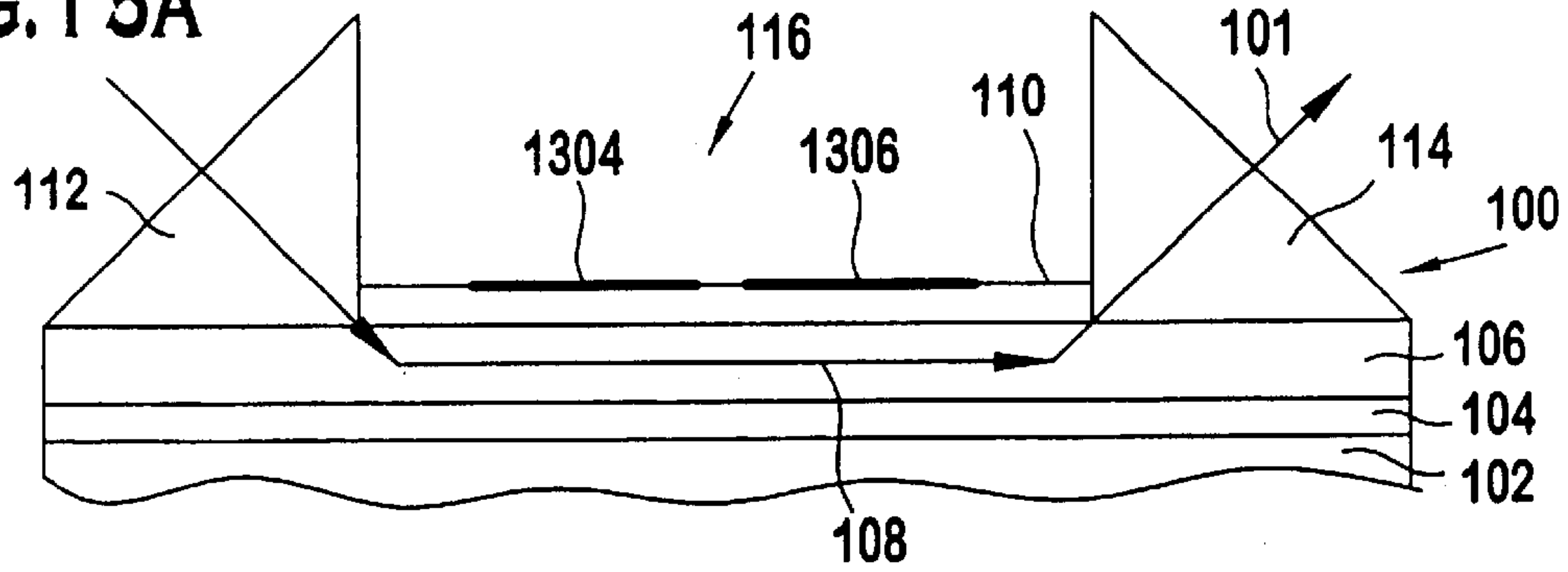
FIG. 15B
