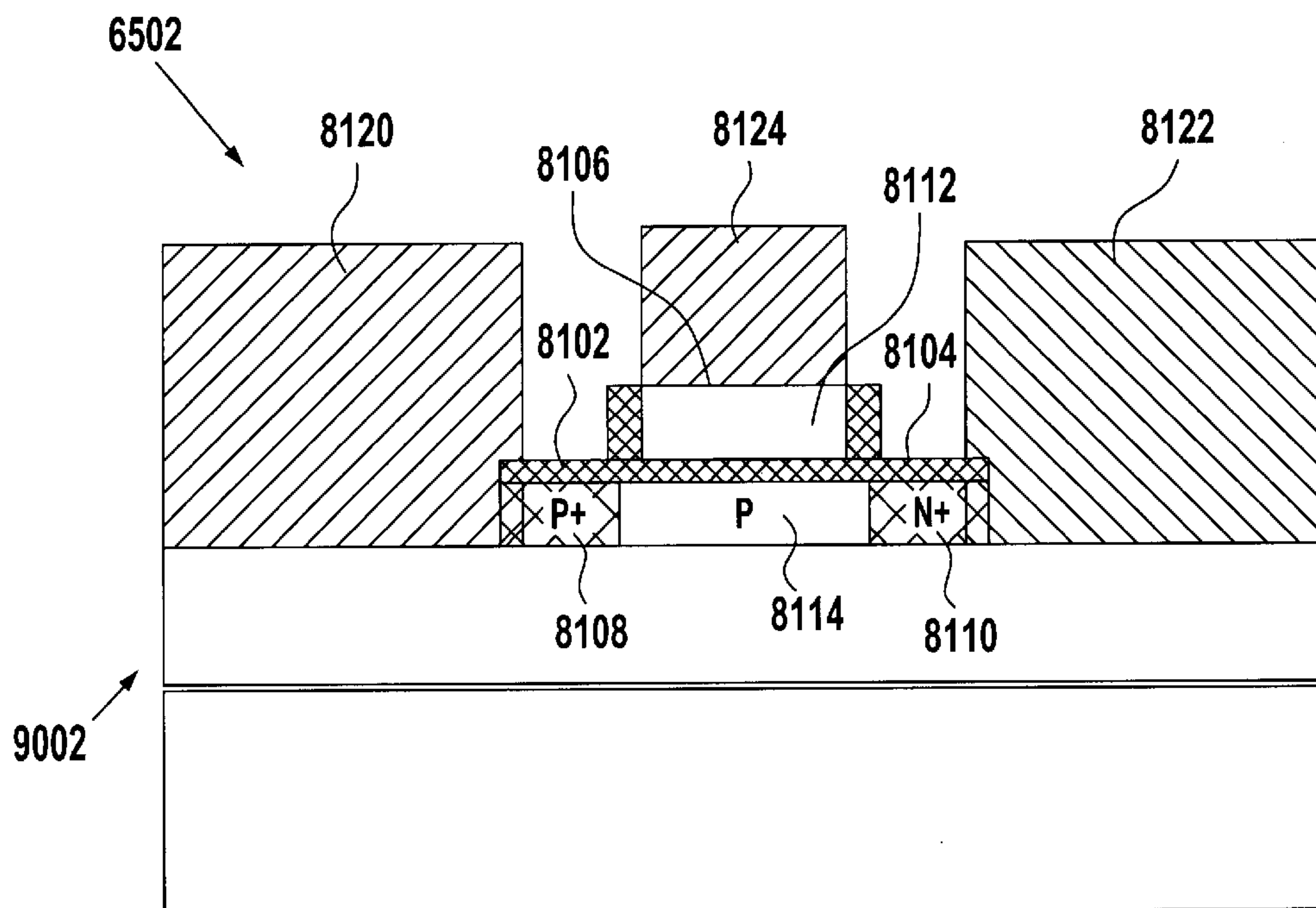
FIG. 90
