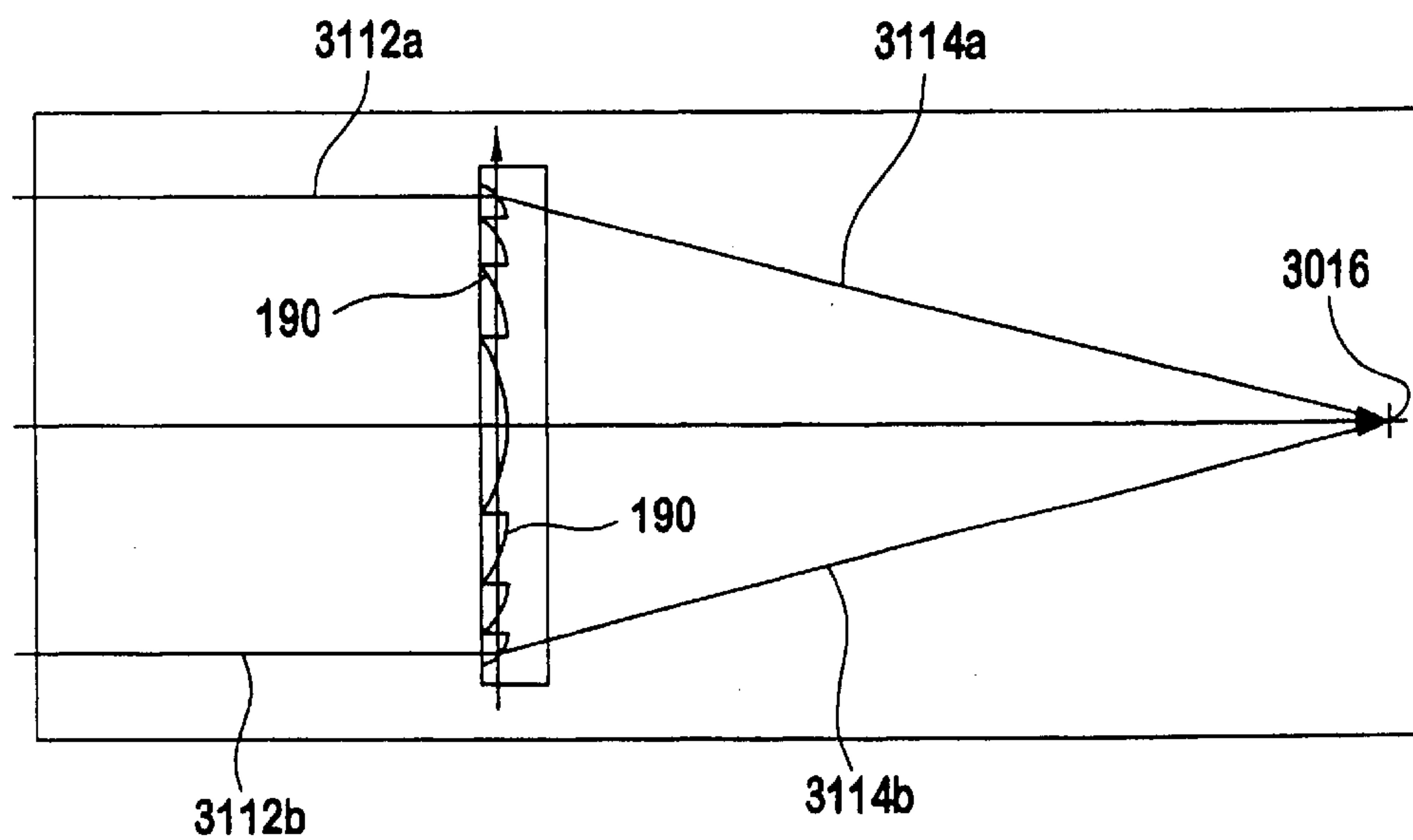
FIG. 31 A
