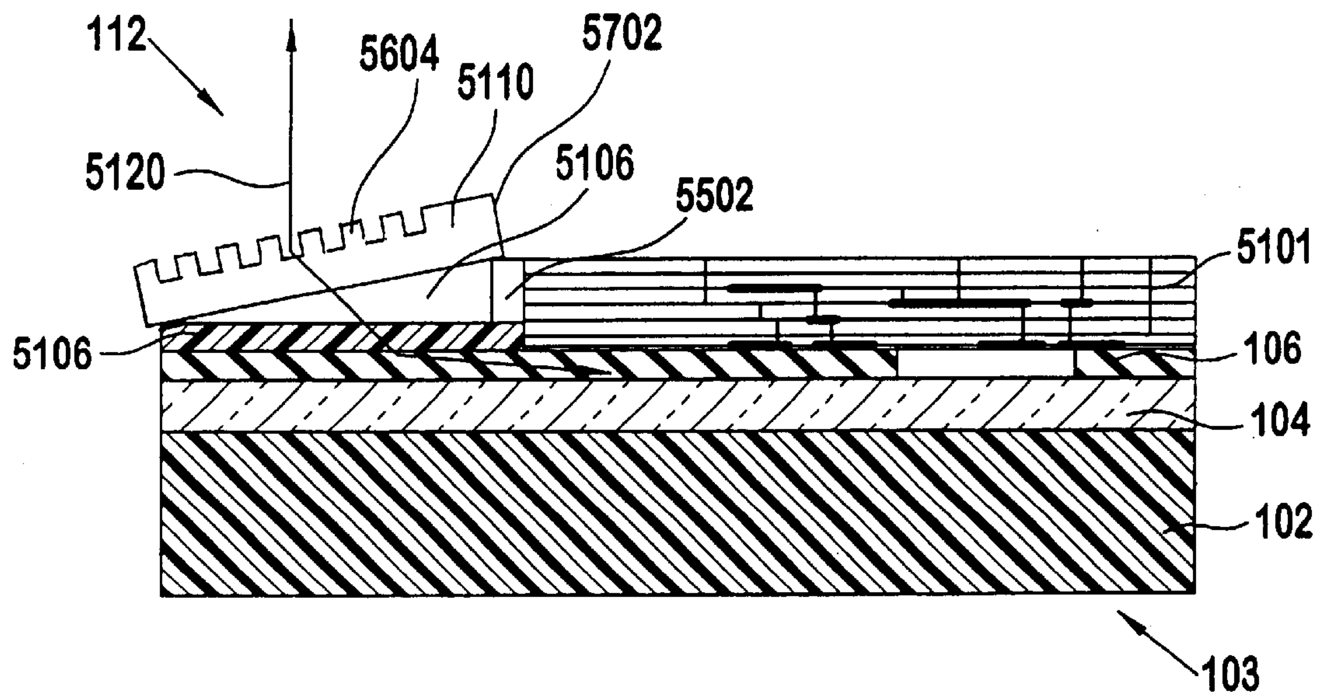
FIG. 57
