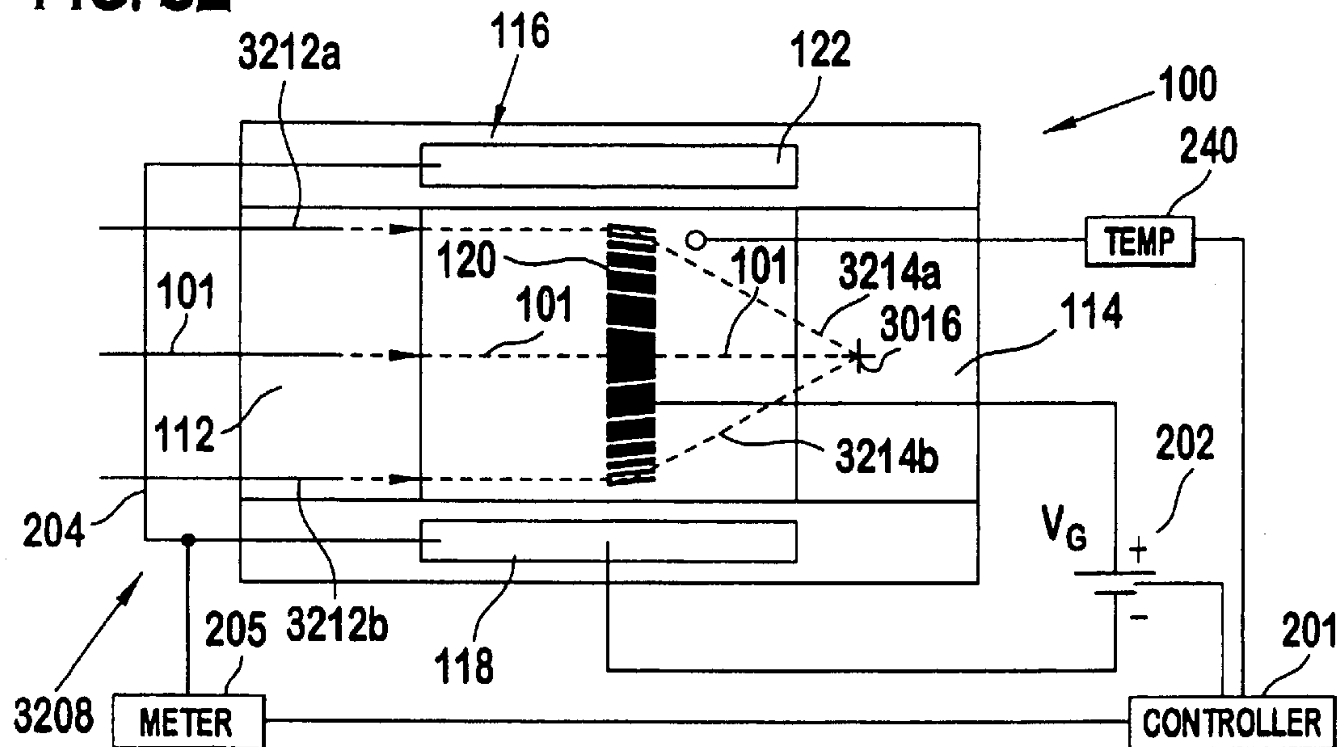
FIG. 32
