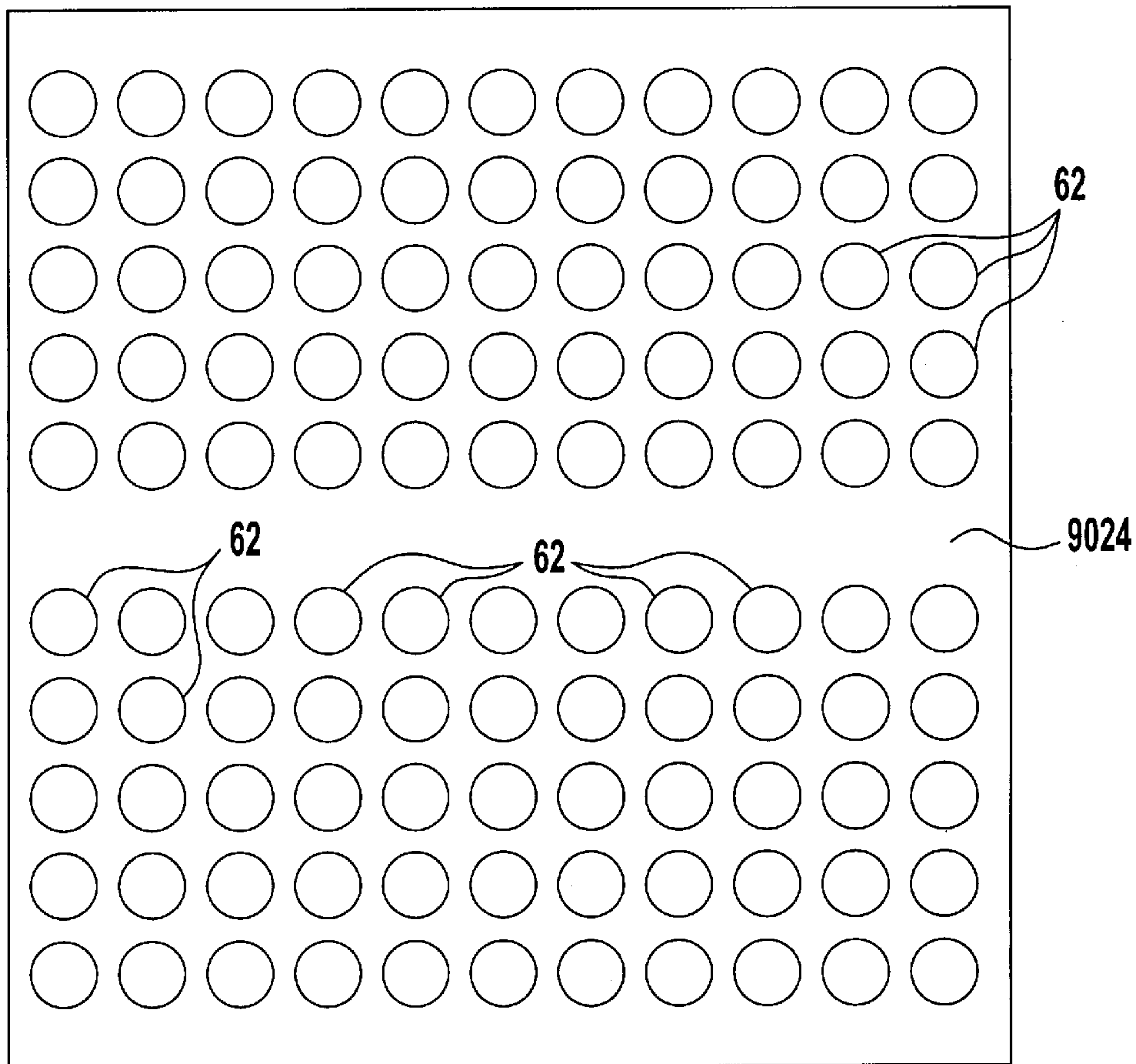
FIG. 86
