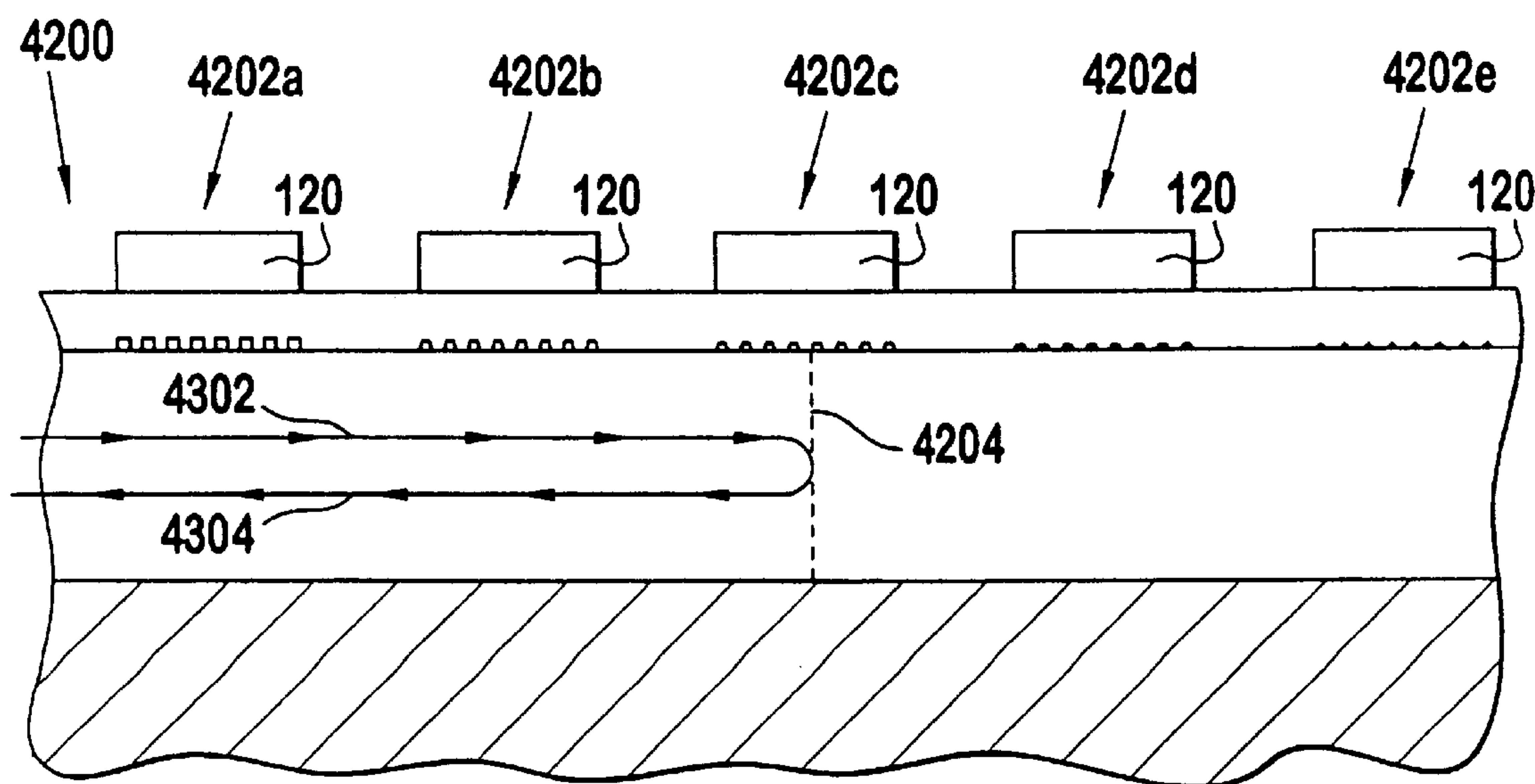
FIG. 43
