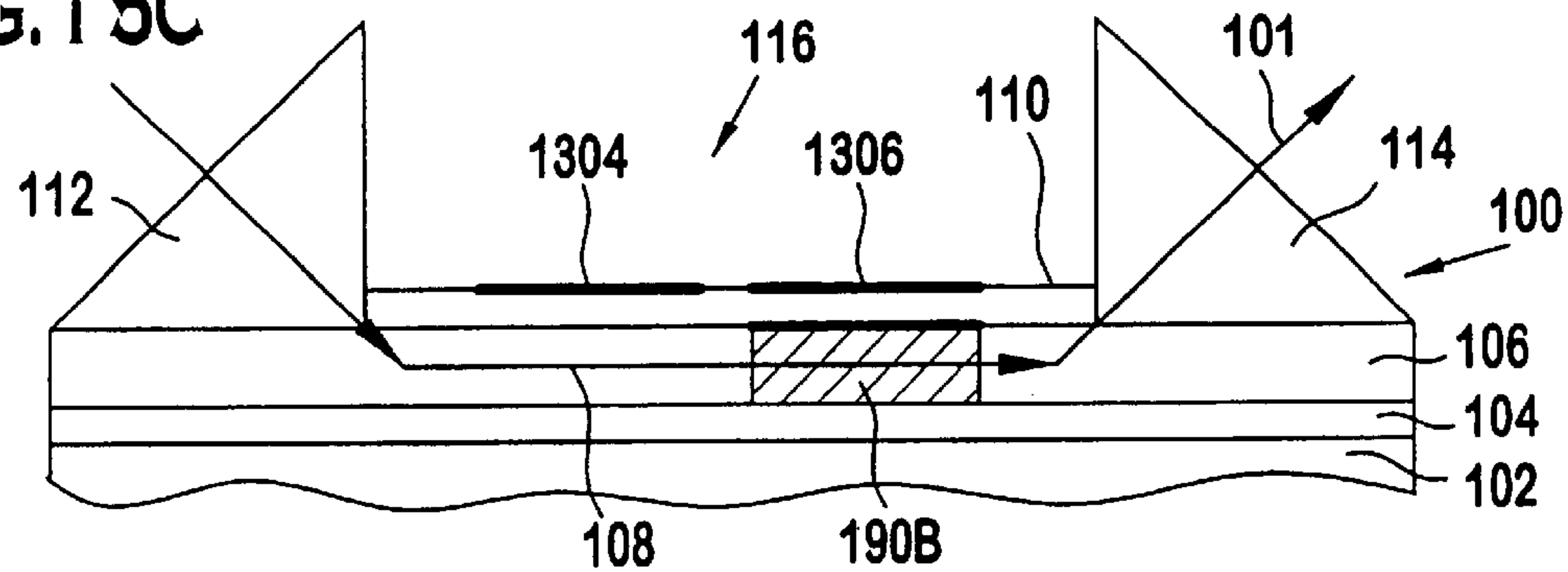
FIG. 15D
