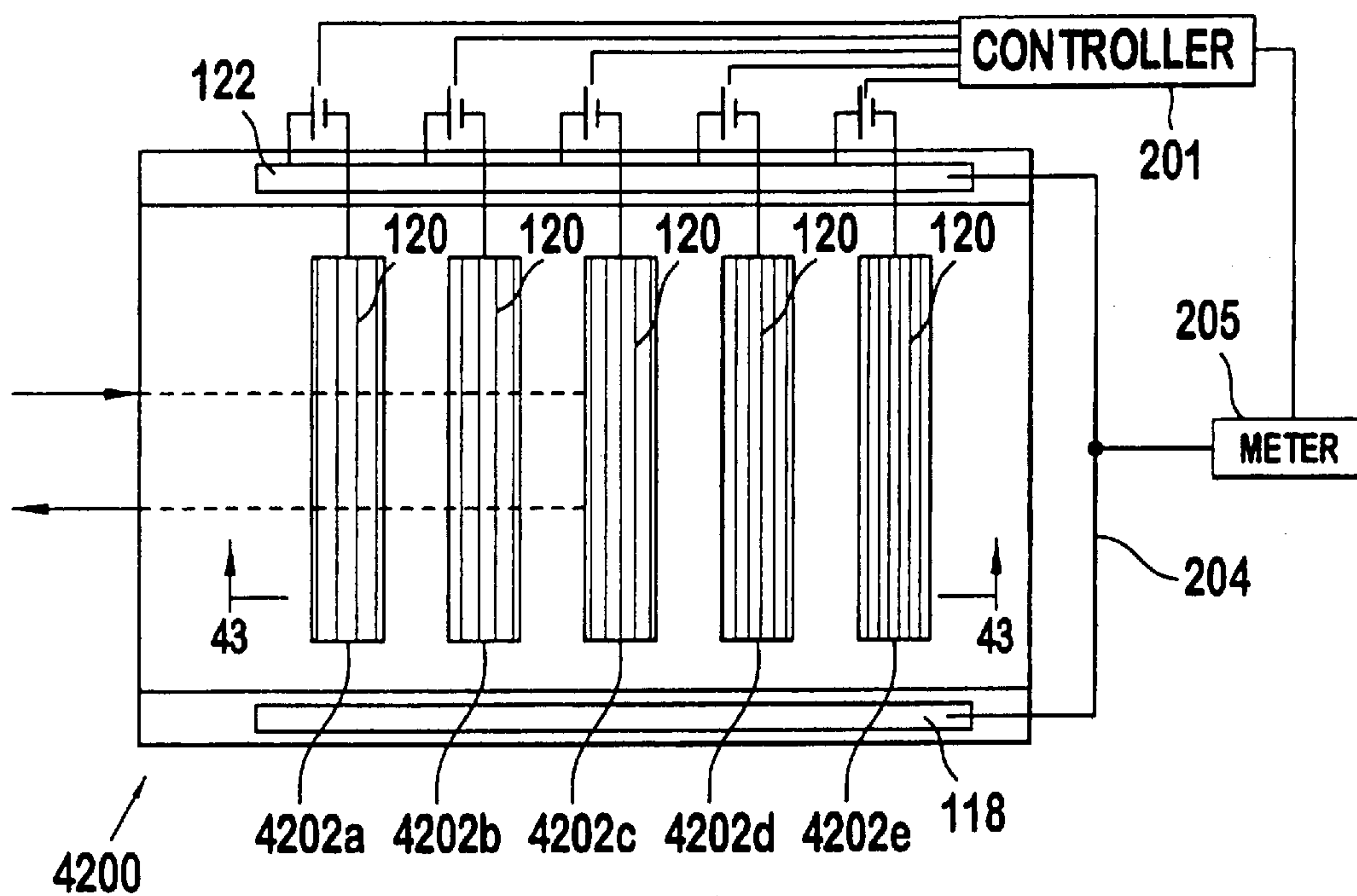
FIG. 42
