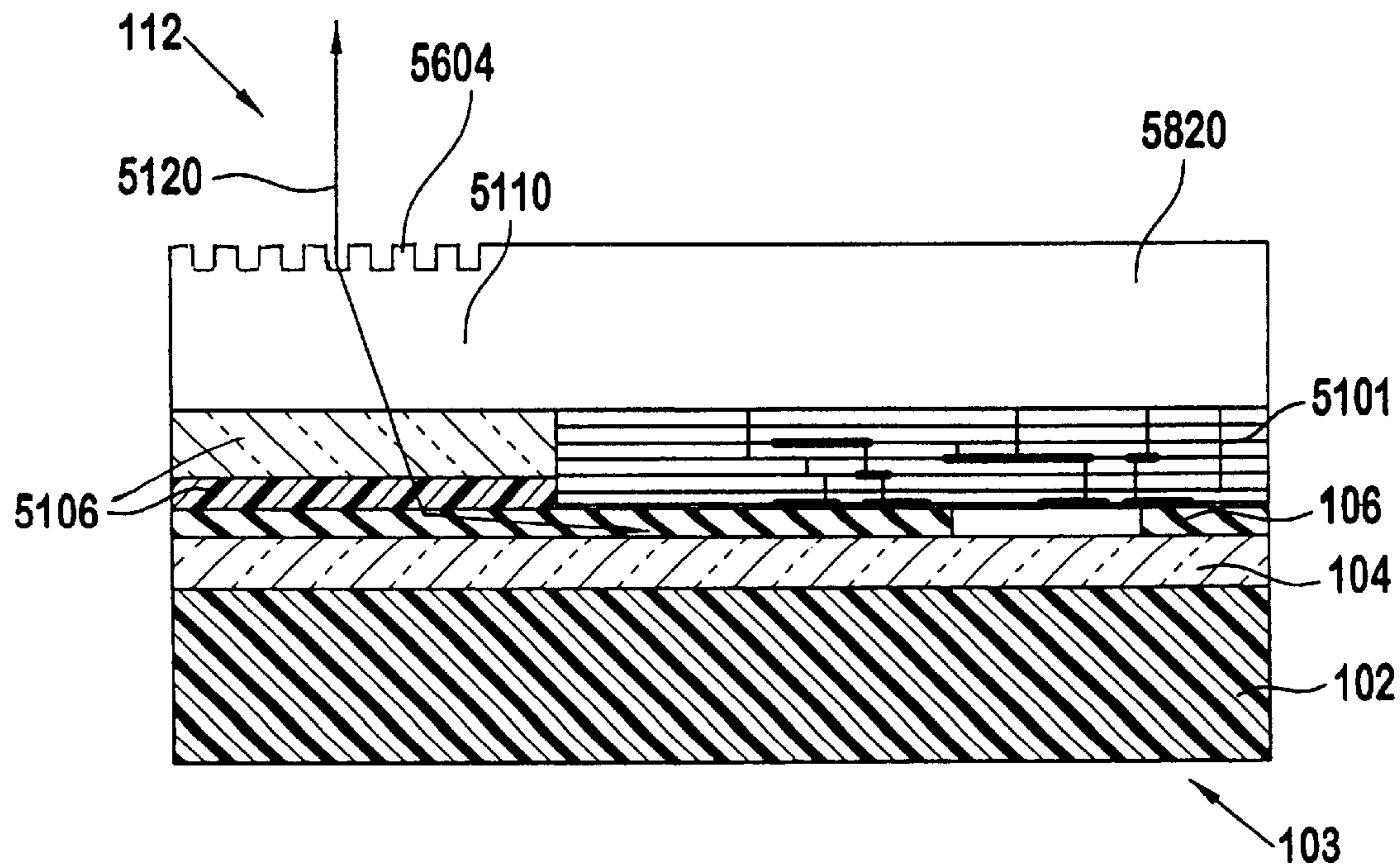
FIG. 58
