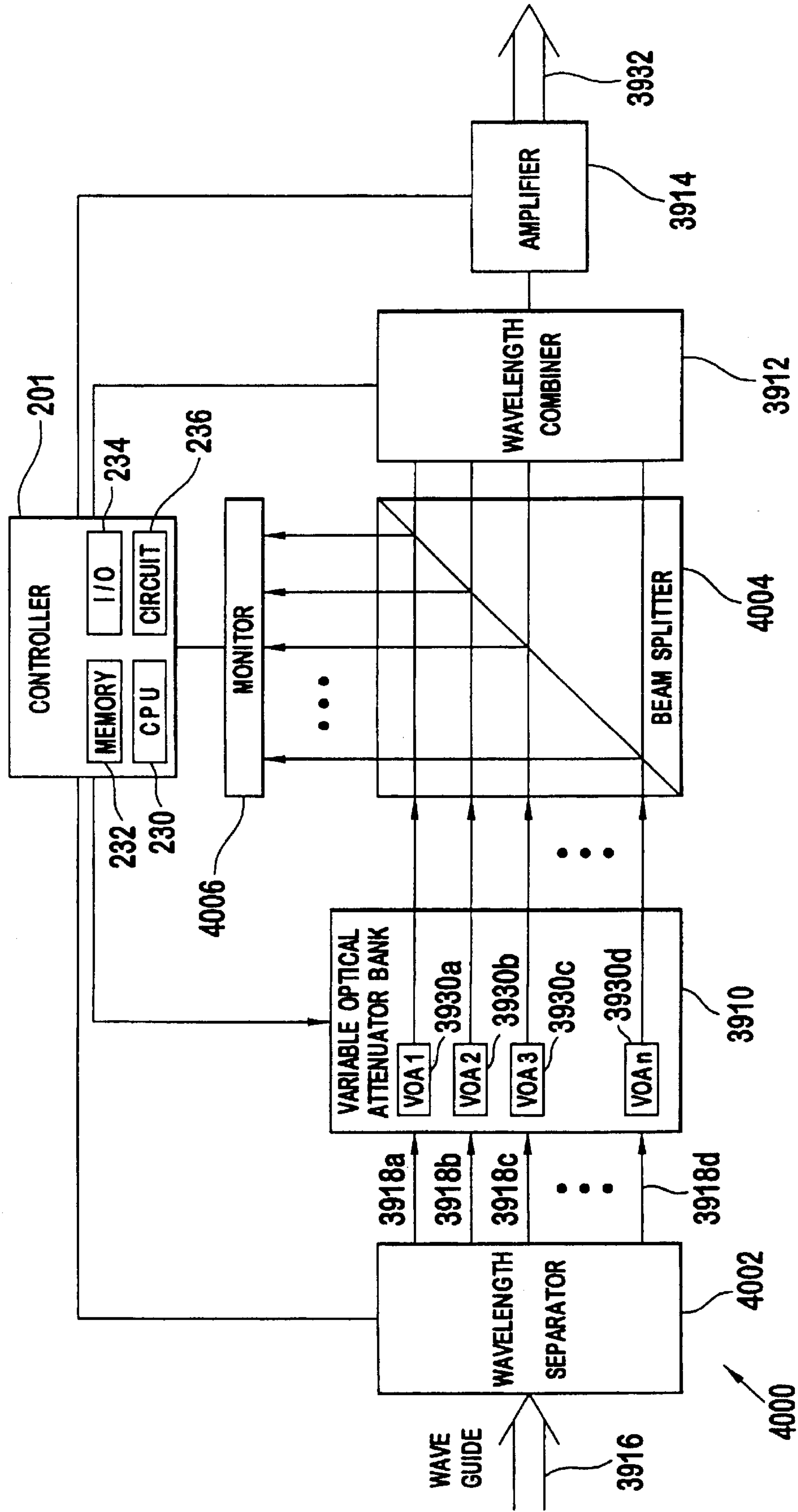
FIG. 40
