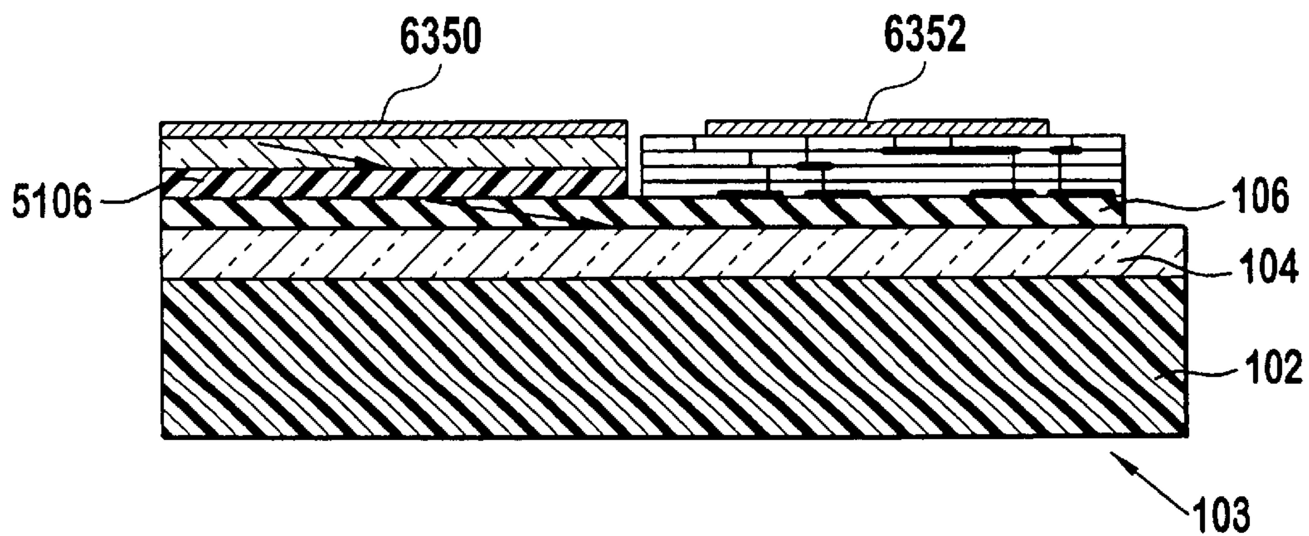
FIG. 63D
