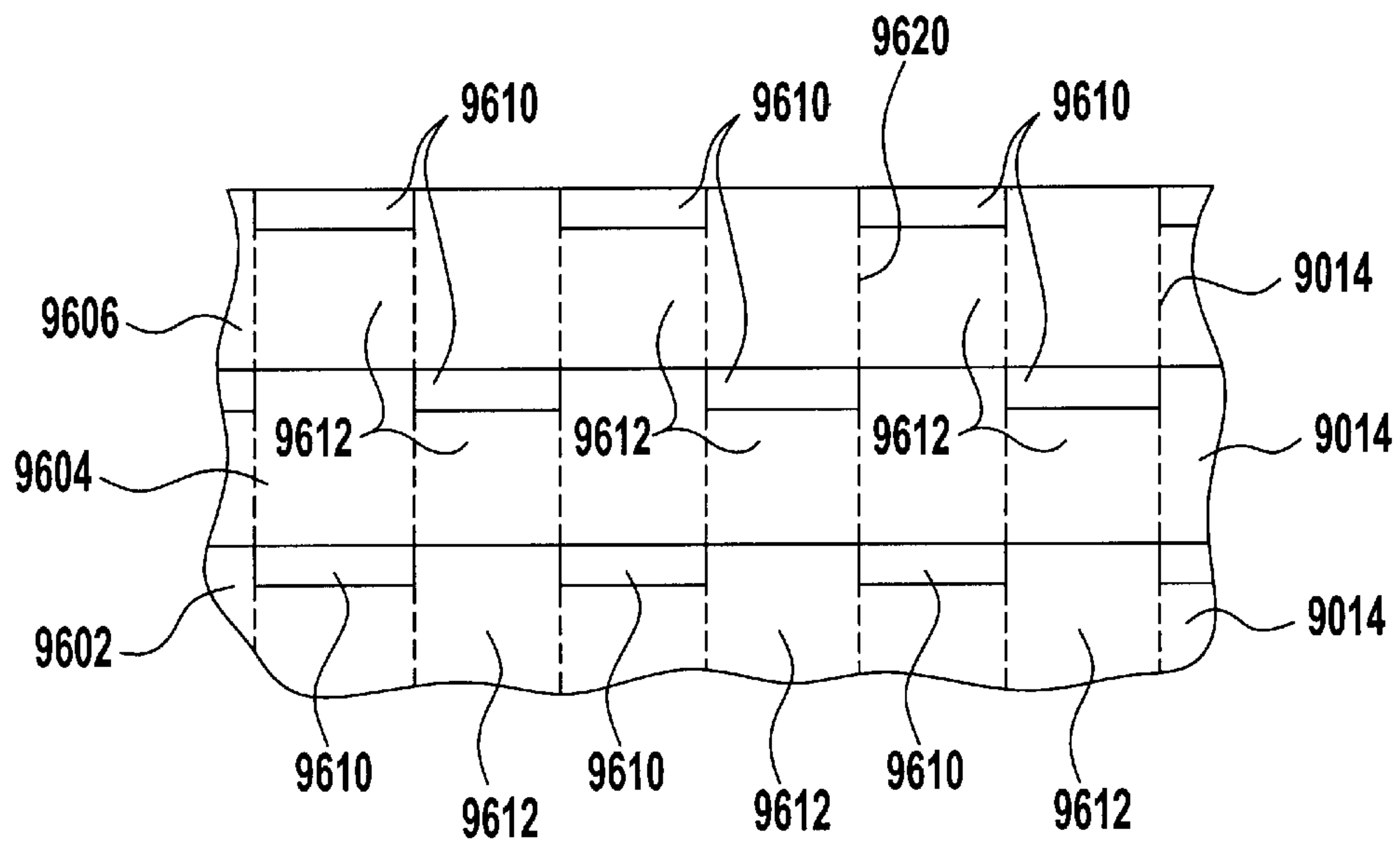
FIG. 87
