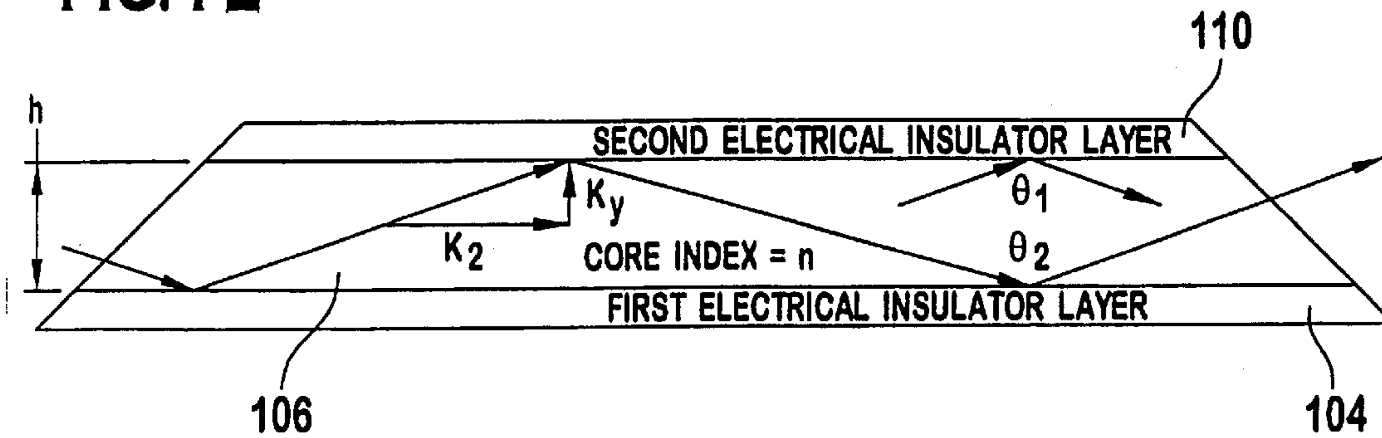
FIG. 12
