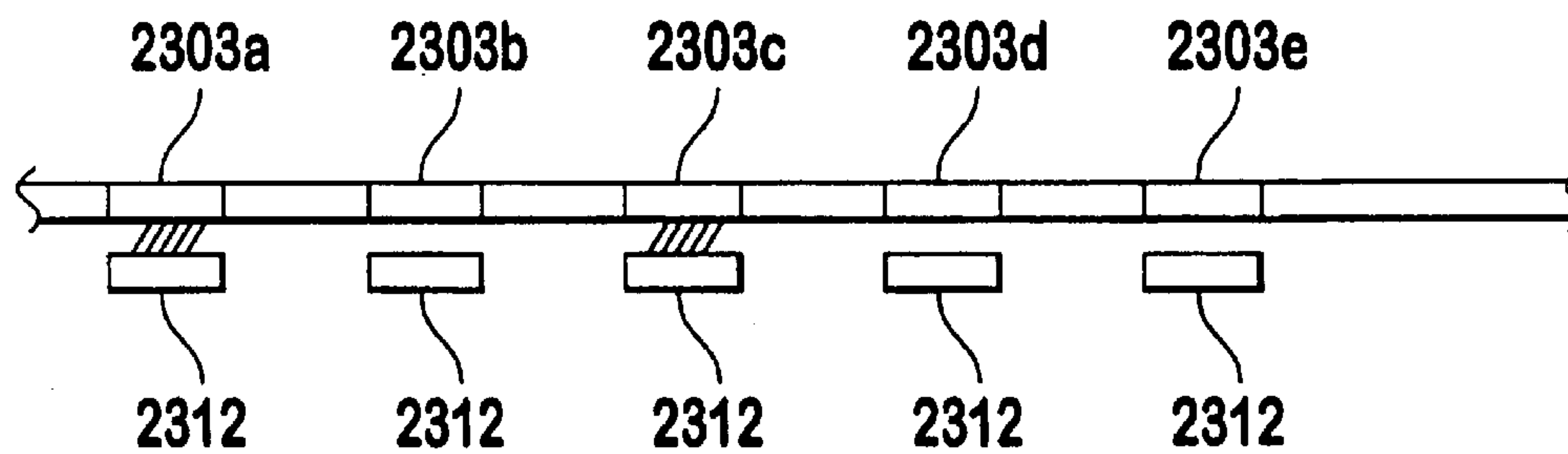
FIG. 24
