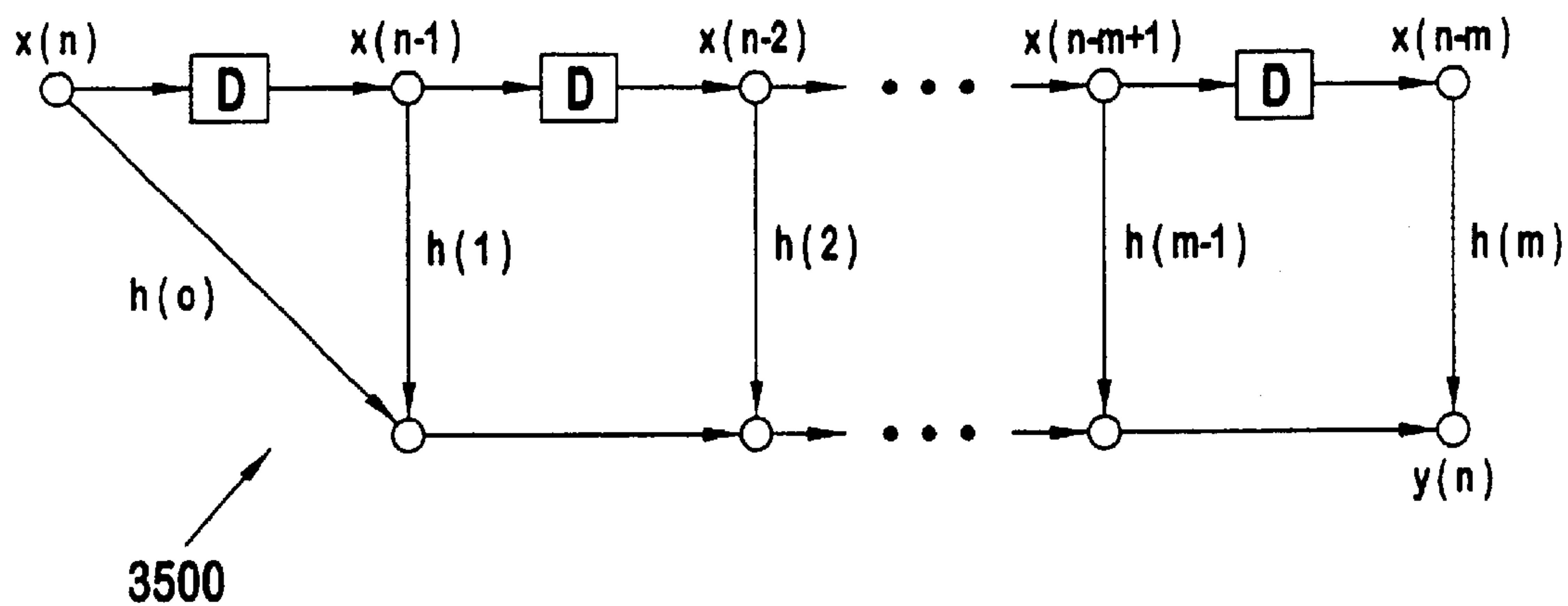
FIG. 35
