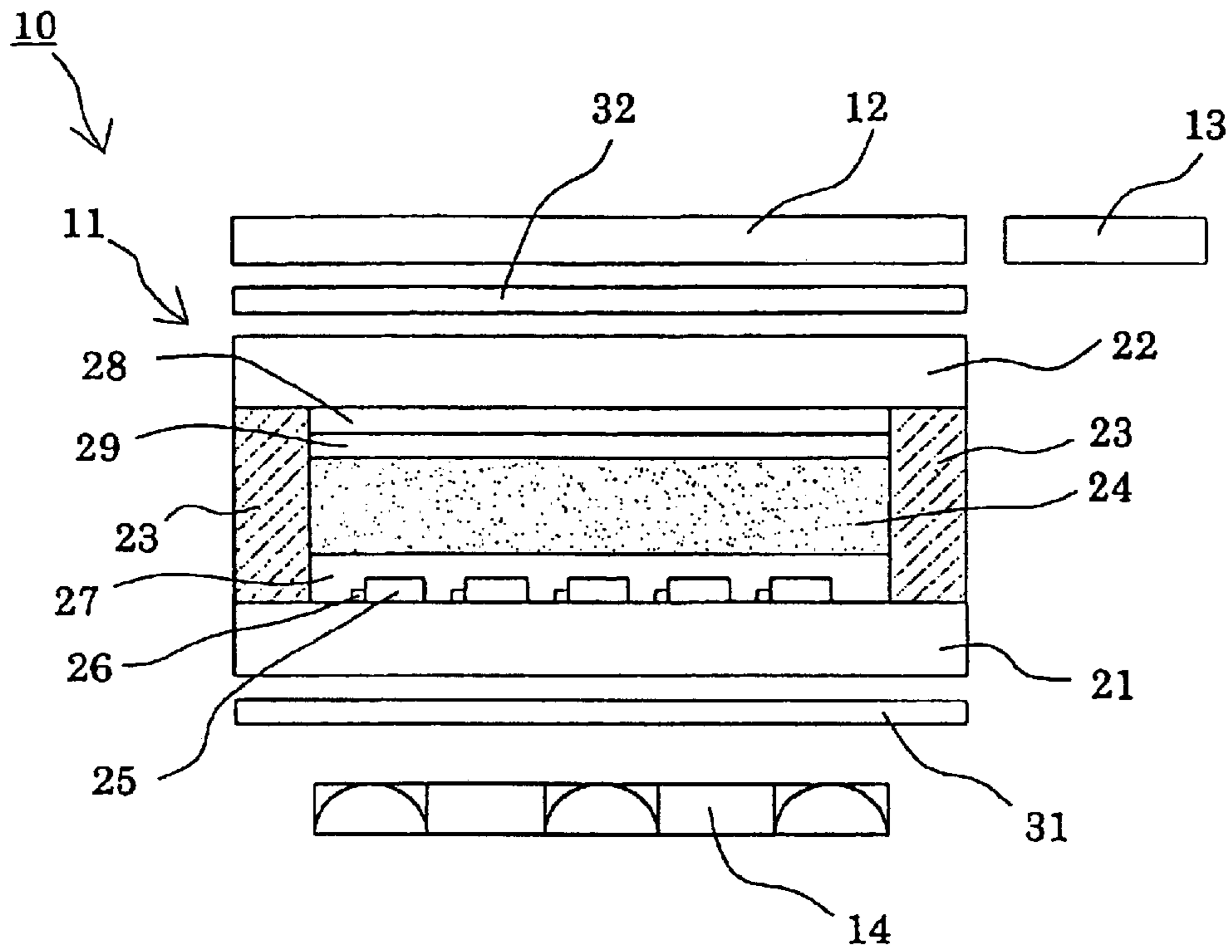
FIG. 1B
