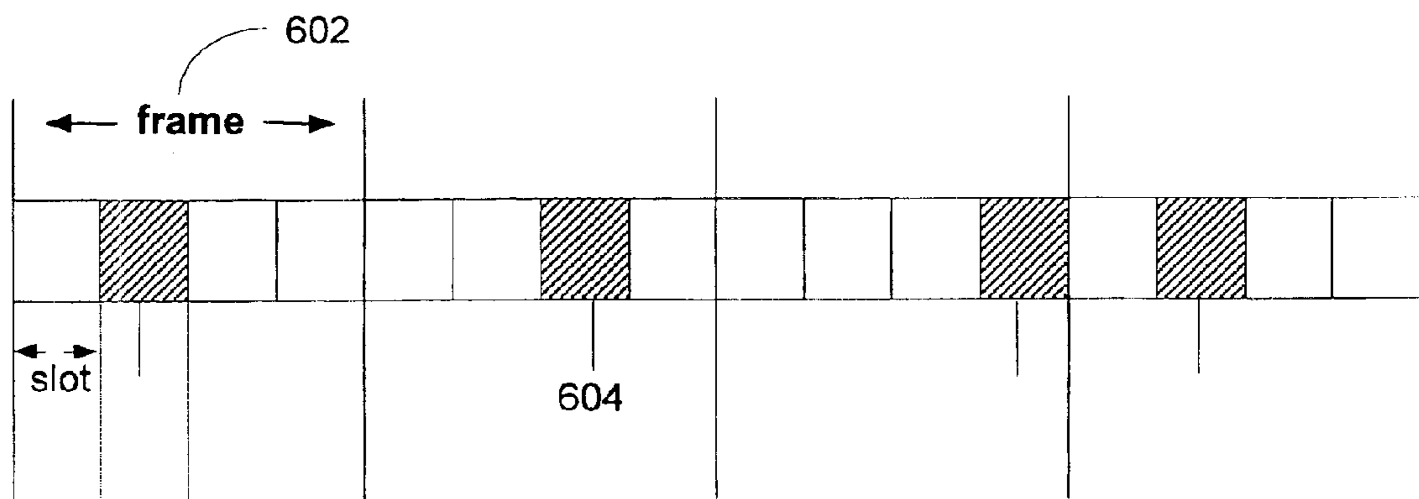
FIG. 6A
