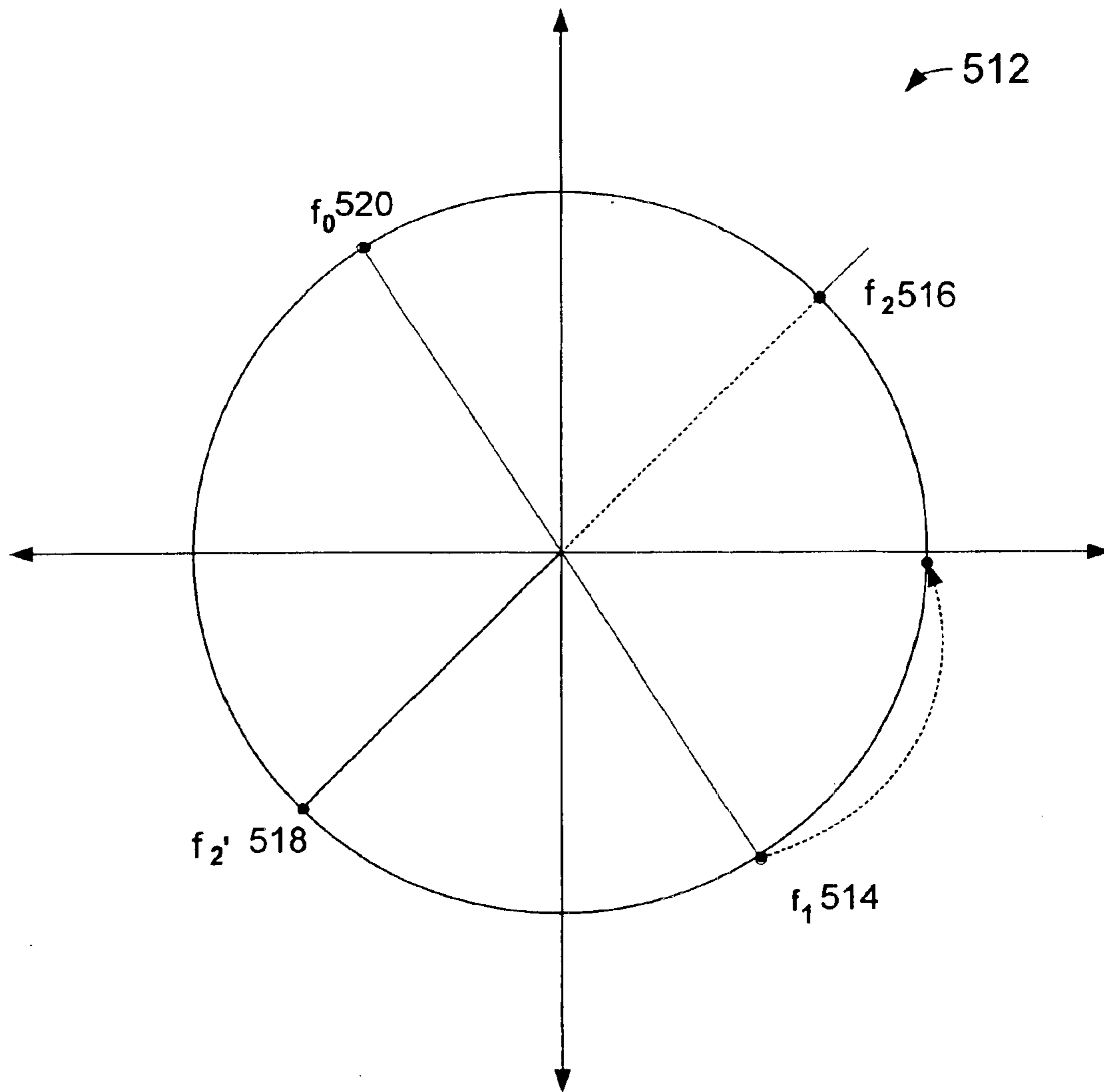
FIG. 5B
