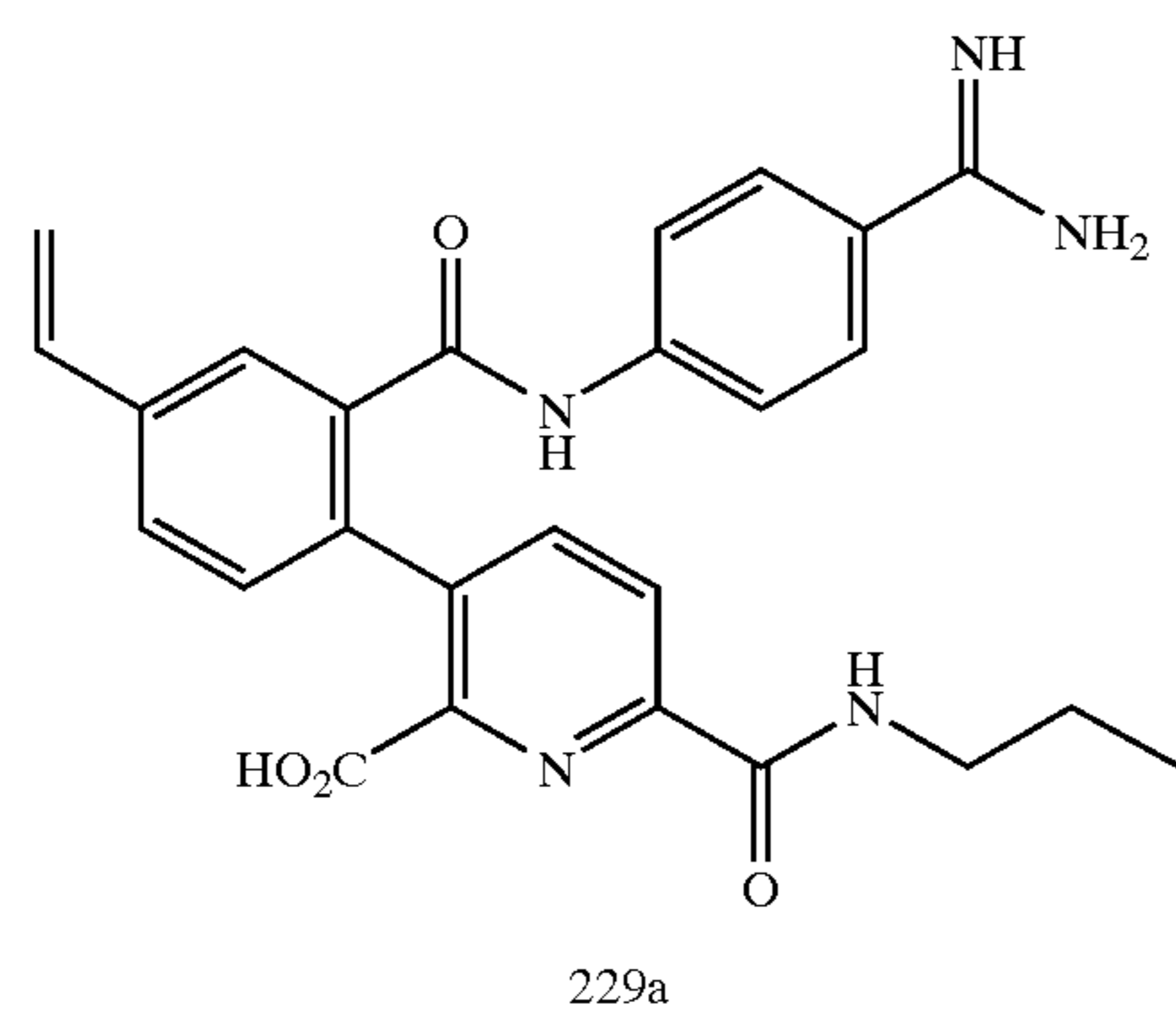
Scheme 31a
