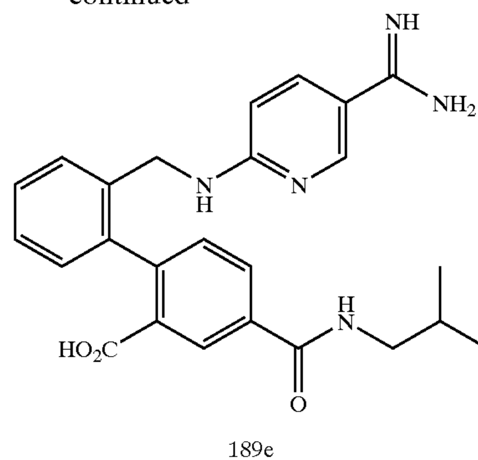
Scheme 25a
