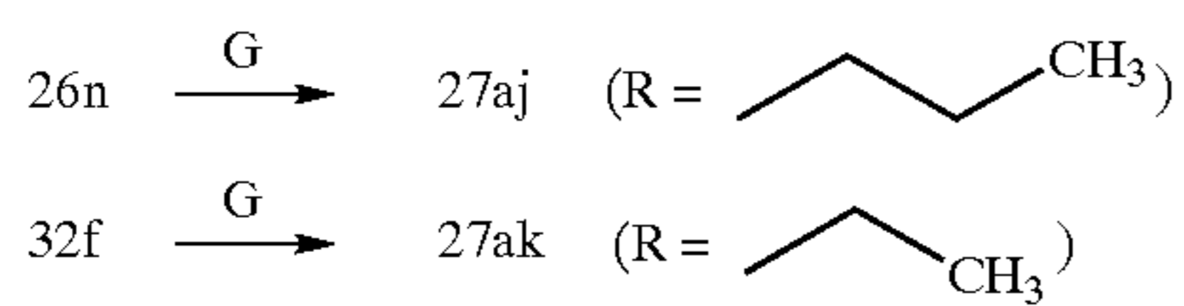
Scheme 8E
