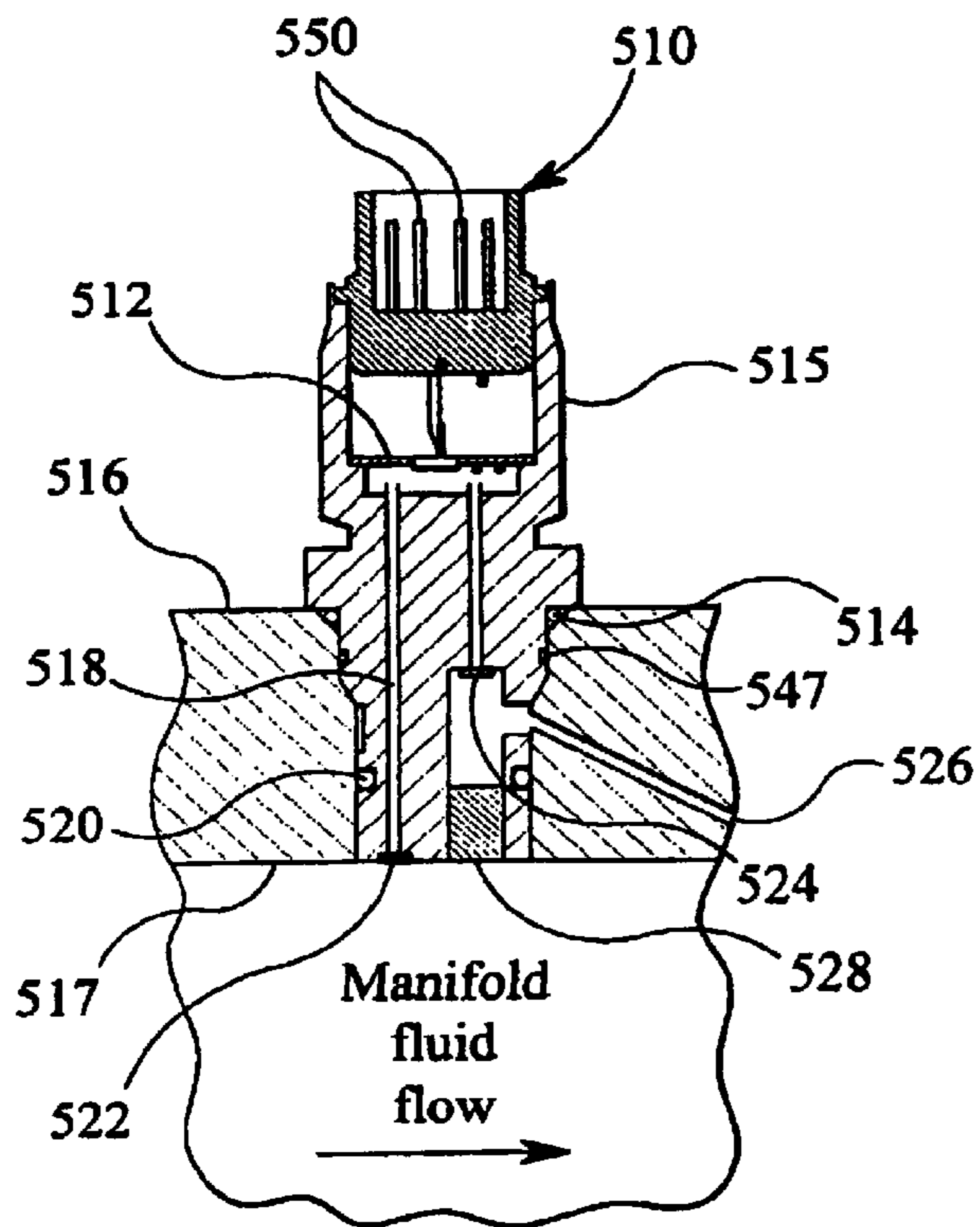
FIG 4 section A-A
