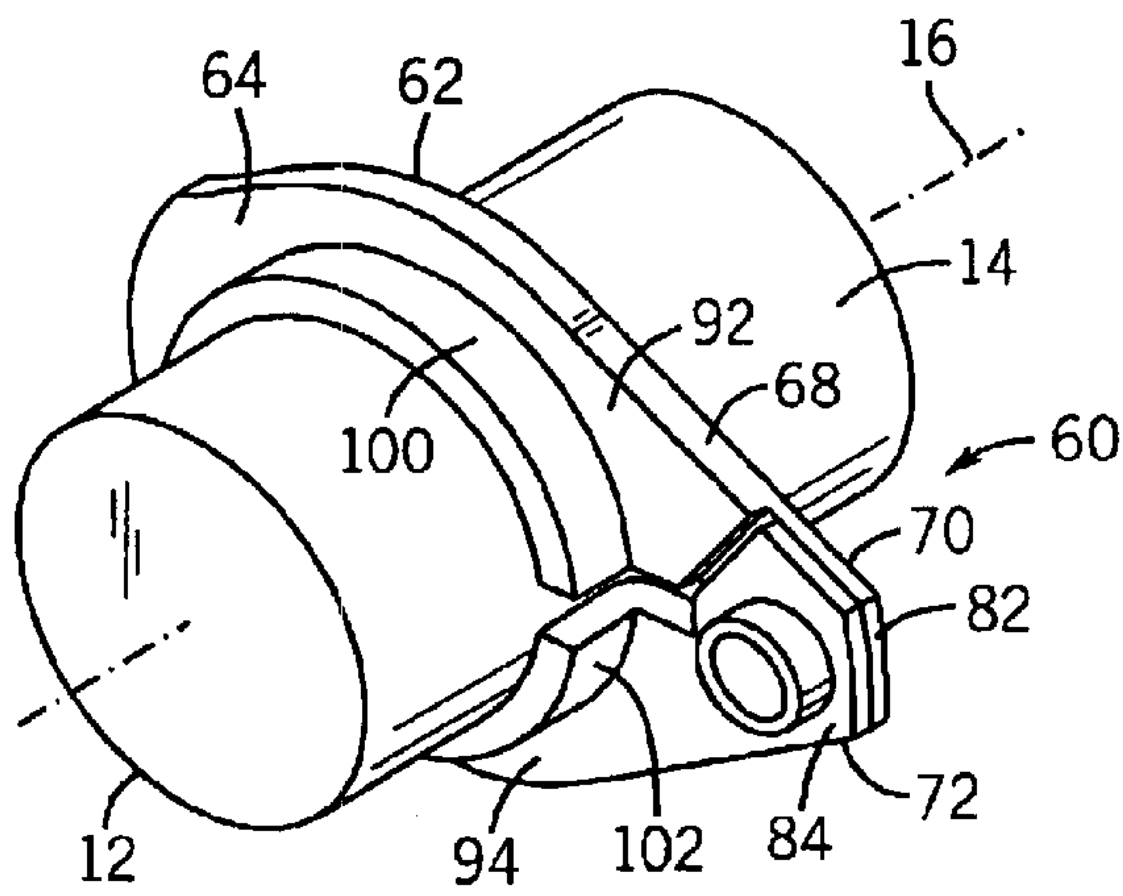
FIG. 11
