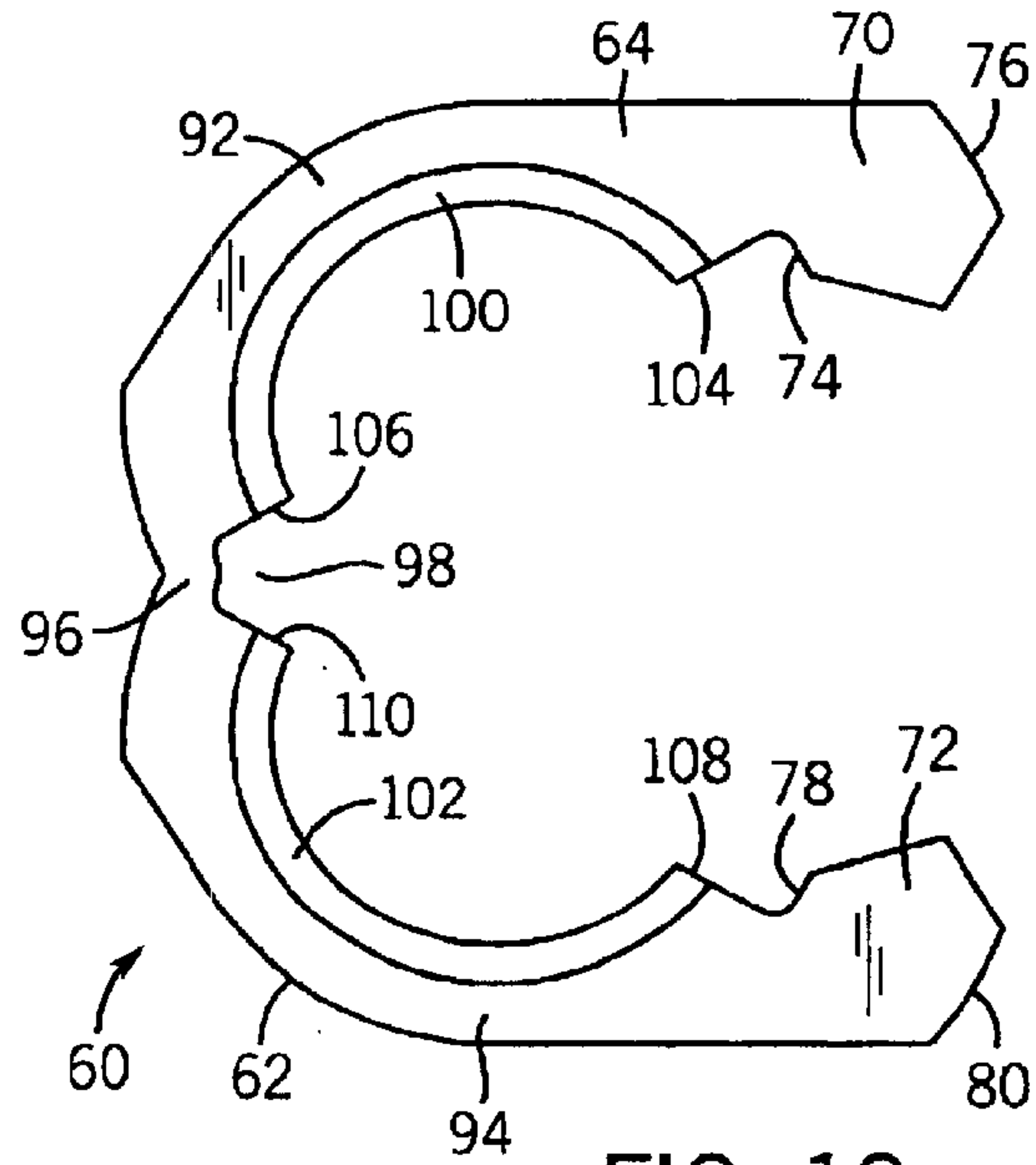
FIG. 12
