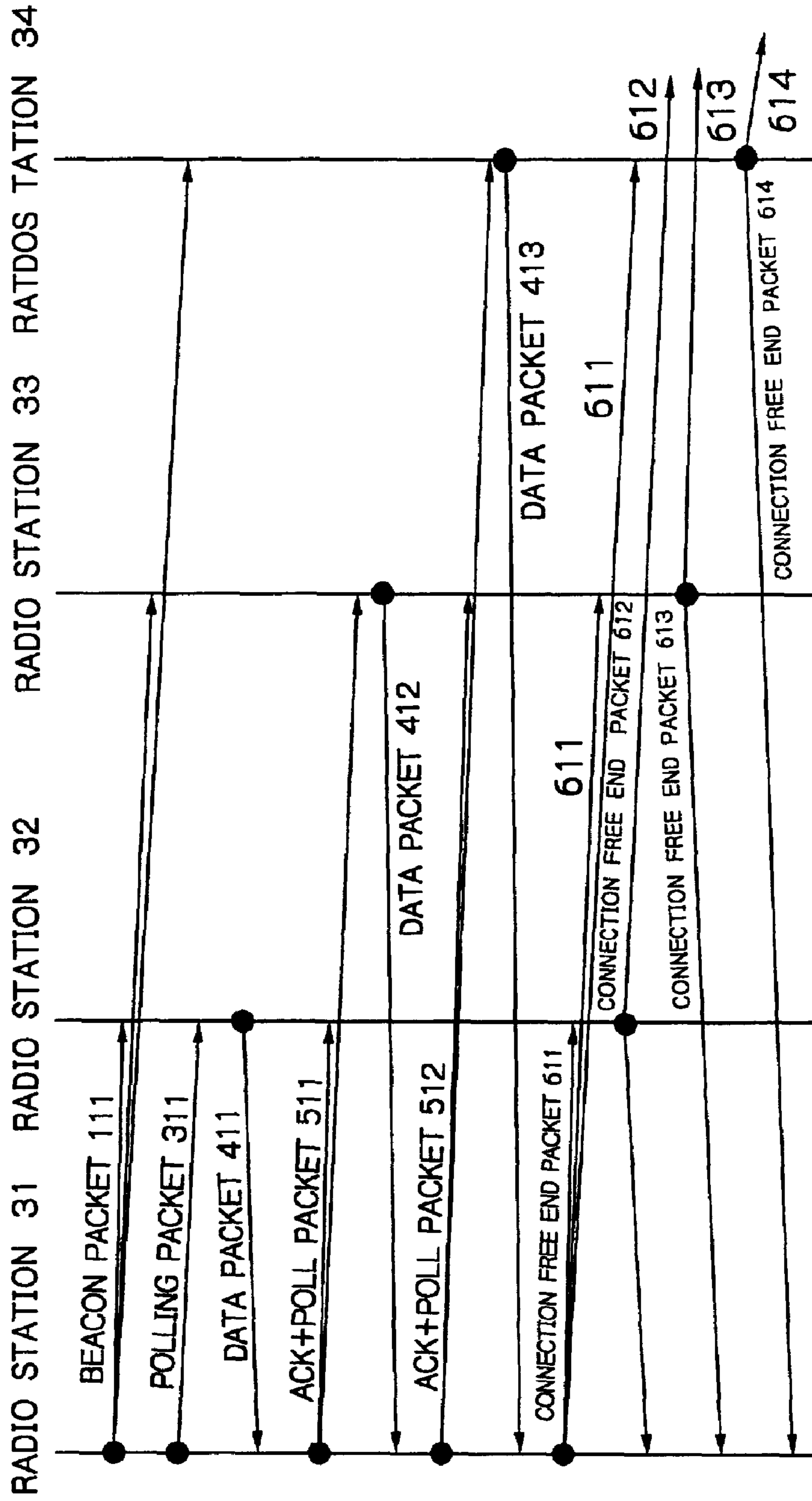
Fig. 3A
