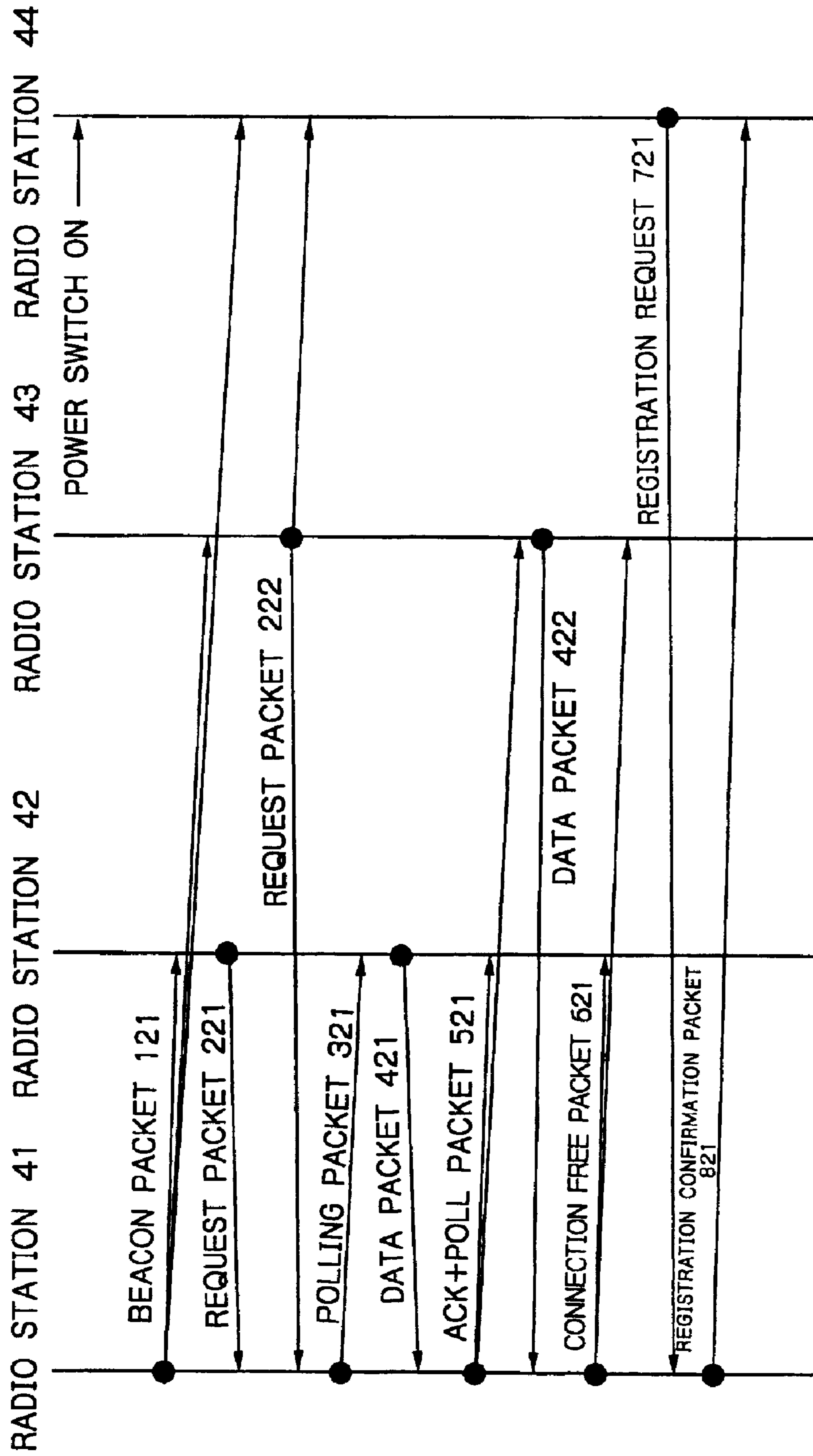
Fig. 4A
