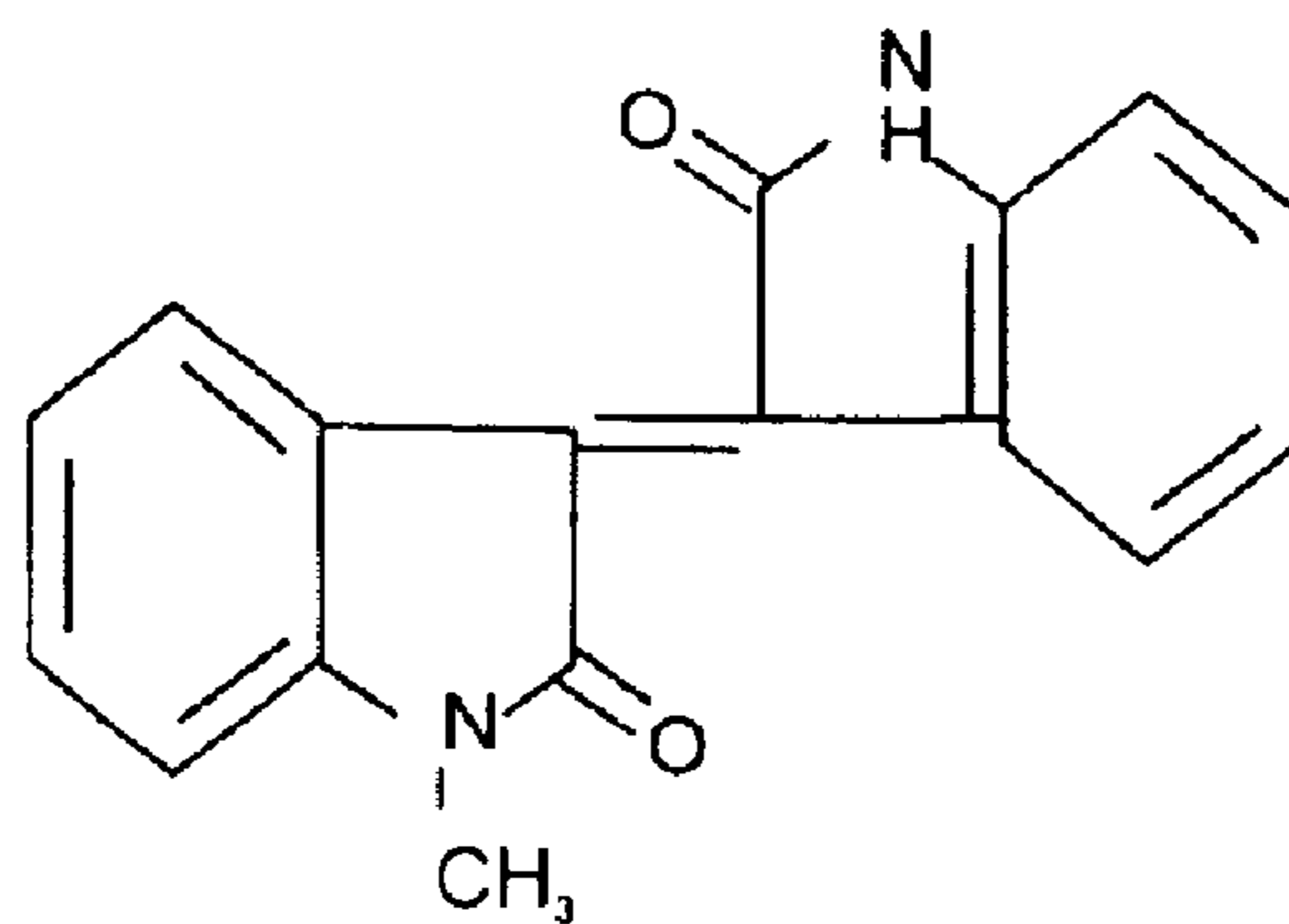
Meisoindigo
