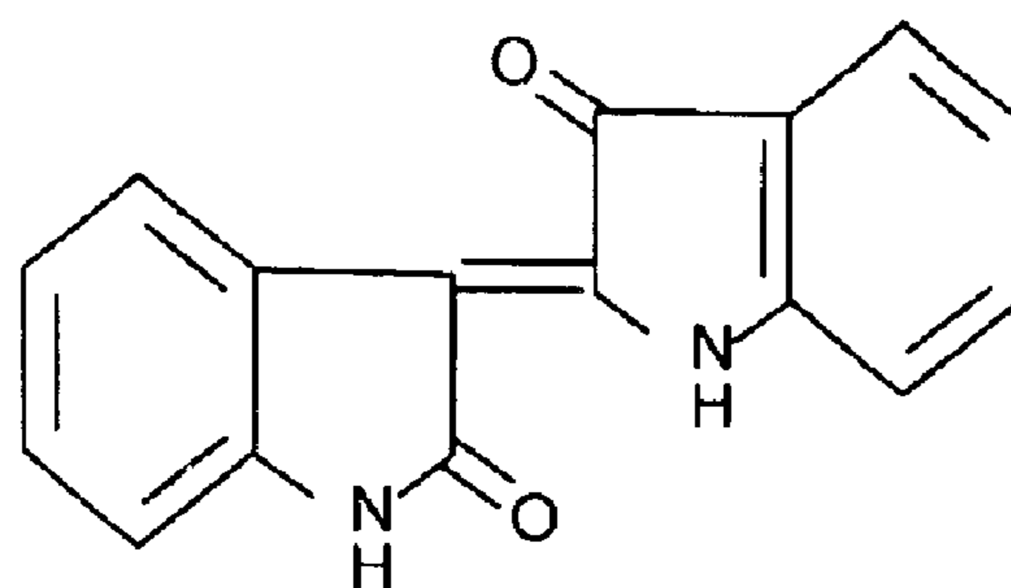
Indirubin
