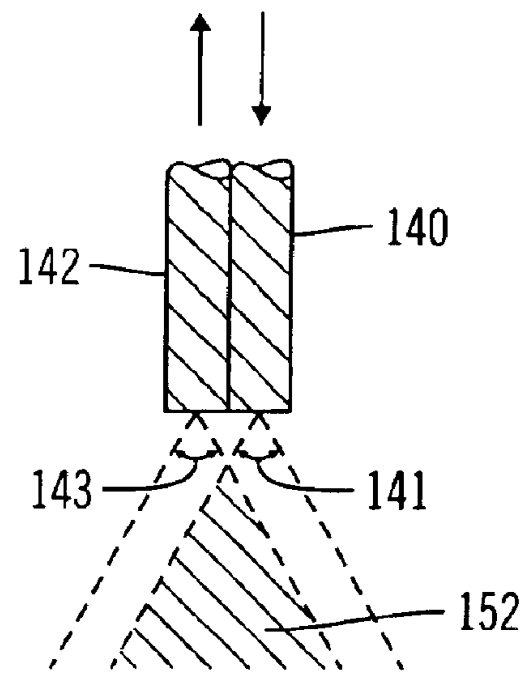
FIG. 10C
