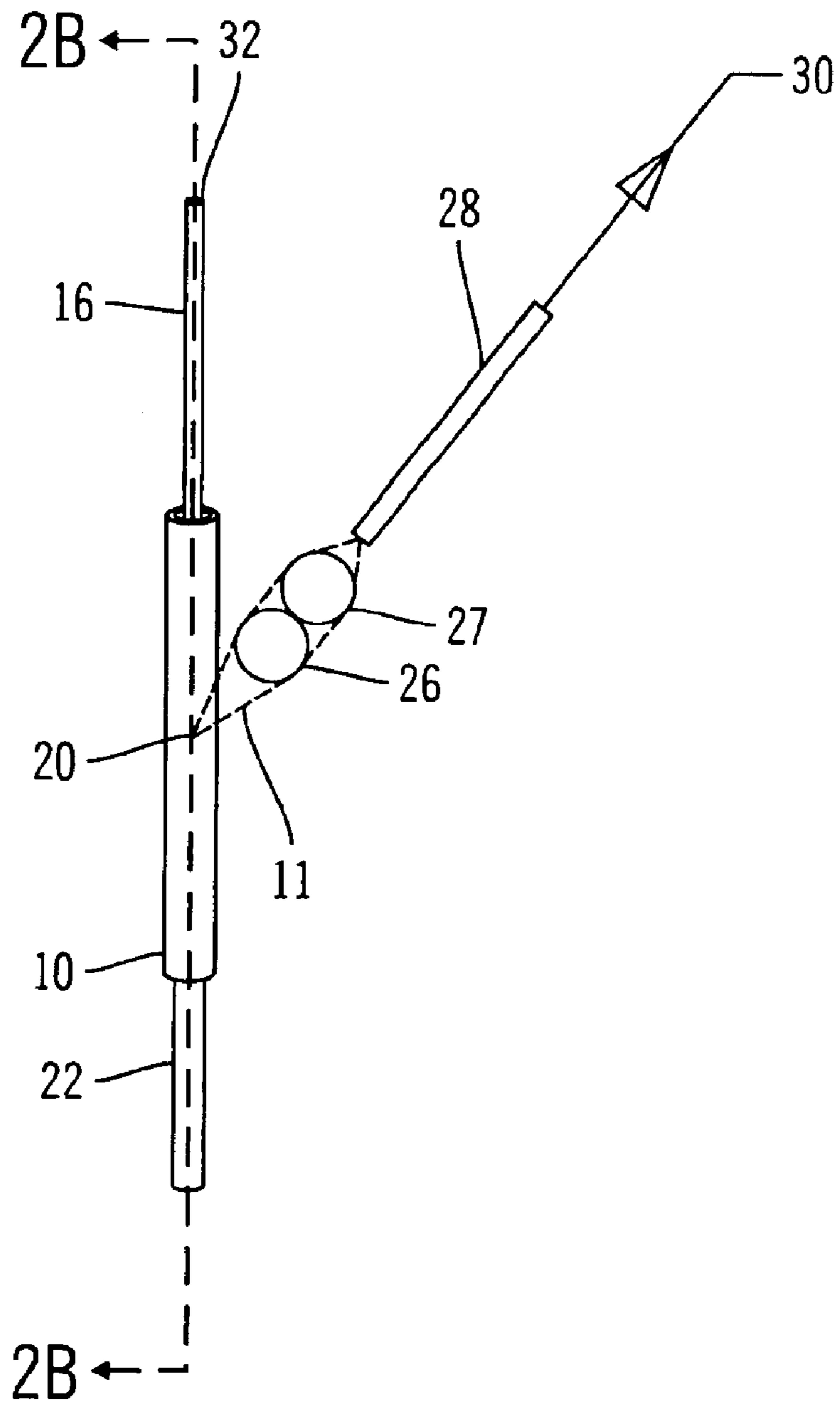
FIG. 2A
