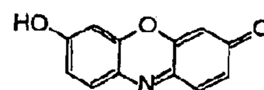
Resorufin (Res)
