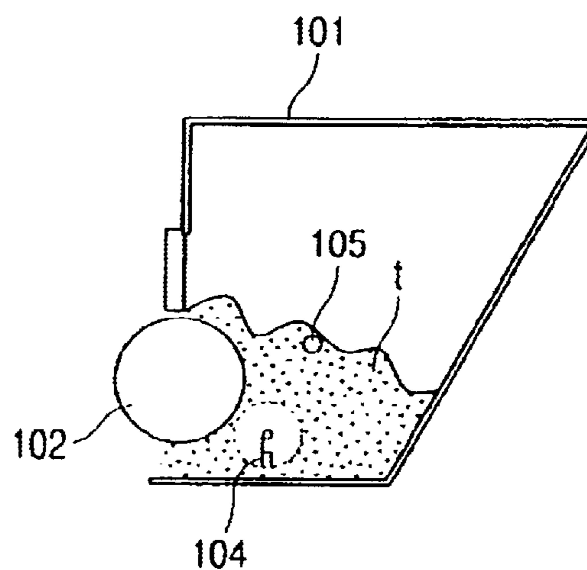
FIG. 7B
