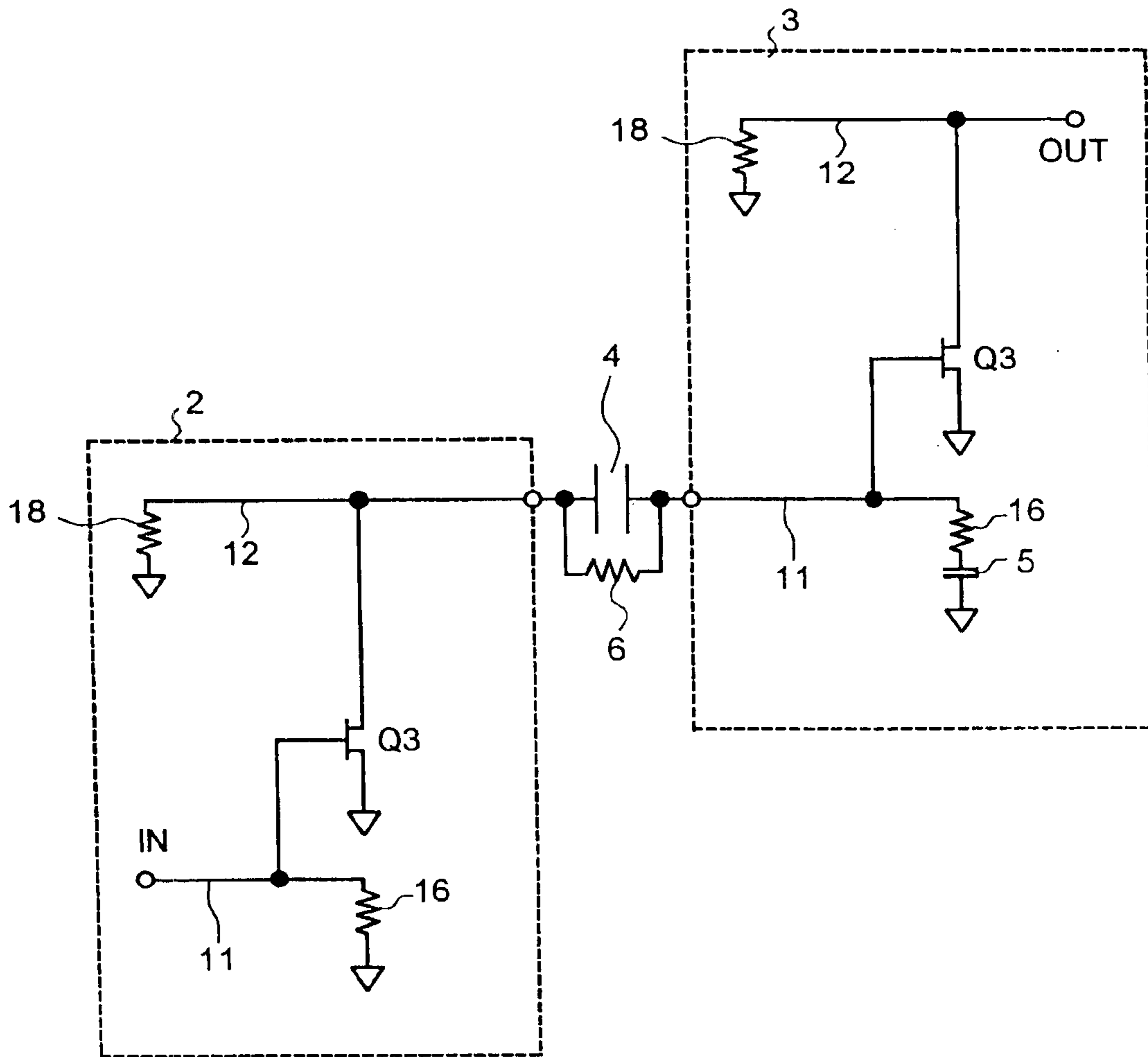
FIG. 10
