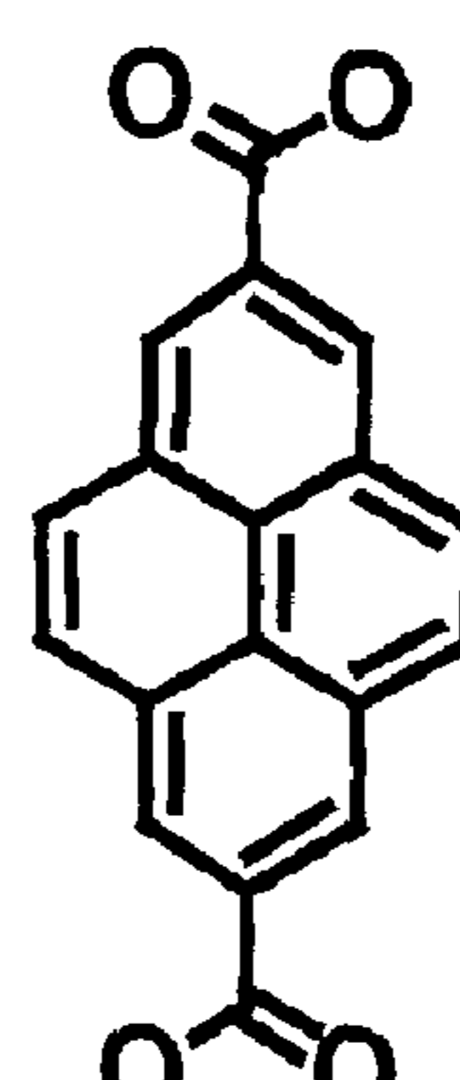
PDC
