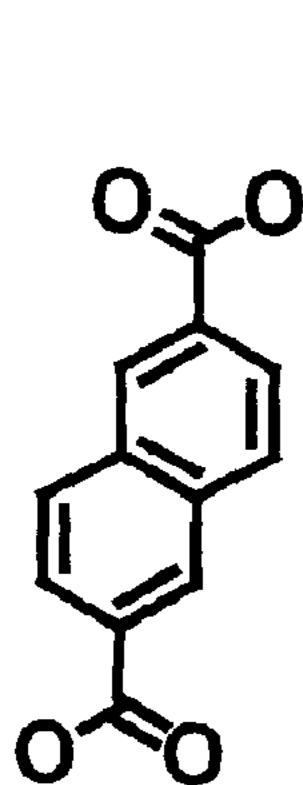
2,6-NDC
