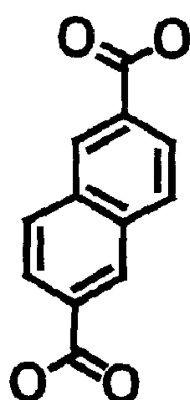
2,6-NDC
