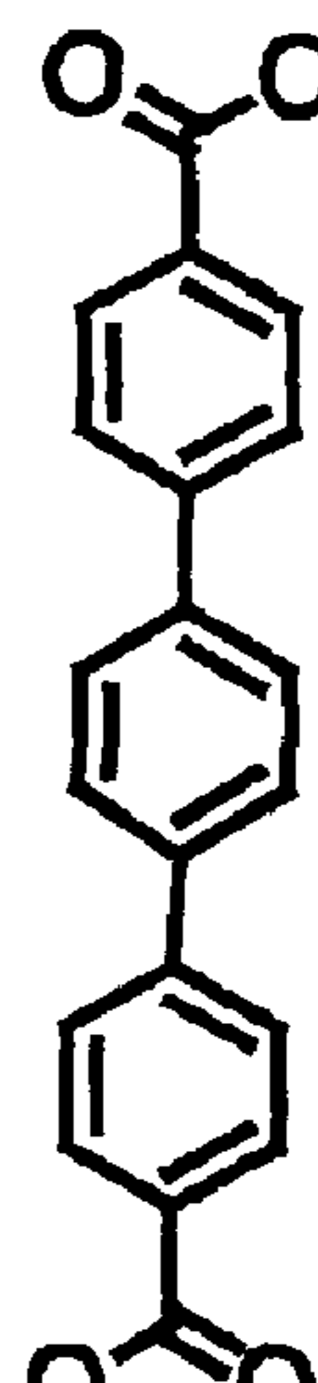
TPDC
