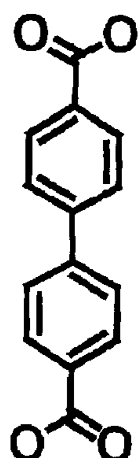
BPDC
