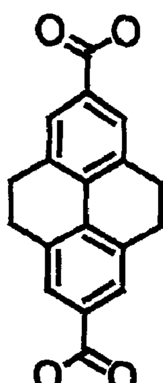
HPDC
