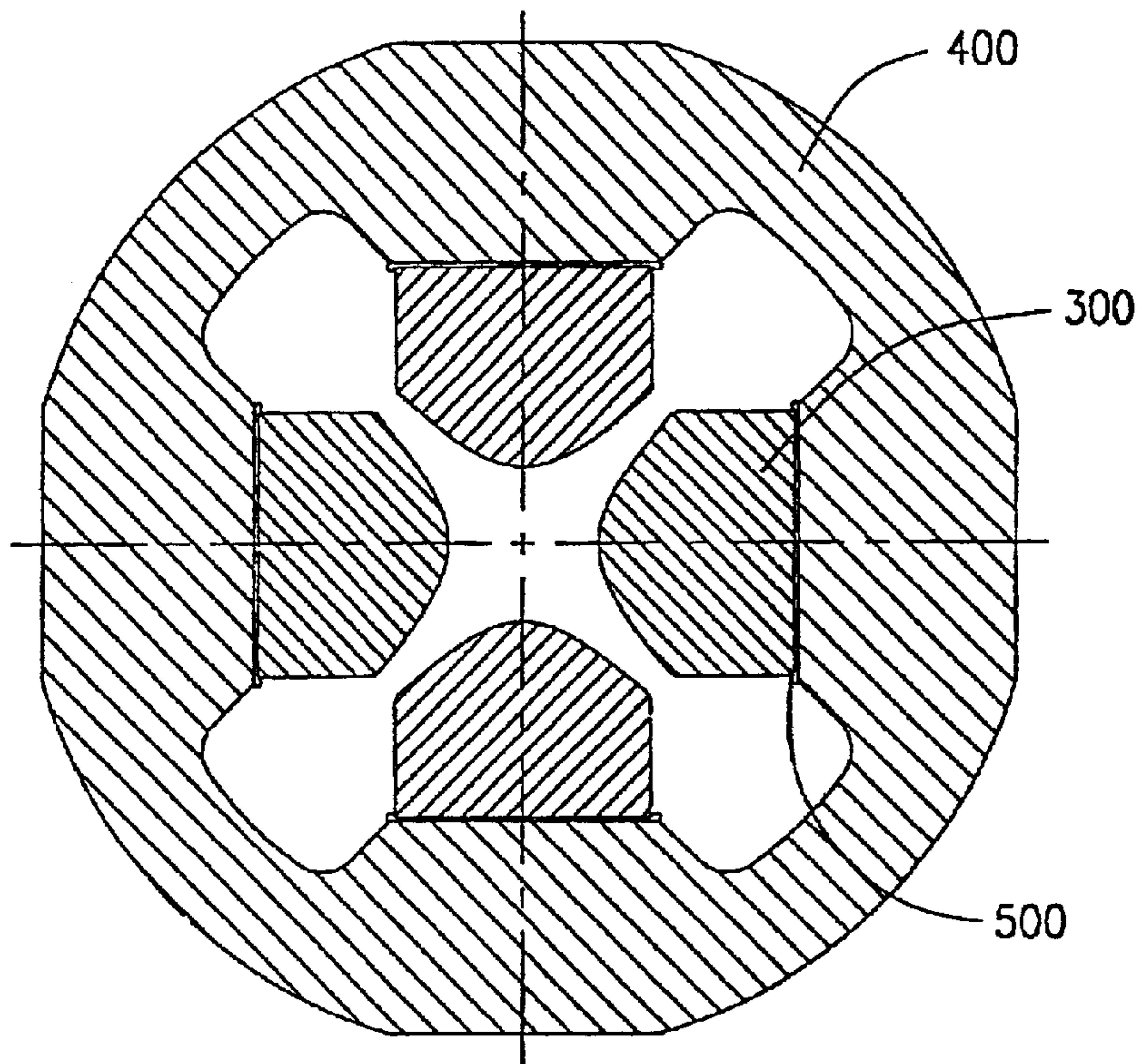
SECTION A-A
