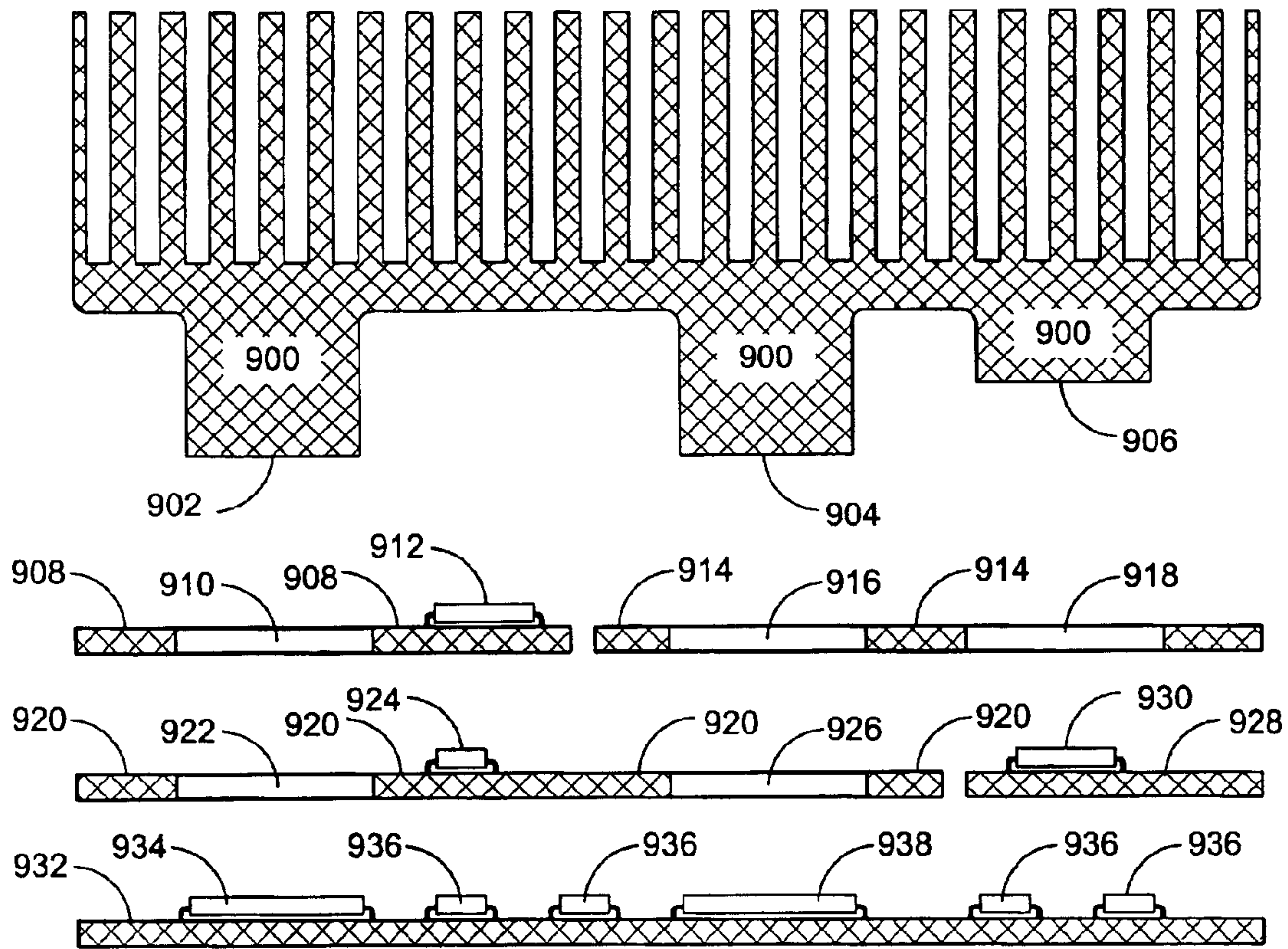
FIG. 9A
