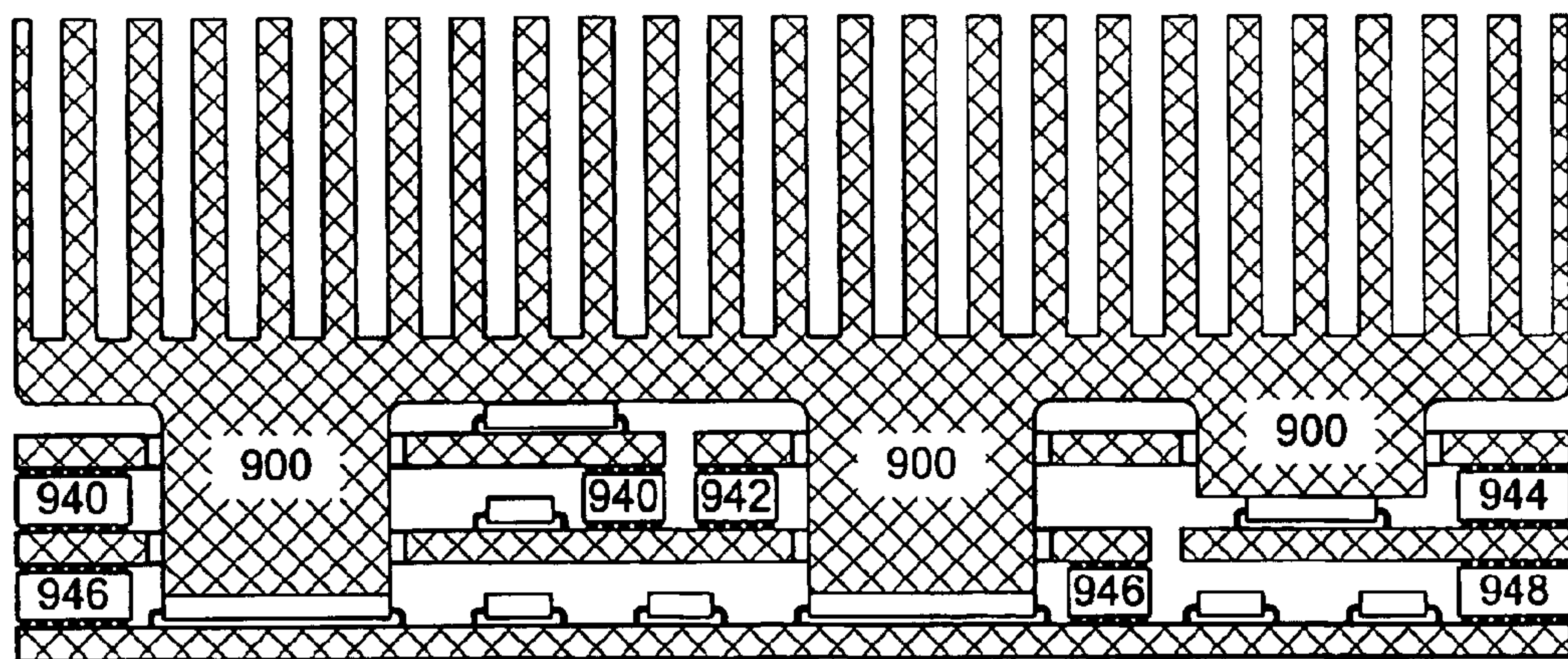
FIG. 9B
