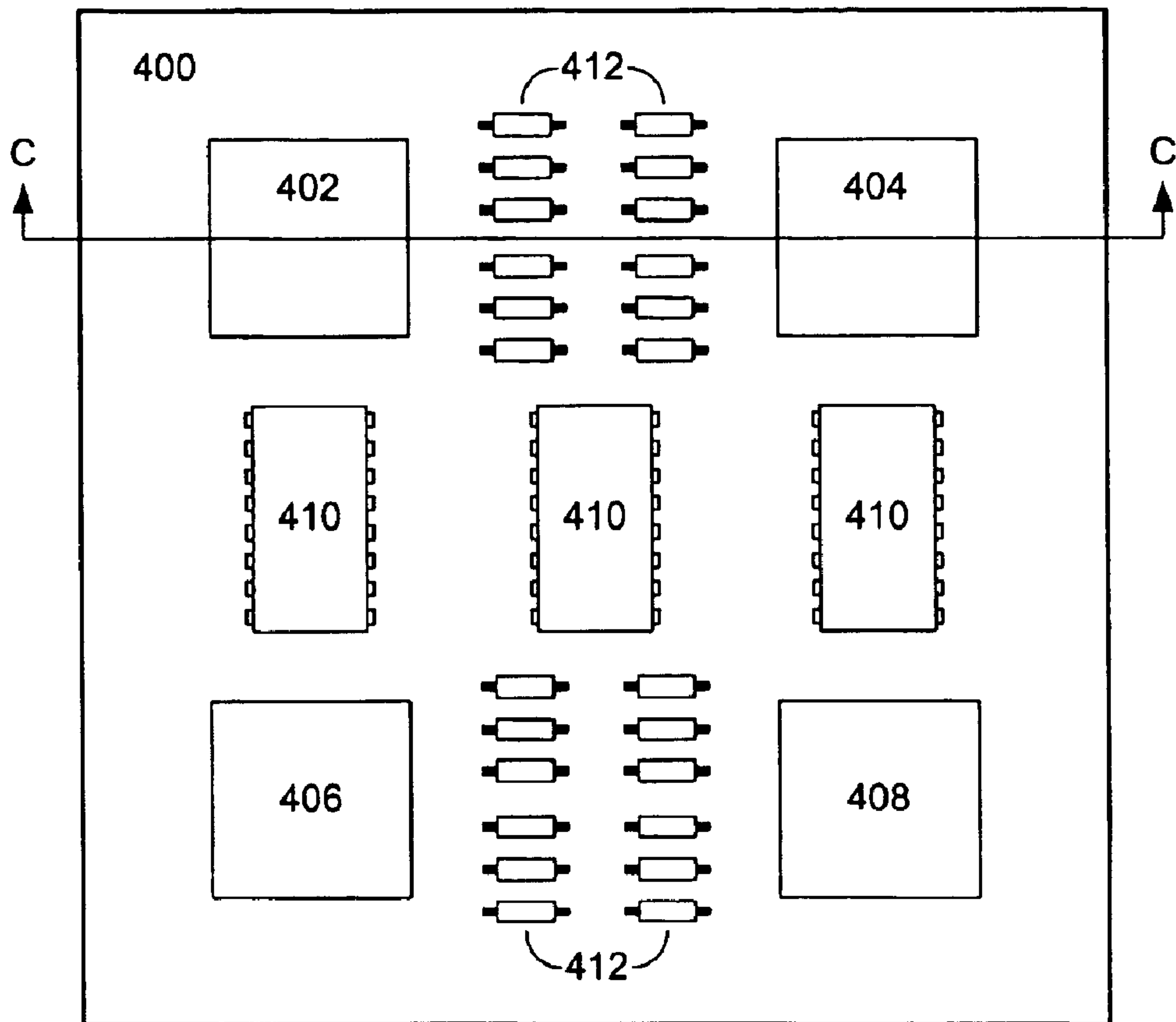
FIG. 4A
