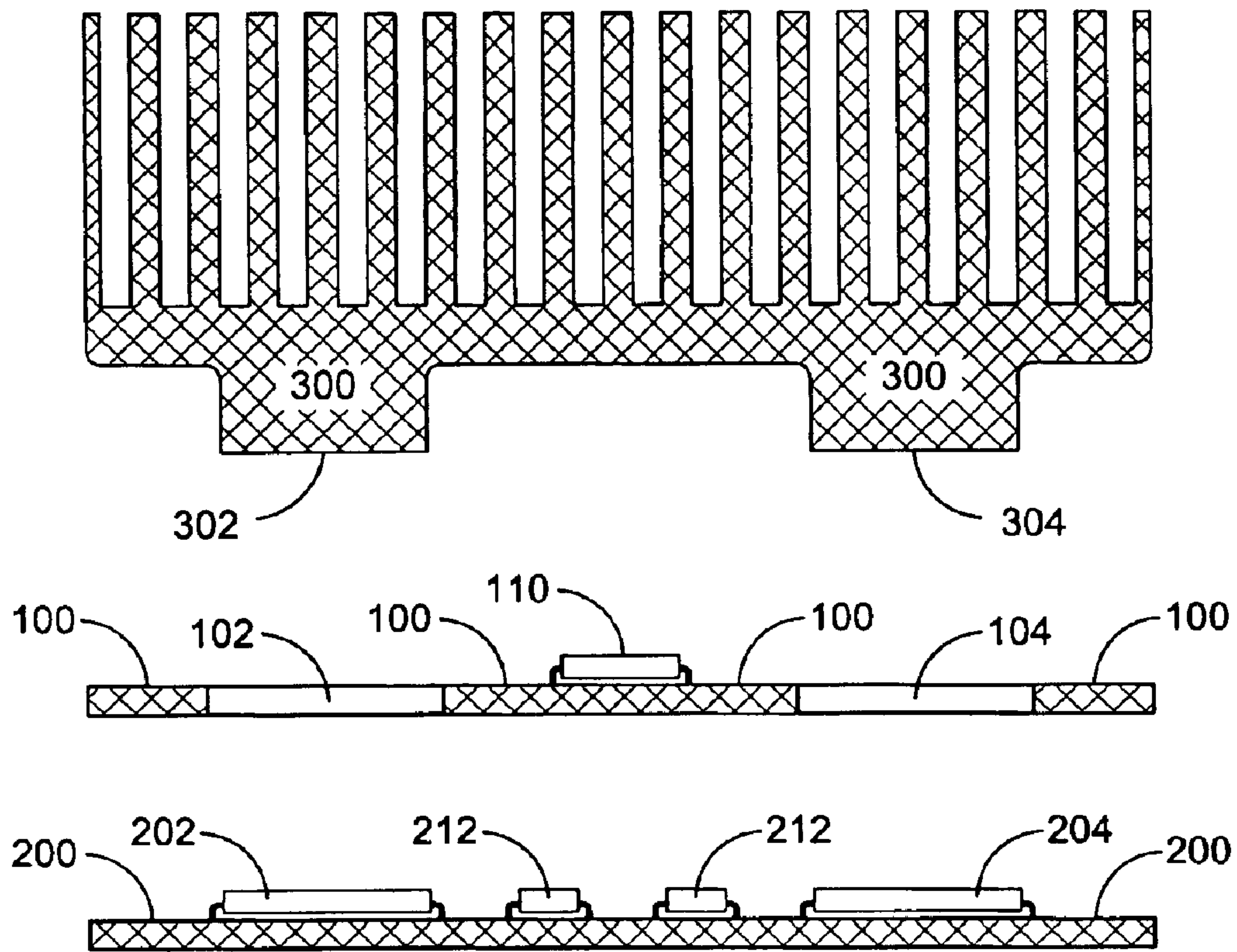
FIG. 3A
