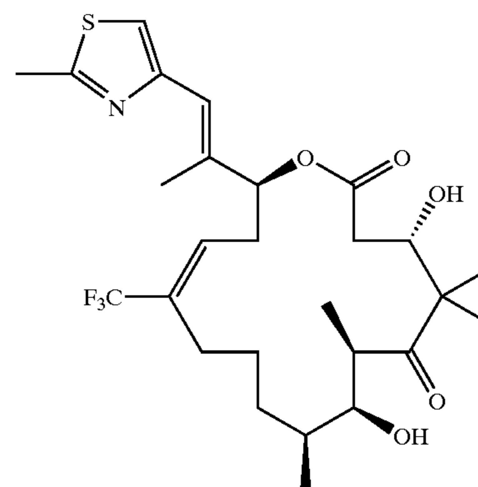
26-F 3 -[16]dEpoB
