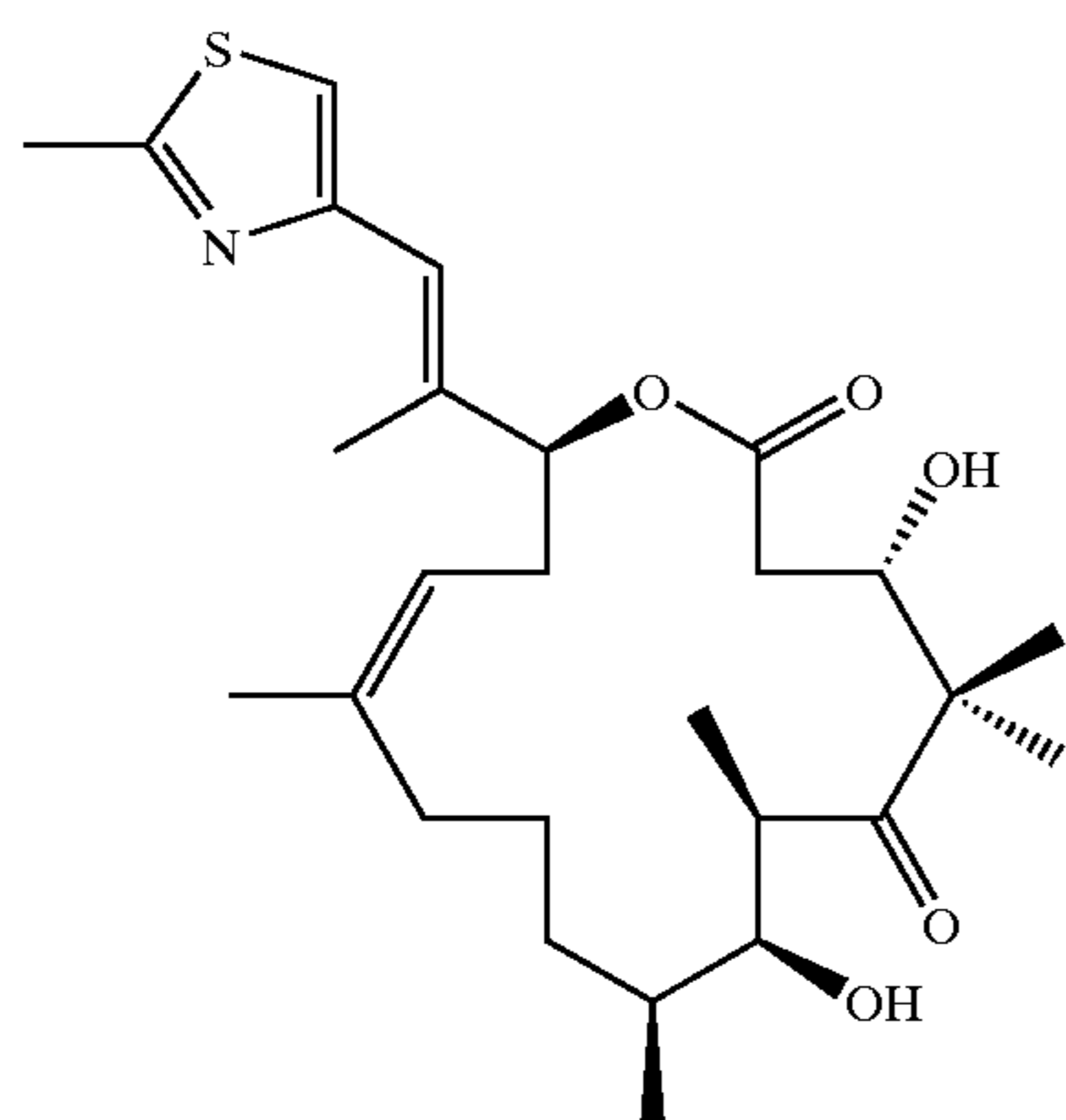
dEpoB (1)
