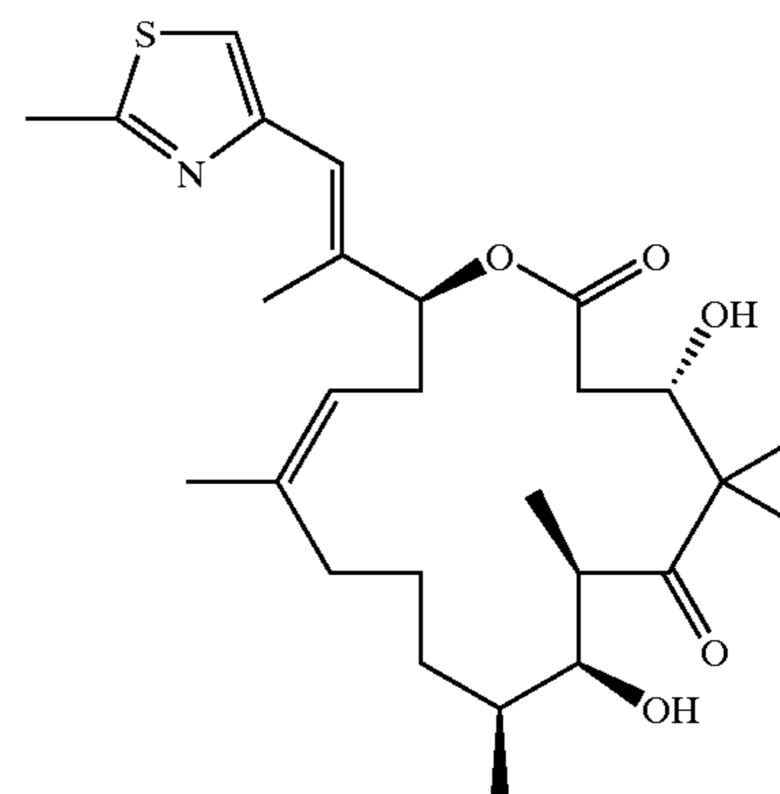
[16]dEpoB
