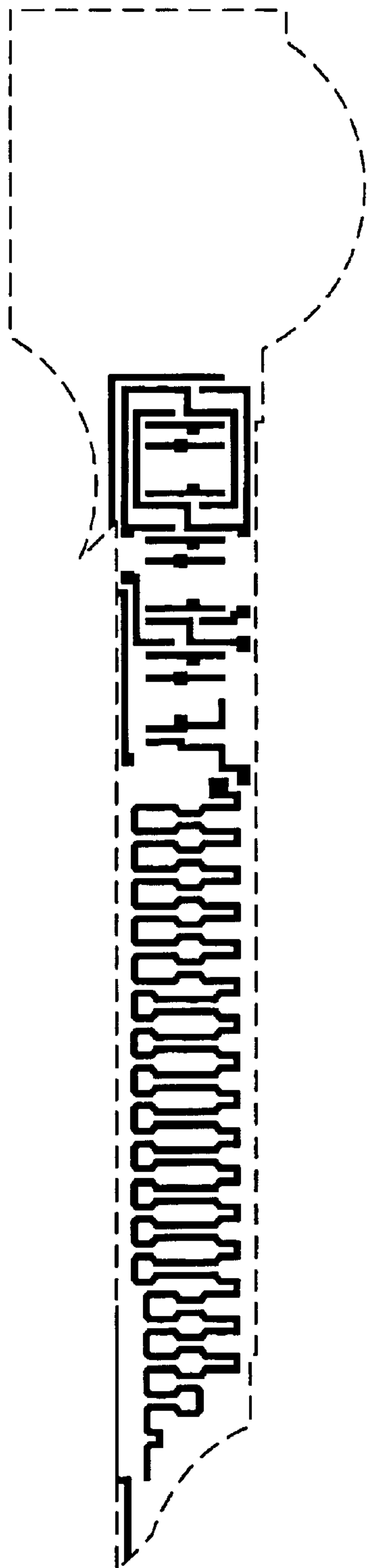
Poly mask
