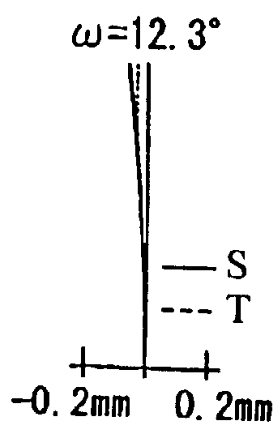
Astigmatism Fig. 3B
