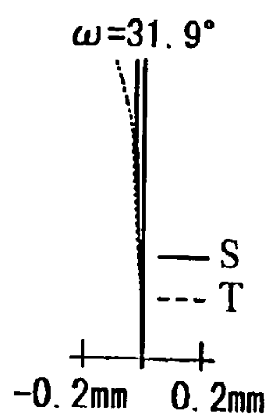
Astigmatism Fig. 2B
