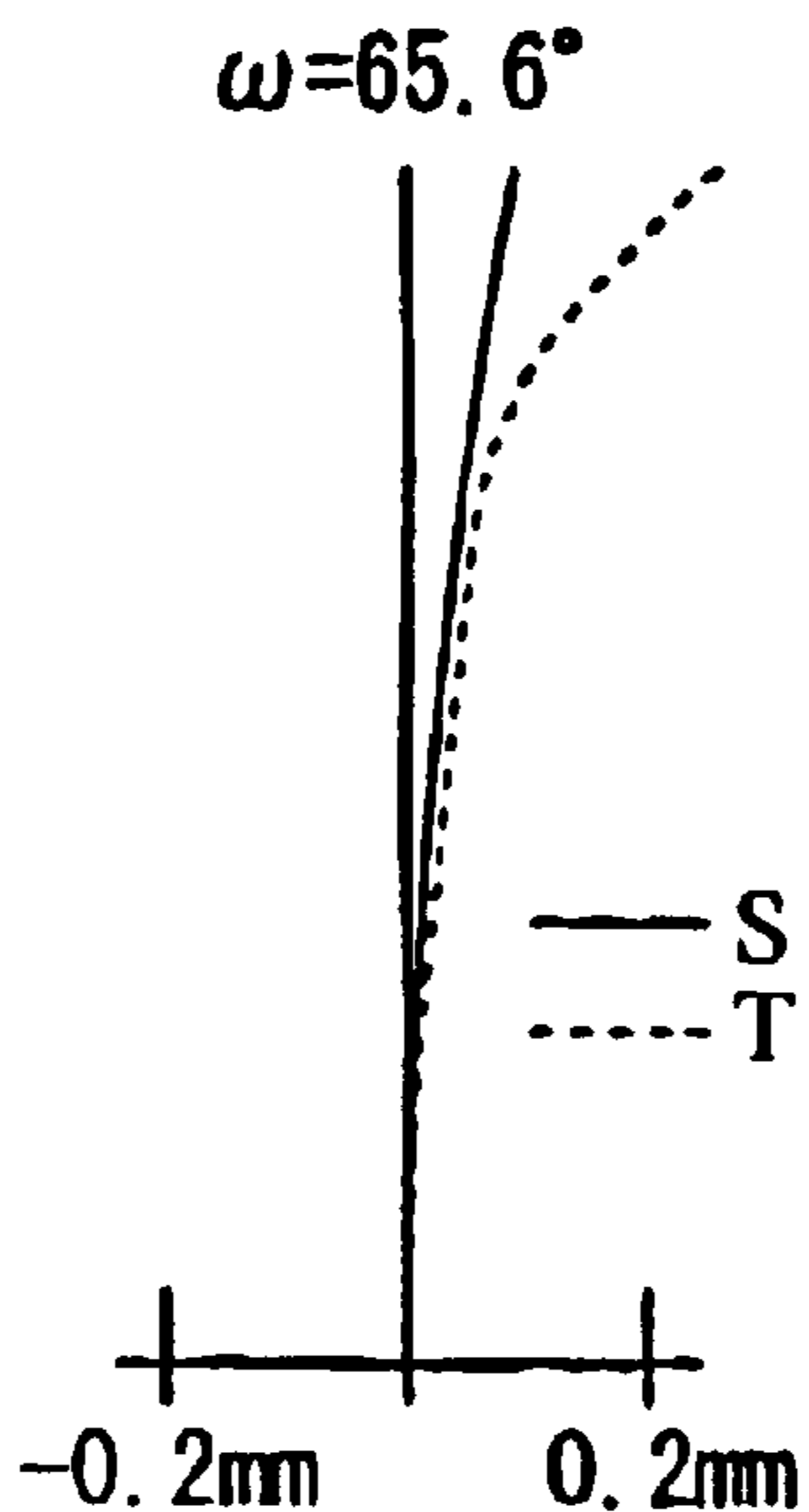
Astigmatism Fig. 8B
