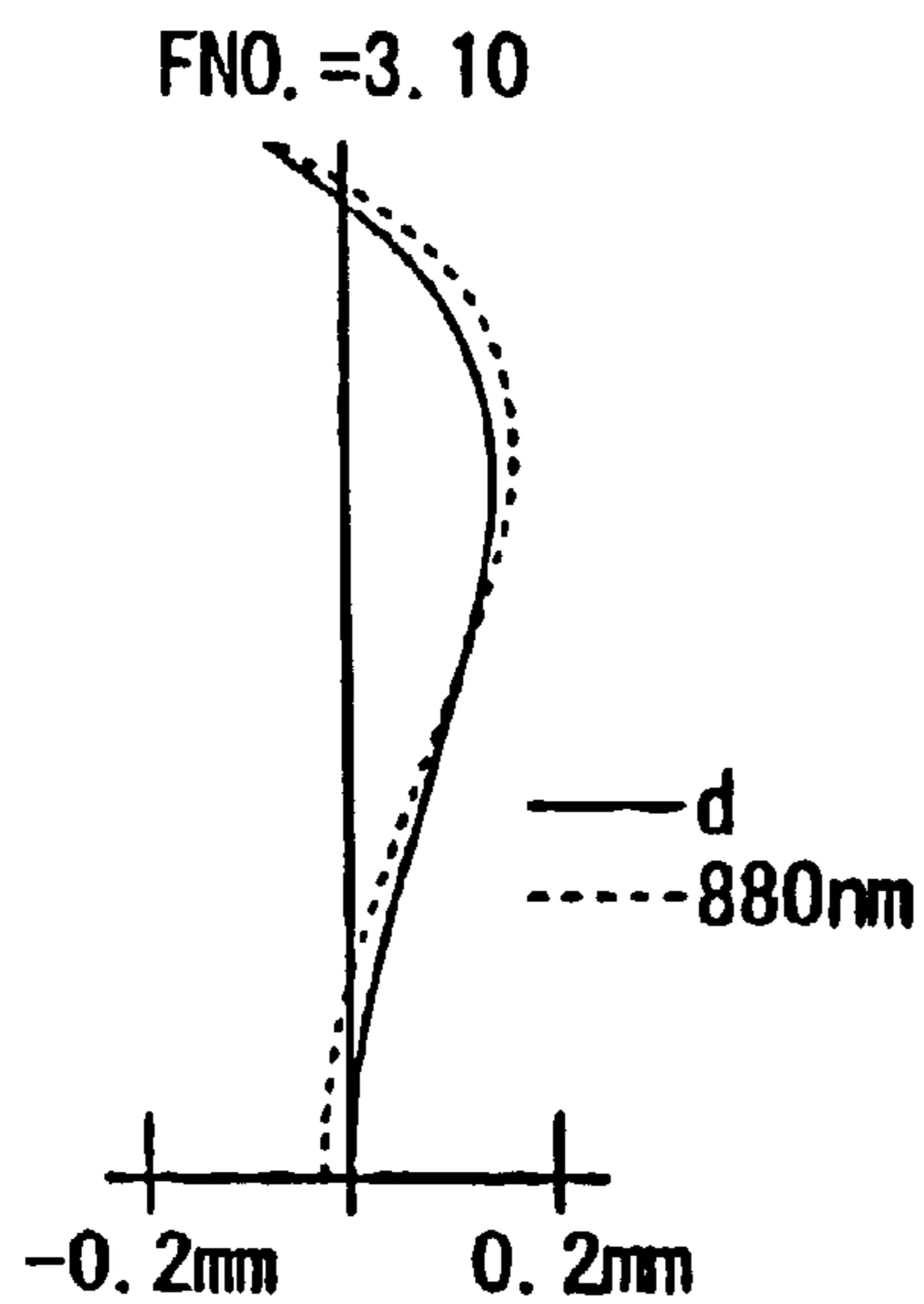
Spherical Aberration Fig. 9A
