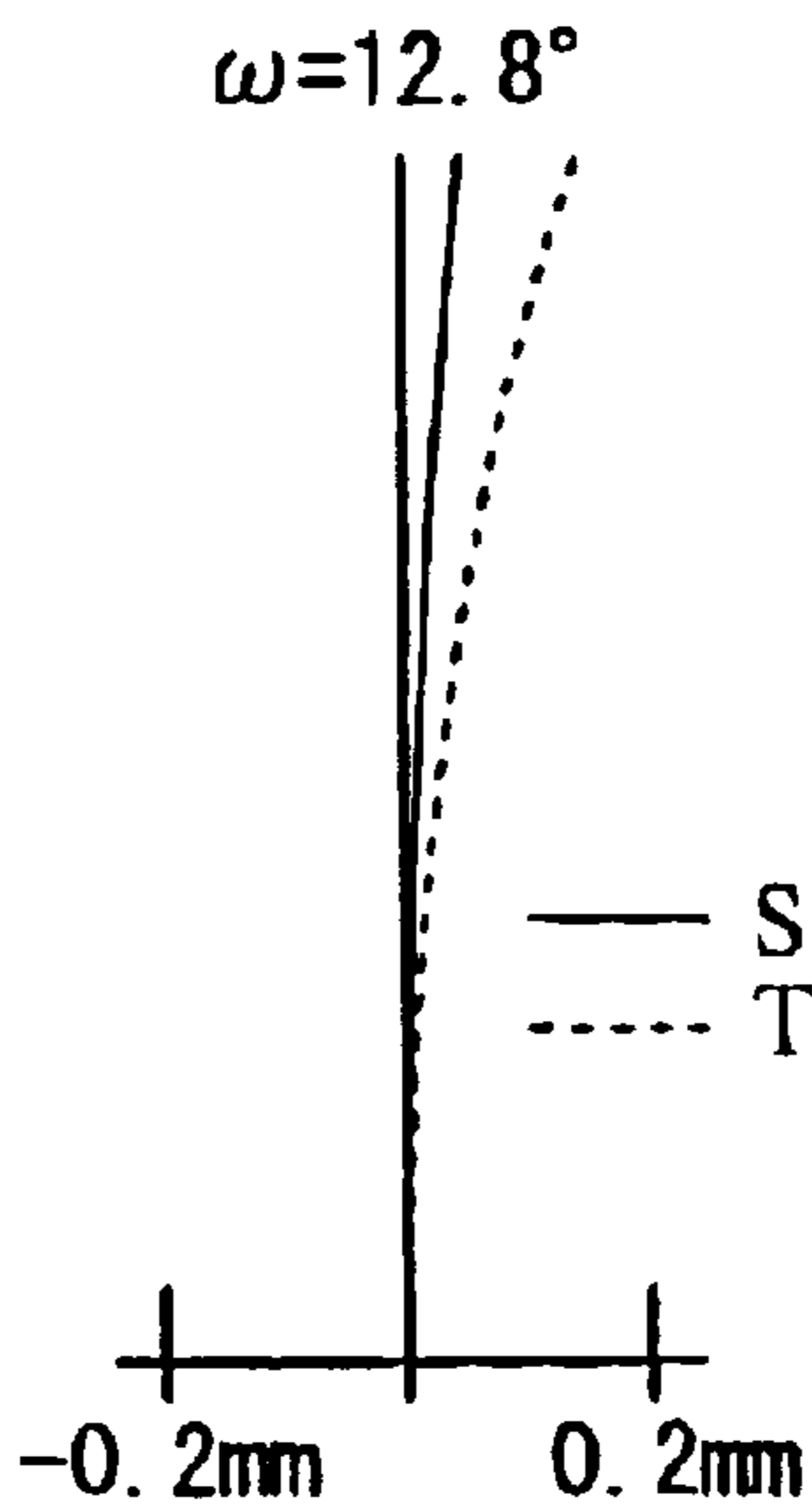
Astigmatism Fig. 7B
