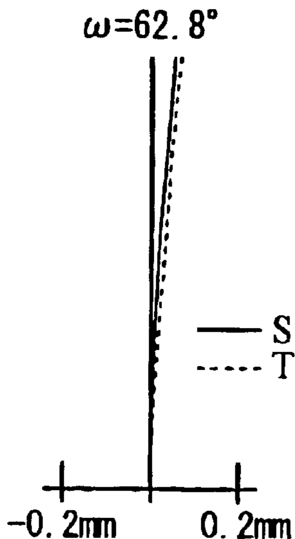
Astigmatism Fig. 2B
