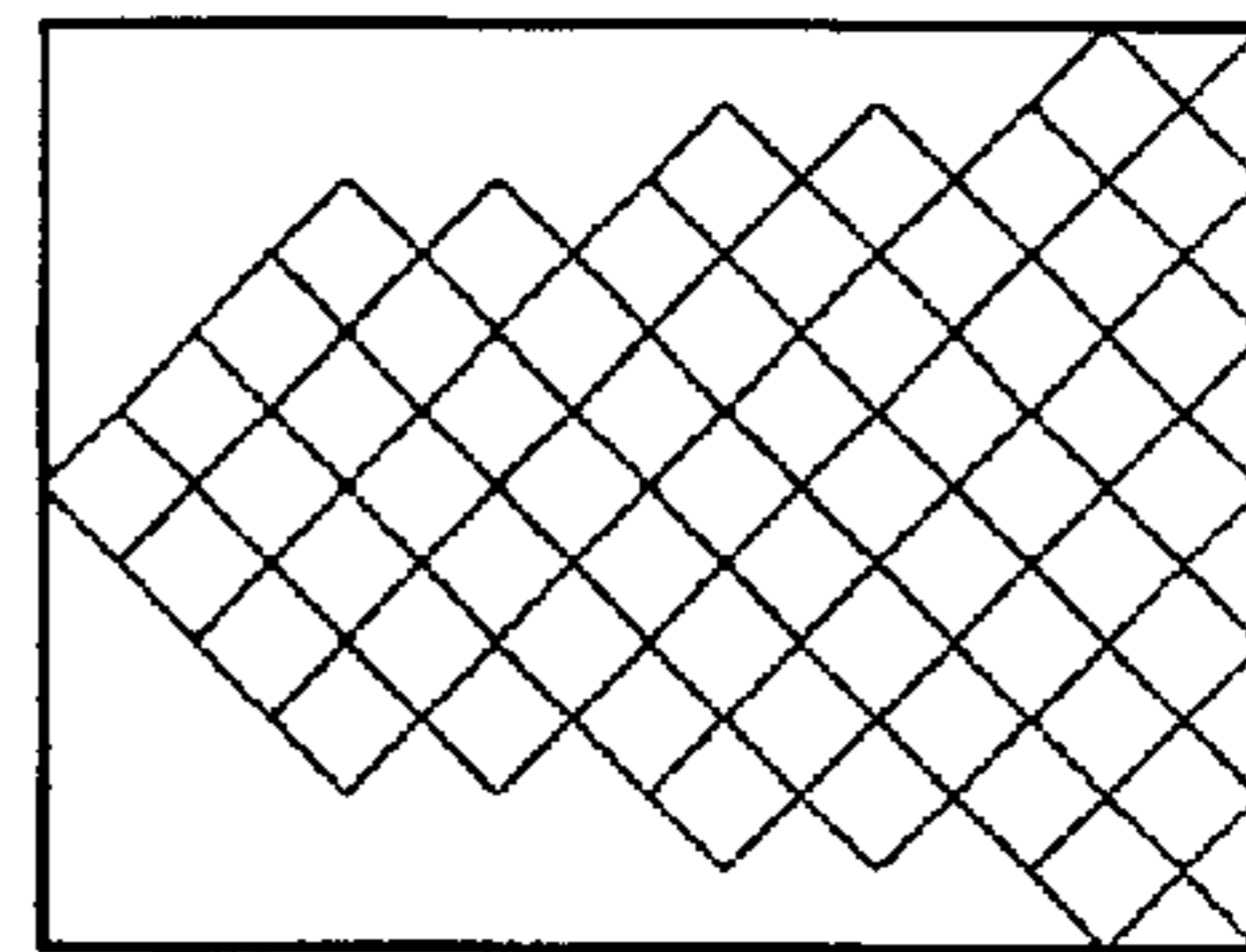
IMAGE B(128 × 96)
