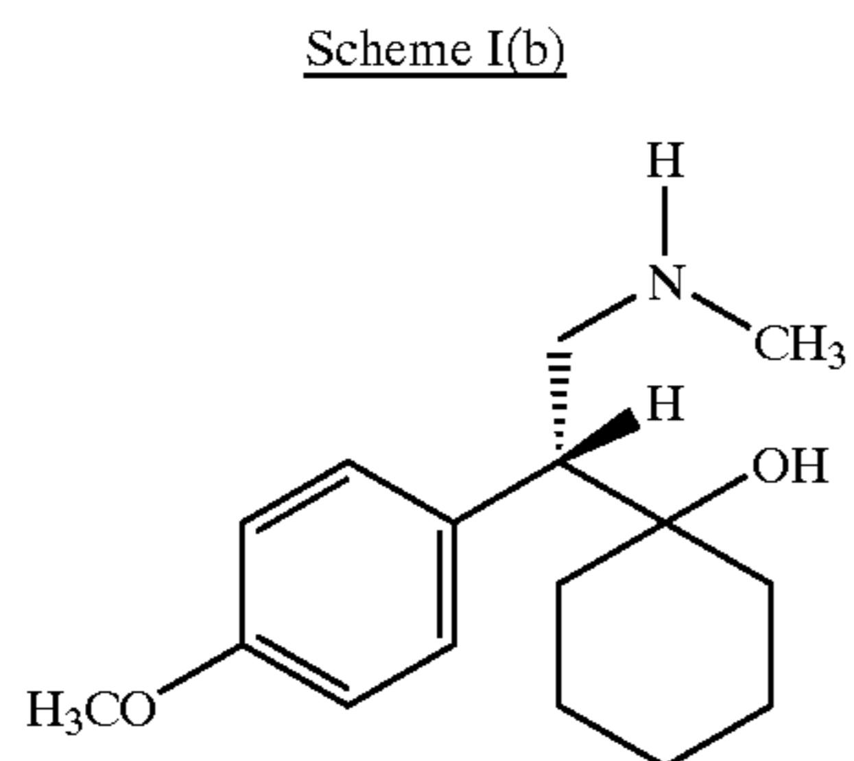
(-)-N-desmethylvenlafaxine
