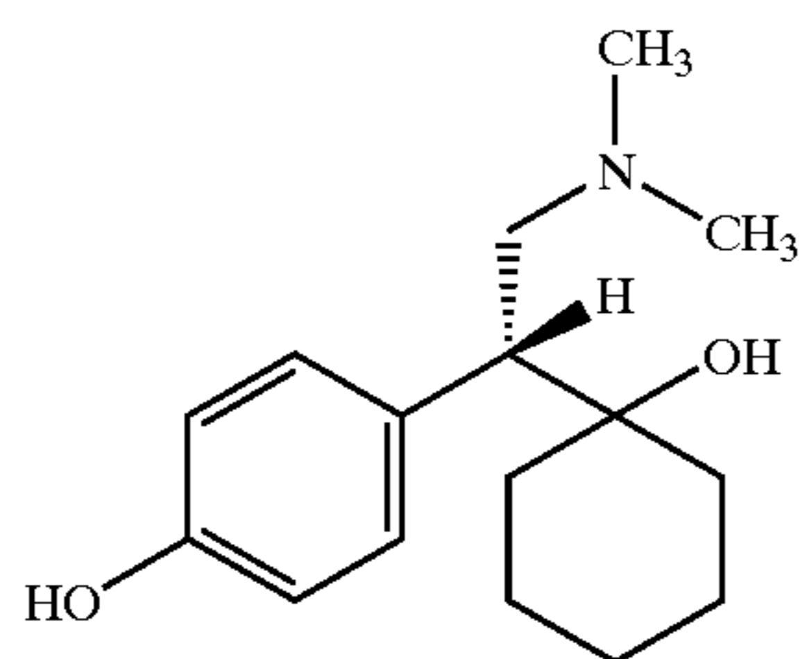
(-)-O-desmethylvenlafaxine
