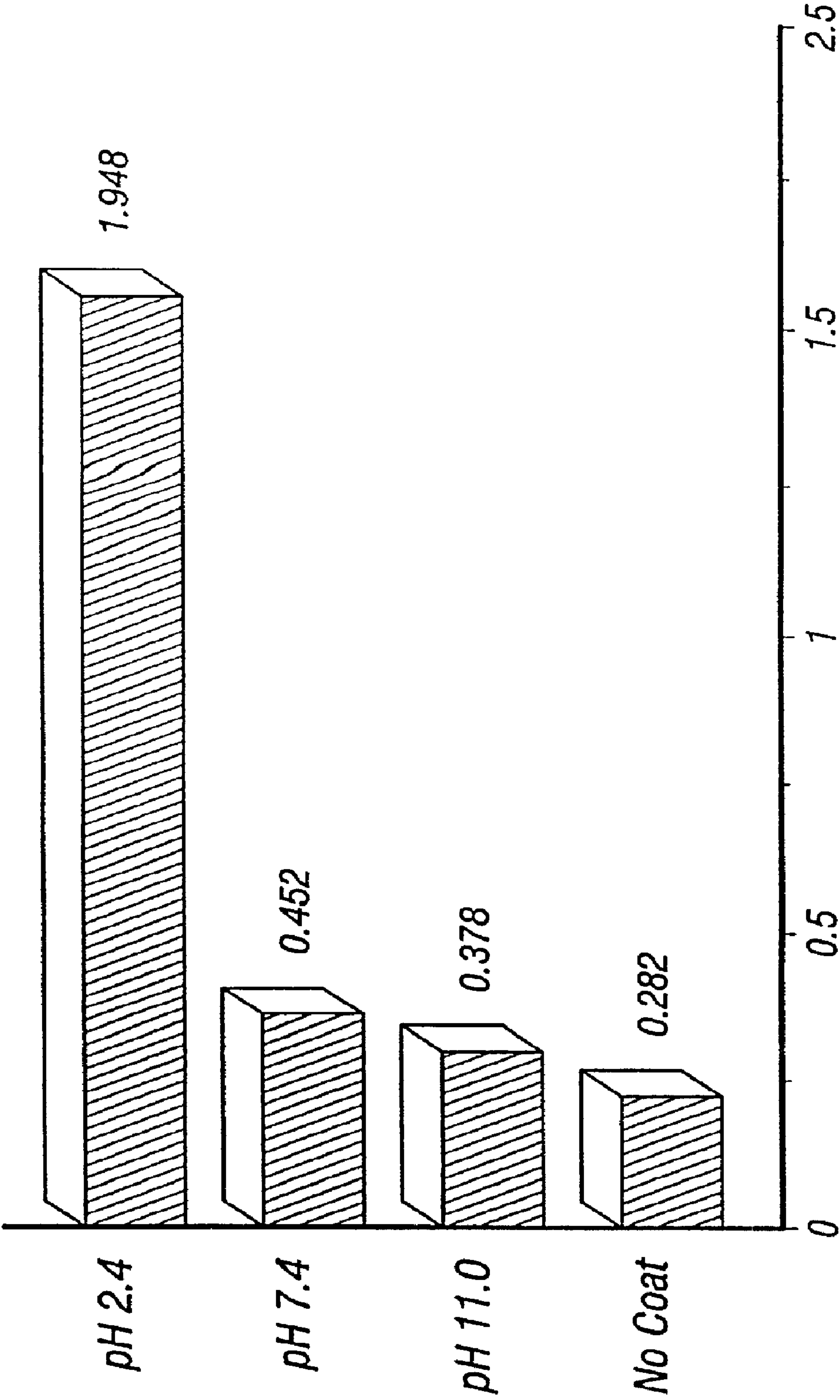
OD @ 280 nM
