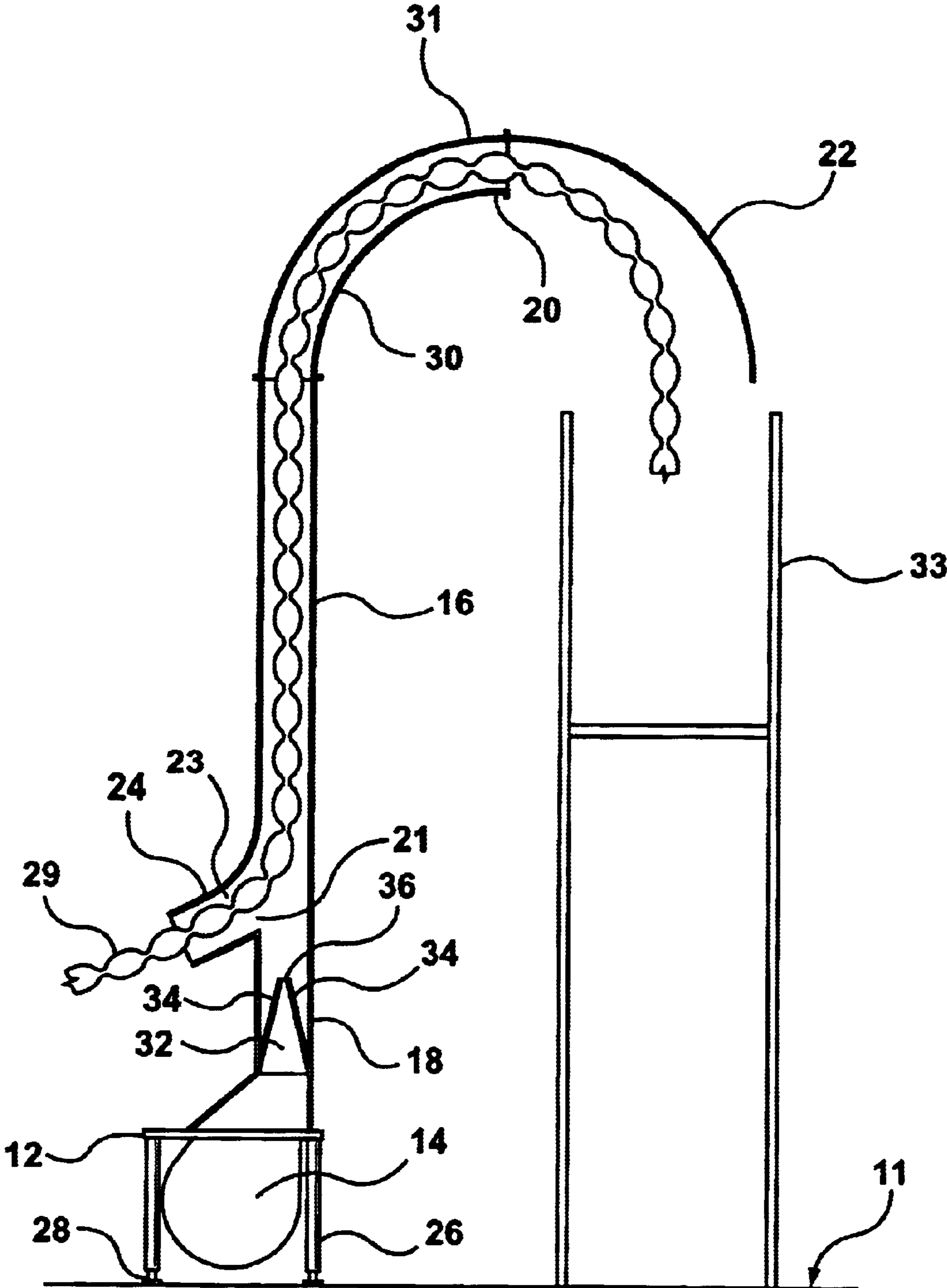
Section A-A
