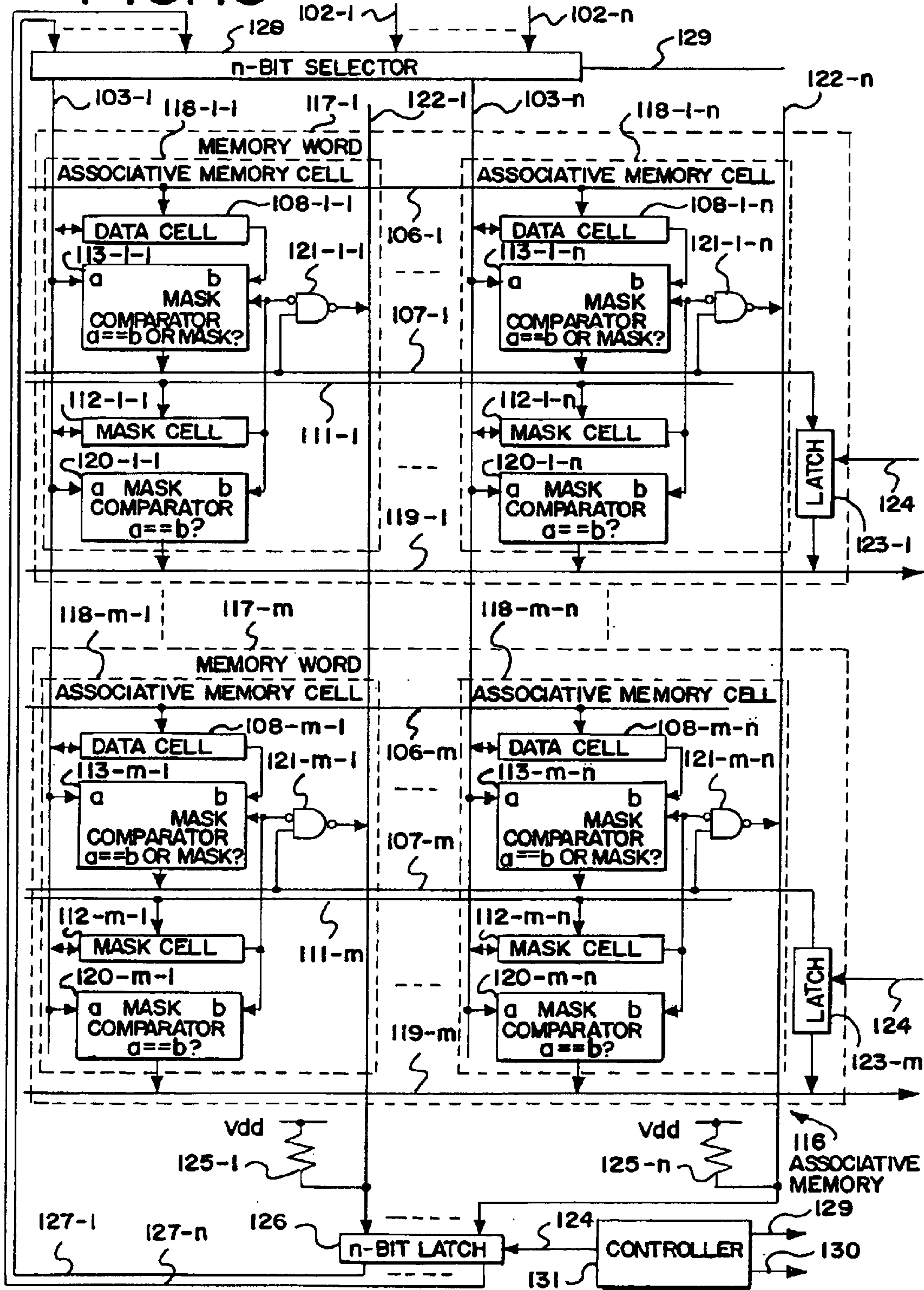
FIG. 15
