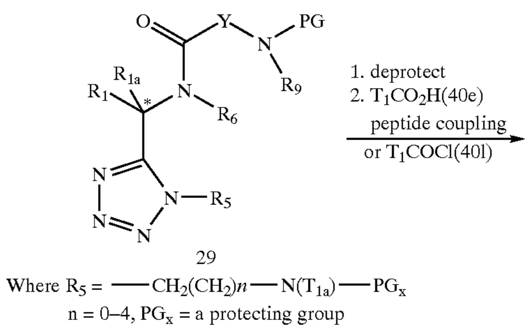
Scheme 3e
