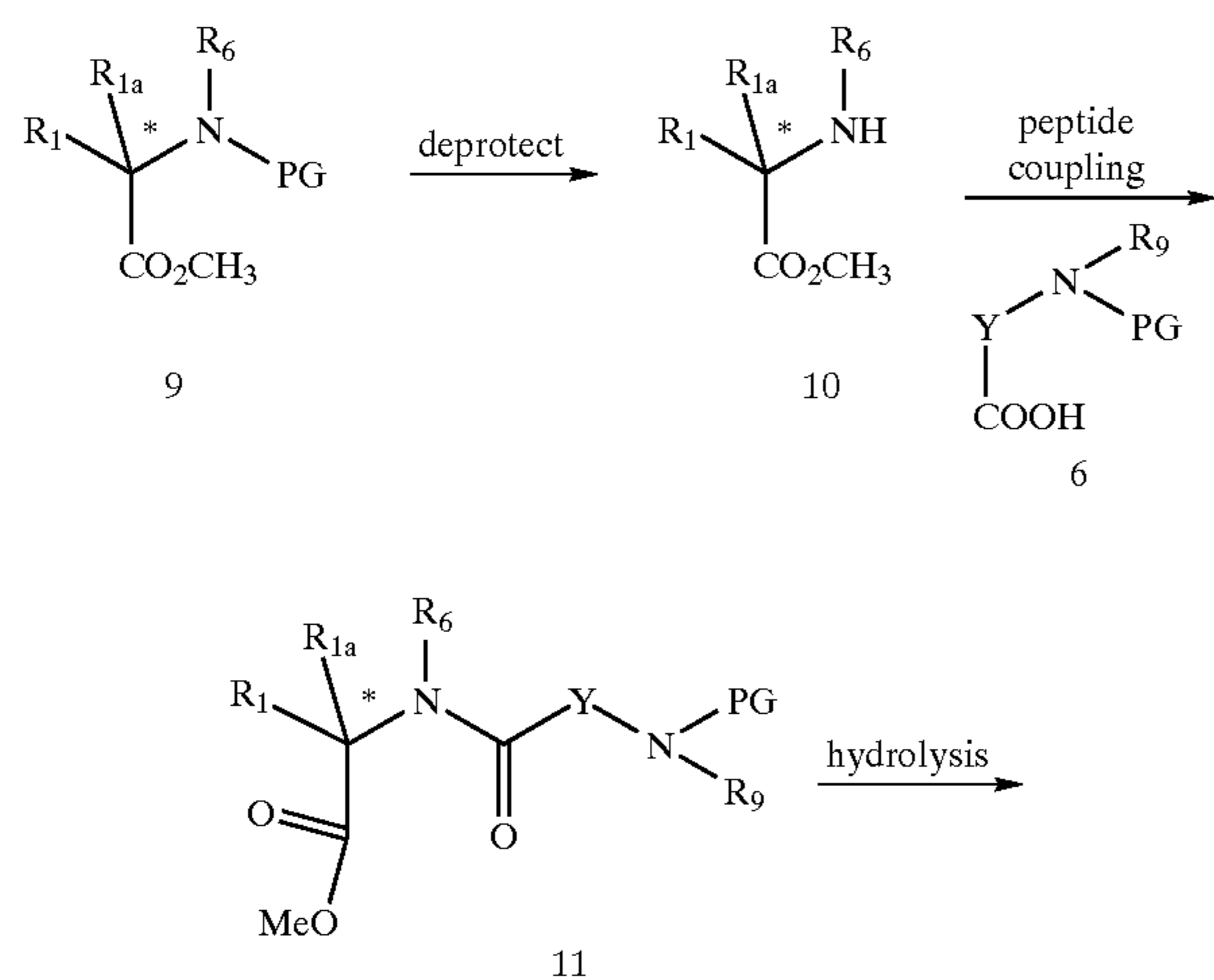
Scheme 1a
