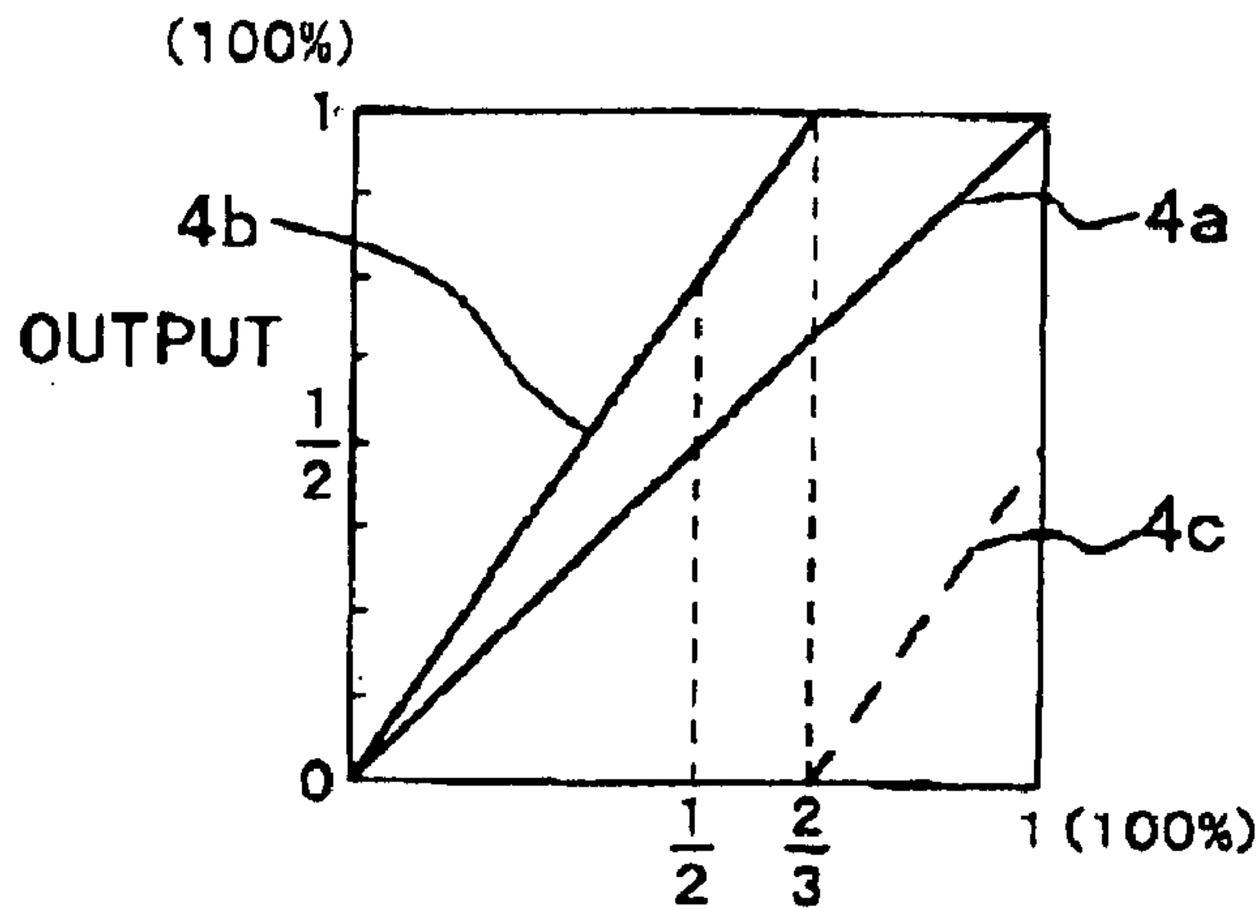
gamma-CORRECTION CKT
