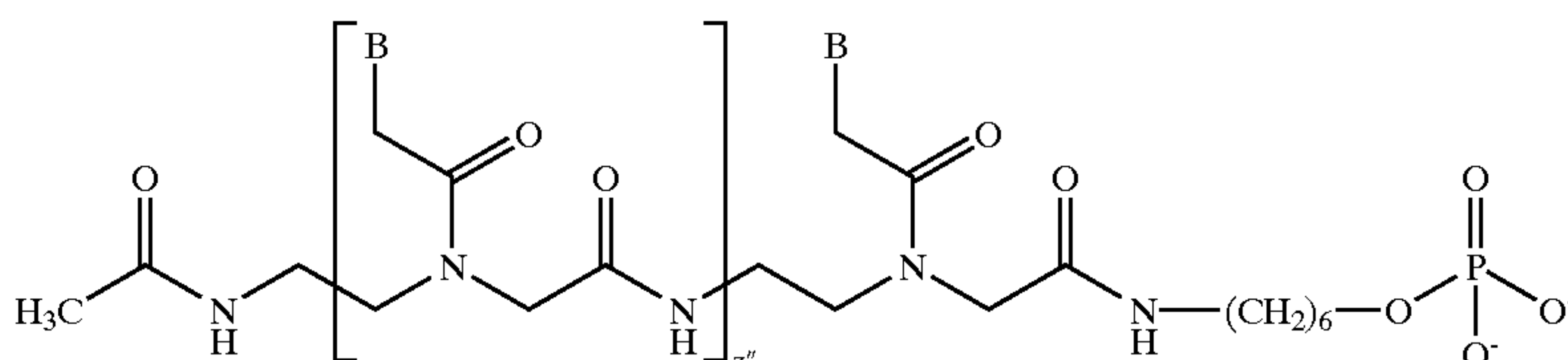
PNA-1:
