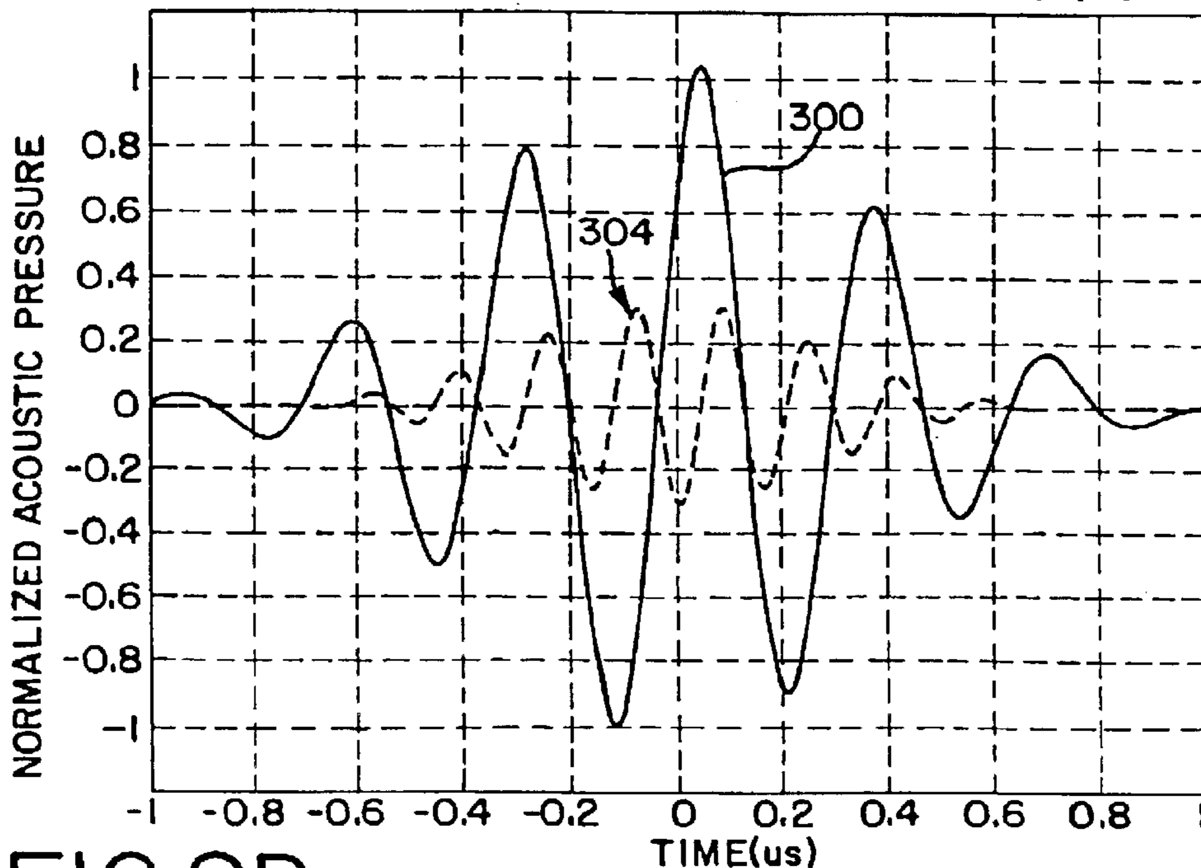
SOURCE WAVEFORM:FUNDAMENTAL(-)AND 2nd HARMONIC(--)-COMPONENTS
