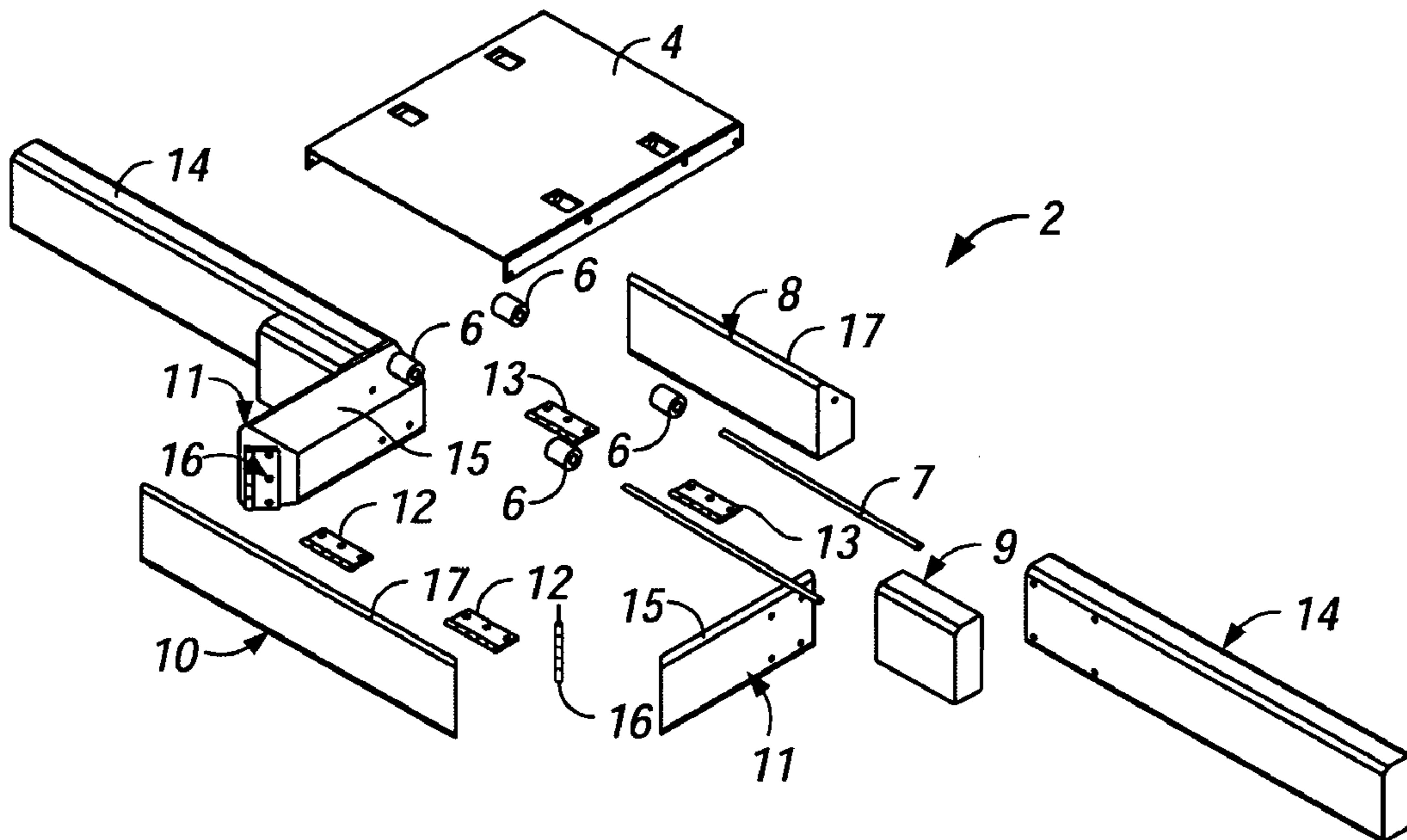
FIG. 2B
