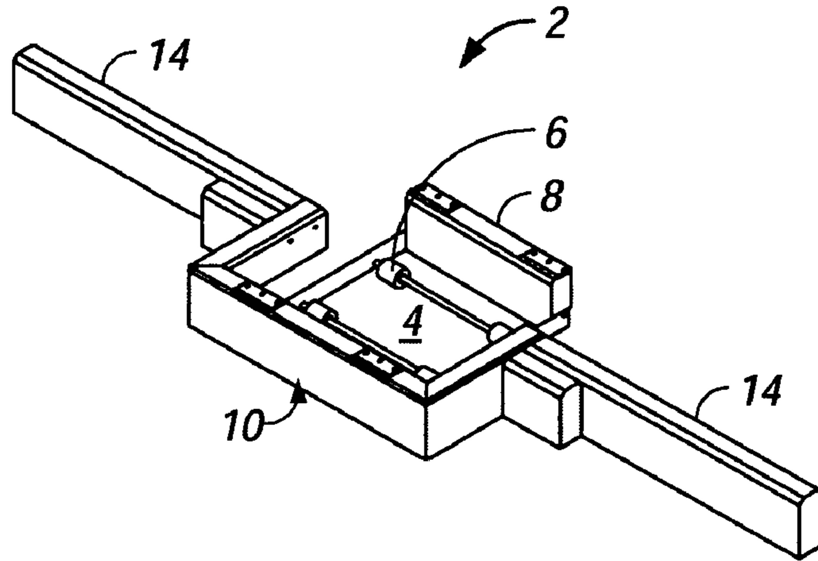
FIG. 2A
