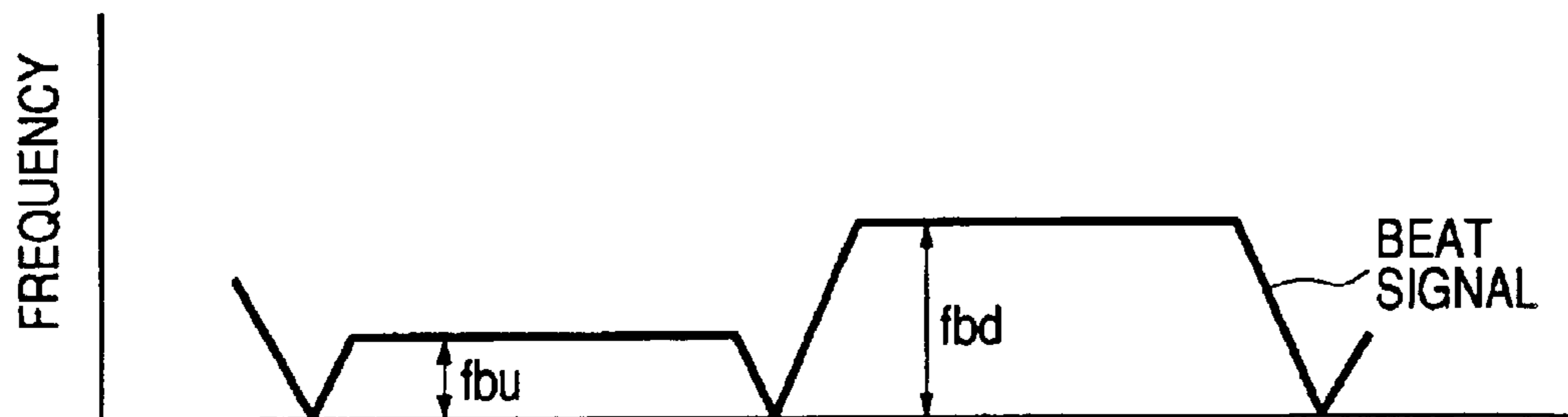
FIG. 7B
