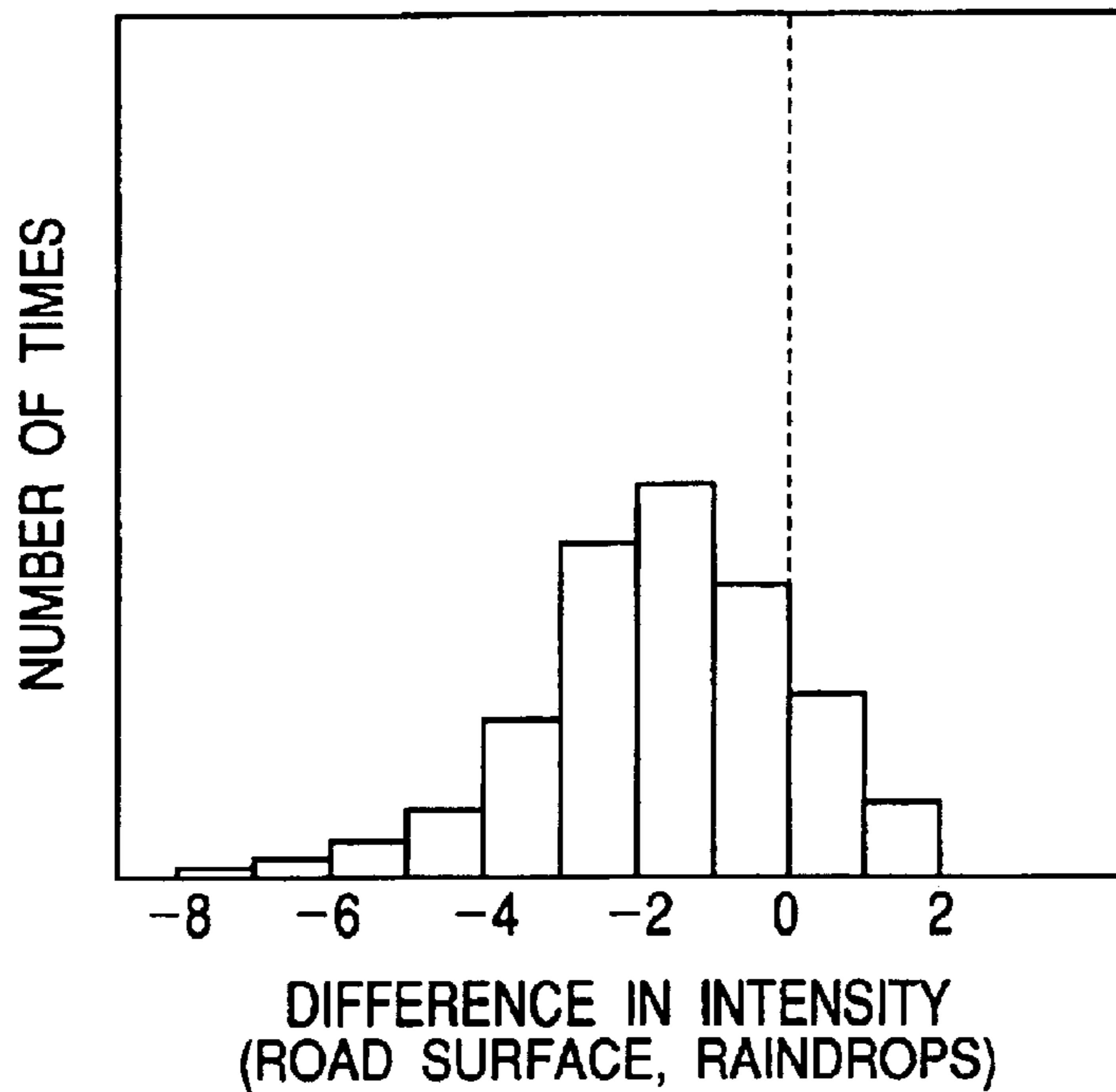
FIG. 6A
