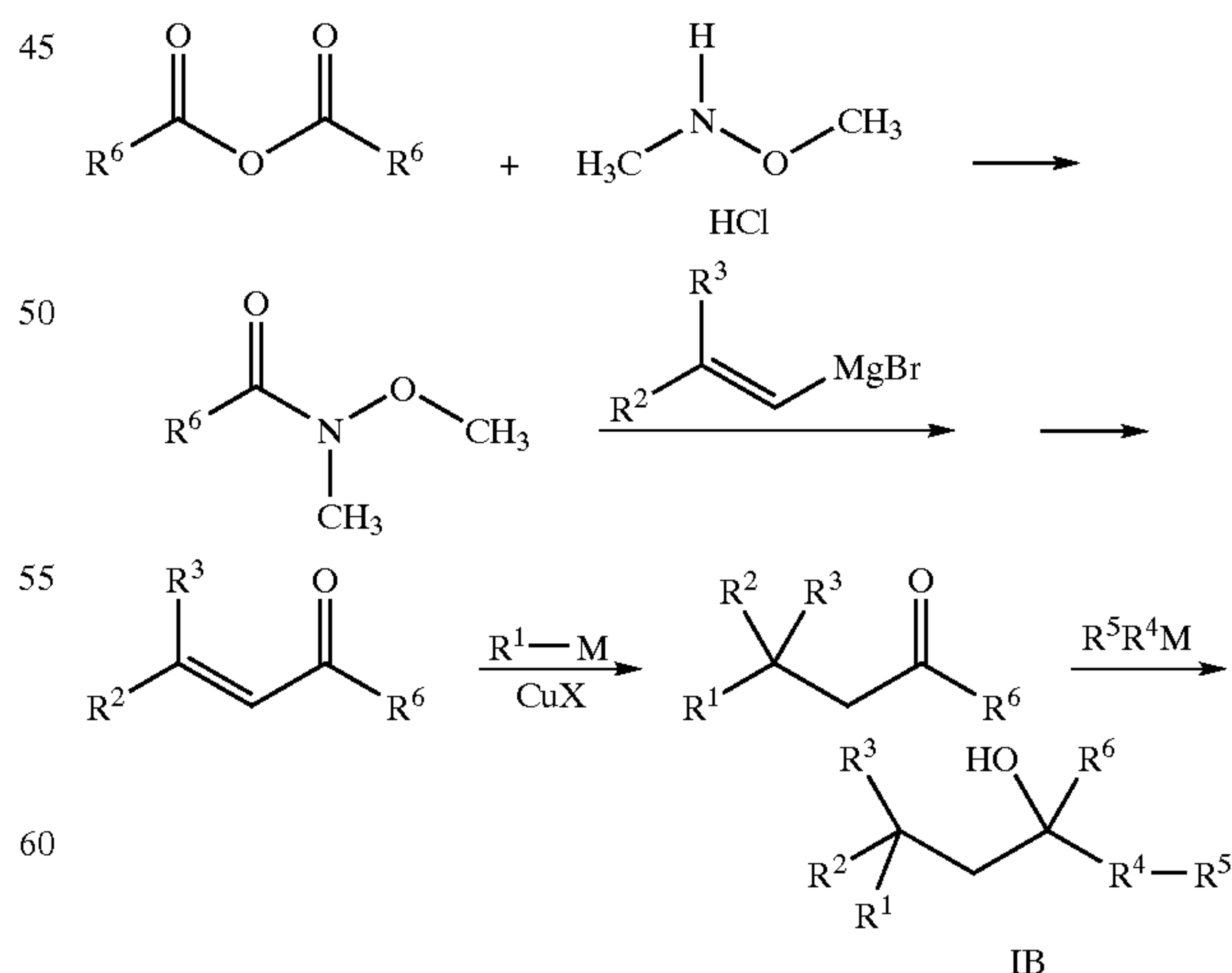
Scheme VI
