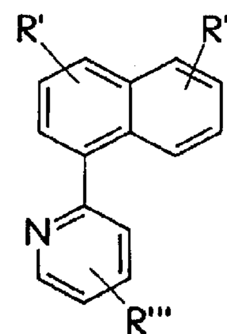
pyridylnaphthalenes
