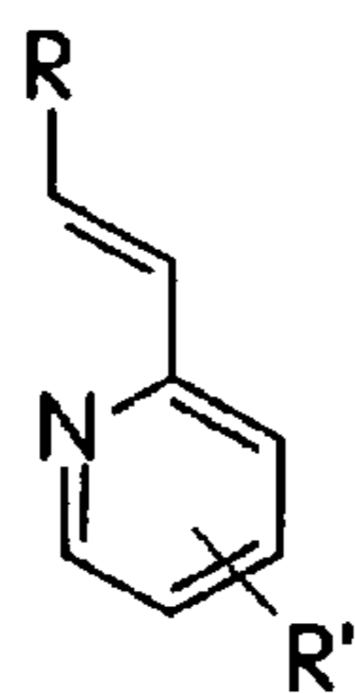
vinylpyridines
