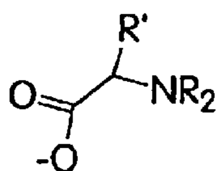
aminoacids
