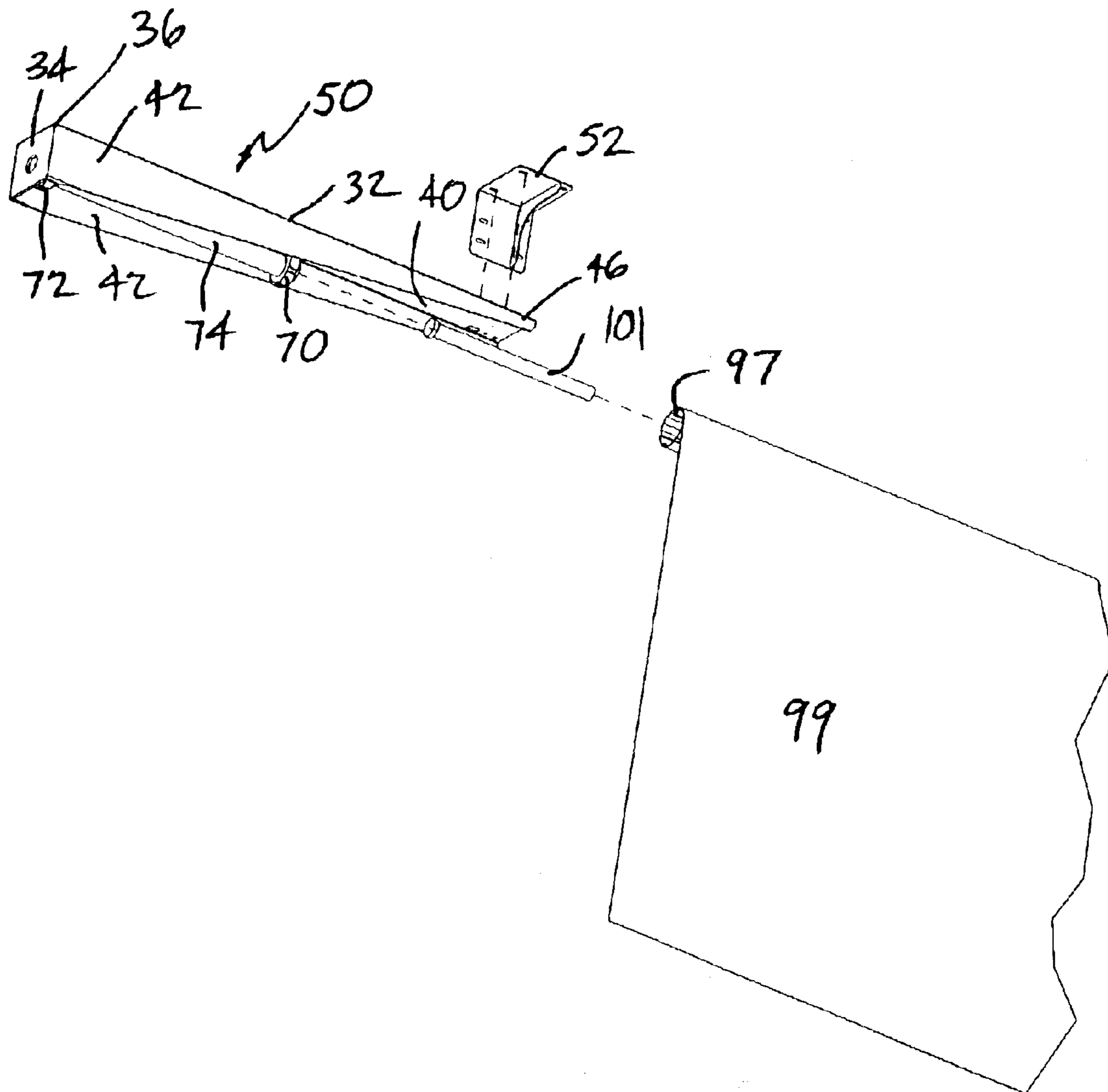
FIG. 17
