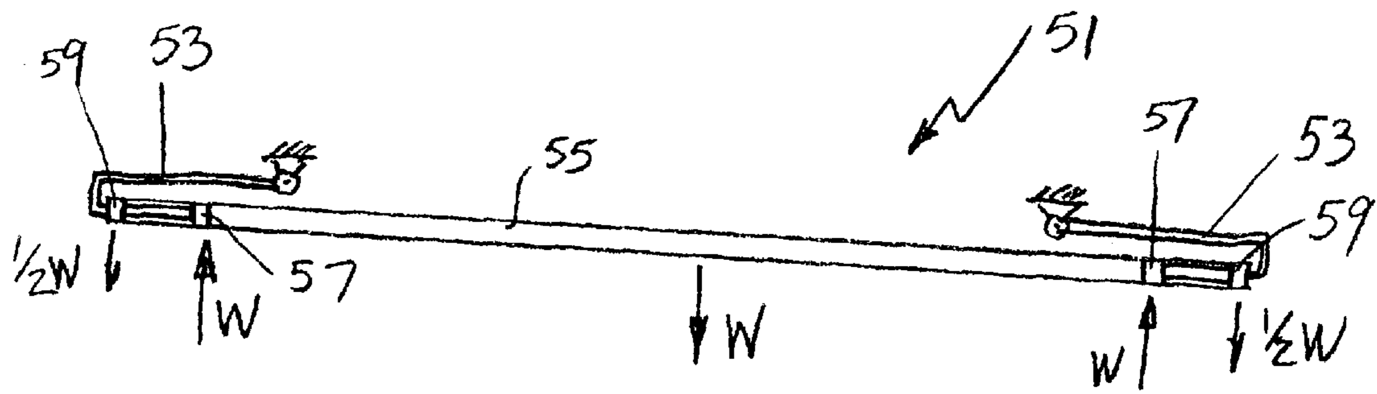
FIG. 10
