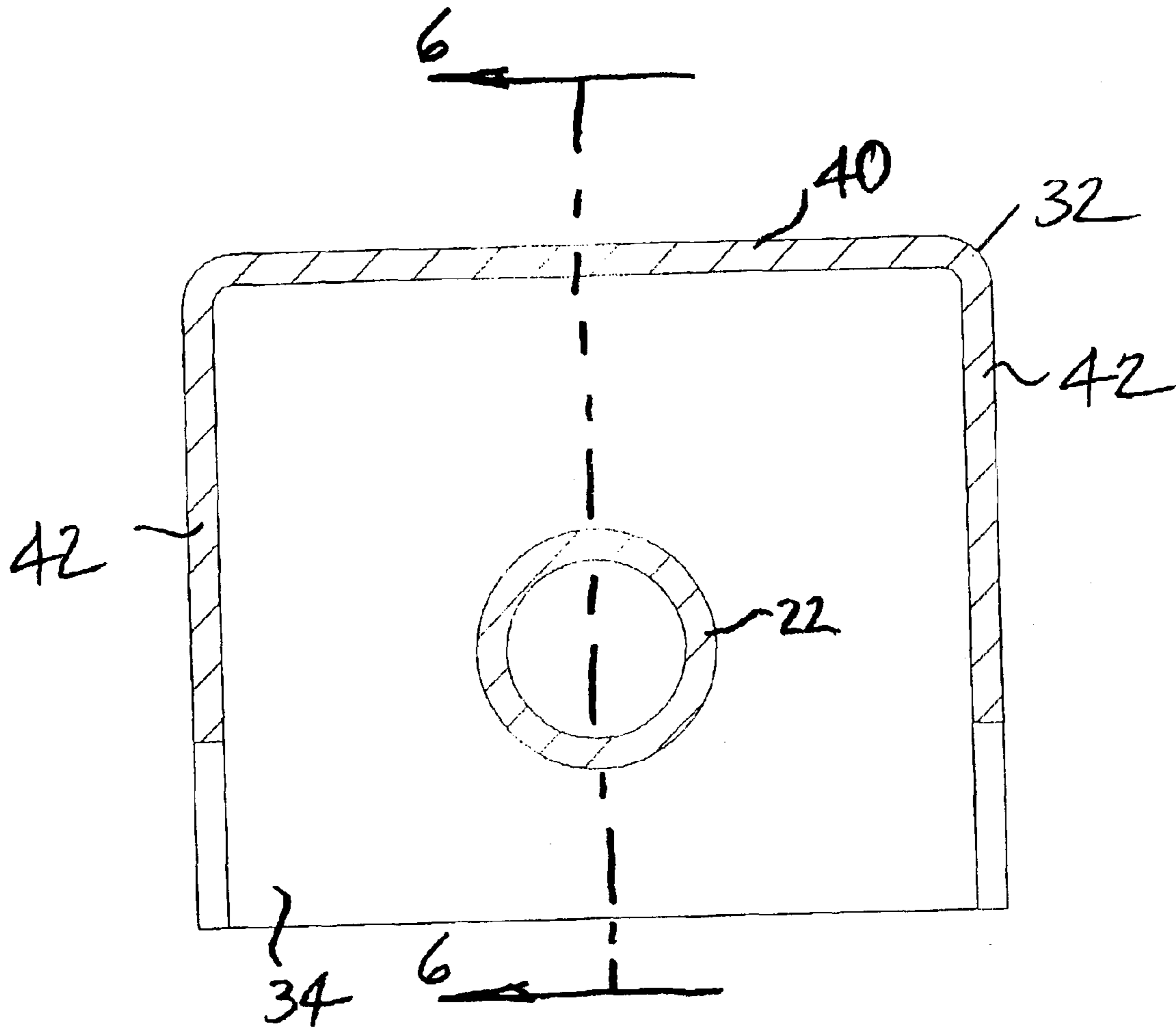
FIG. 5A
