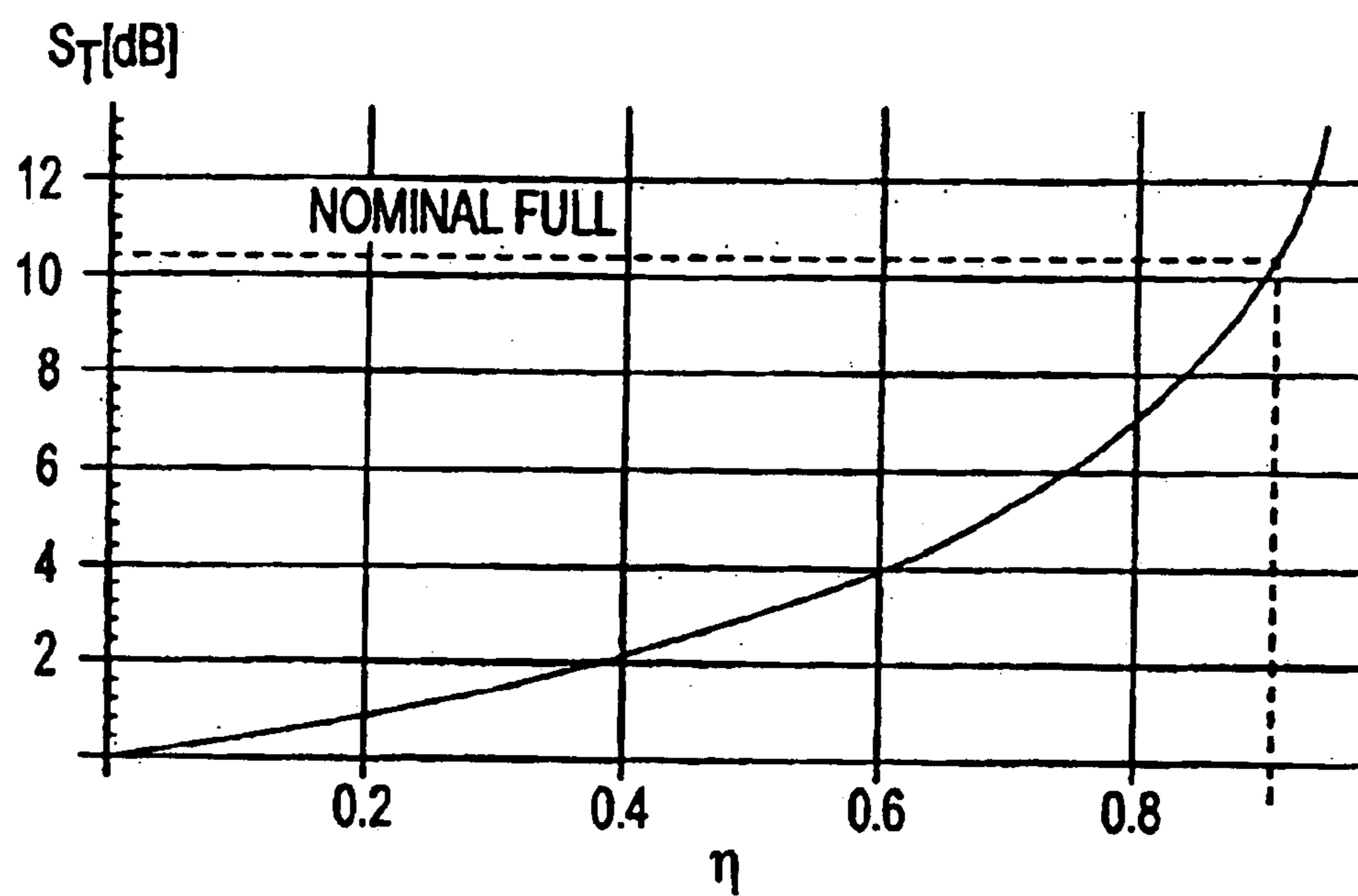
FIG. 17A
