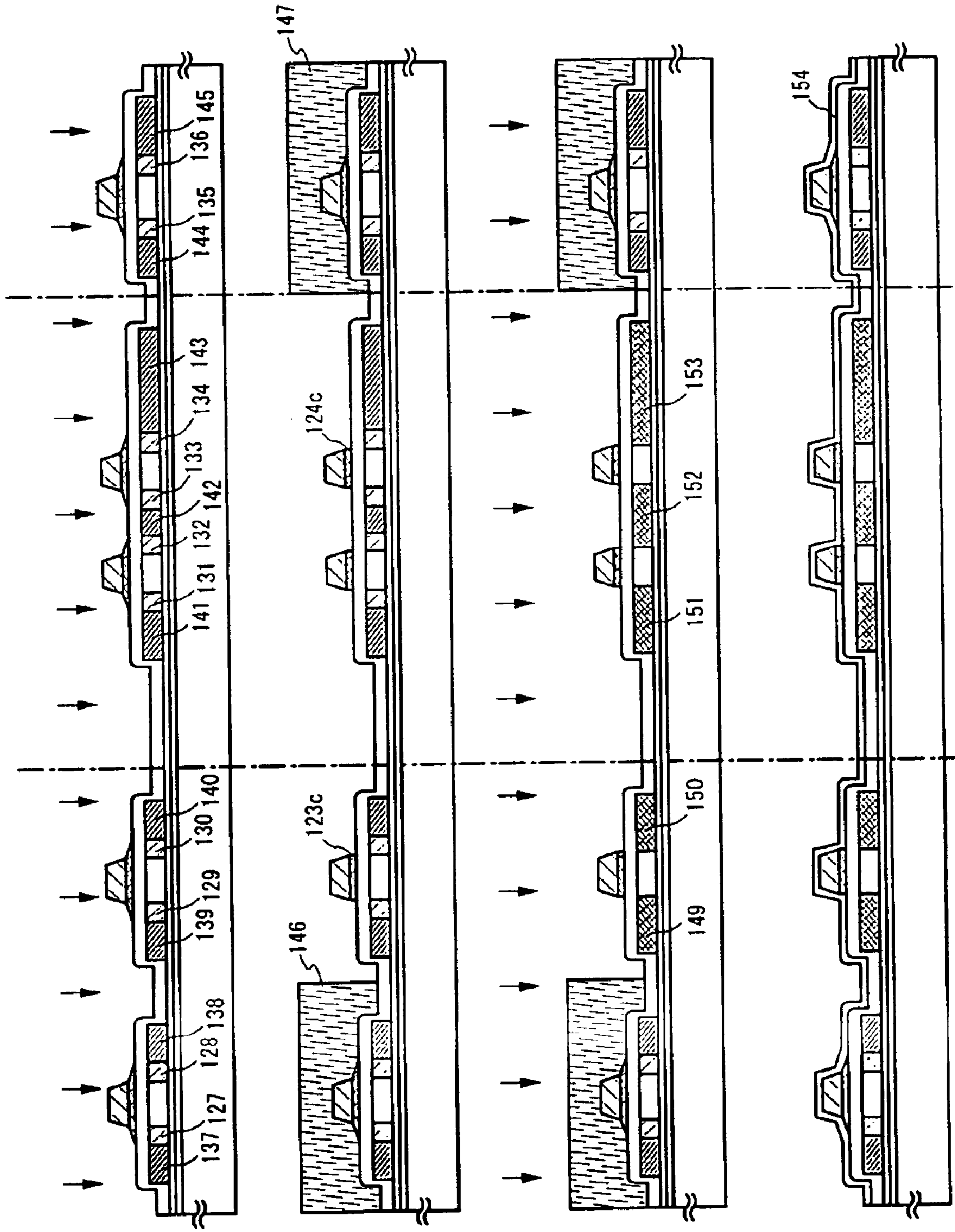
FIG. 2A
