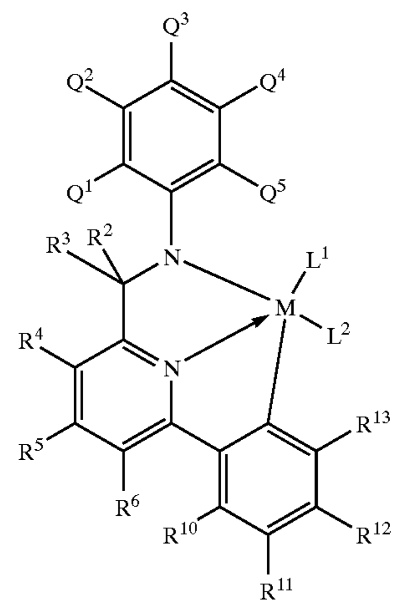
3,2 Complex
