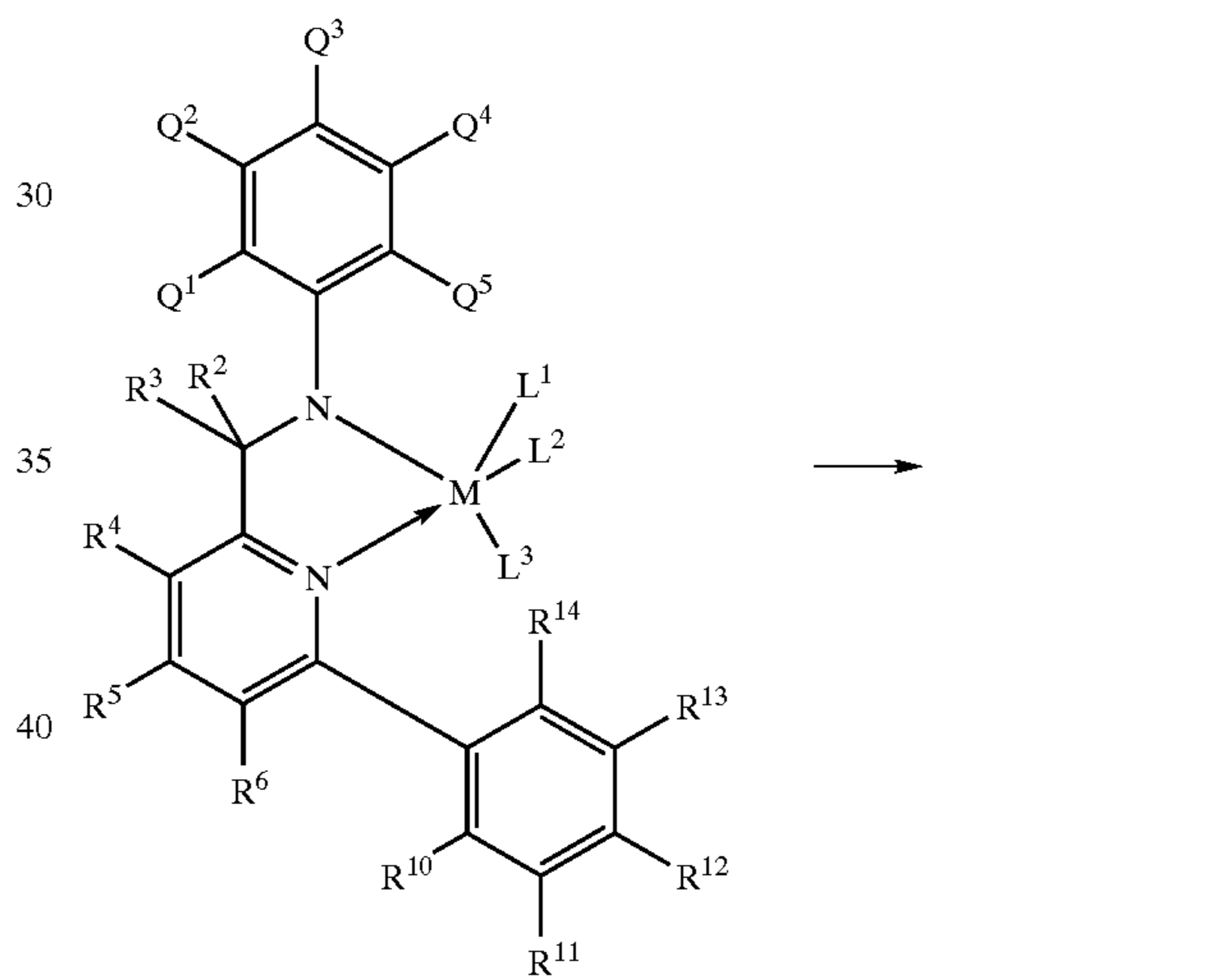
2,1 Complex
