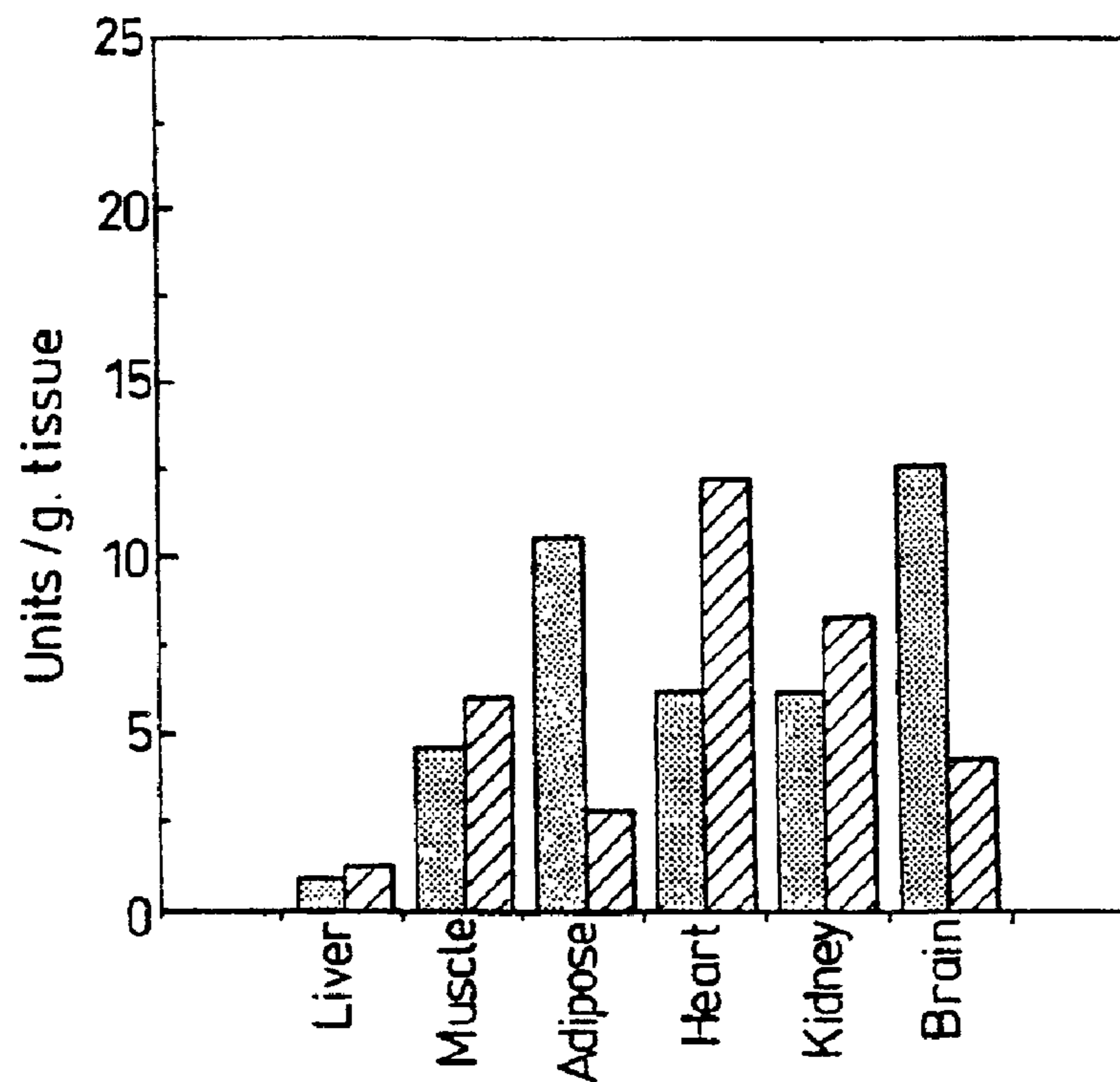
Fig. 4 (D) cAMP-dependent protein kinase-P assay
