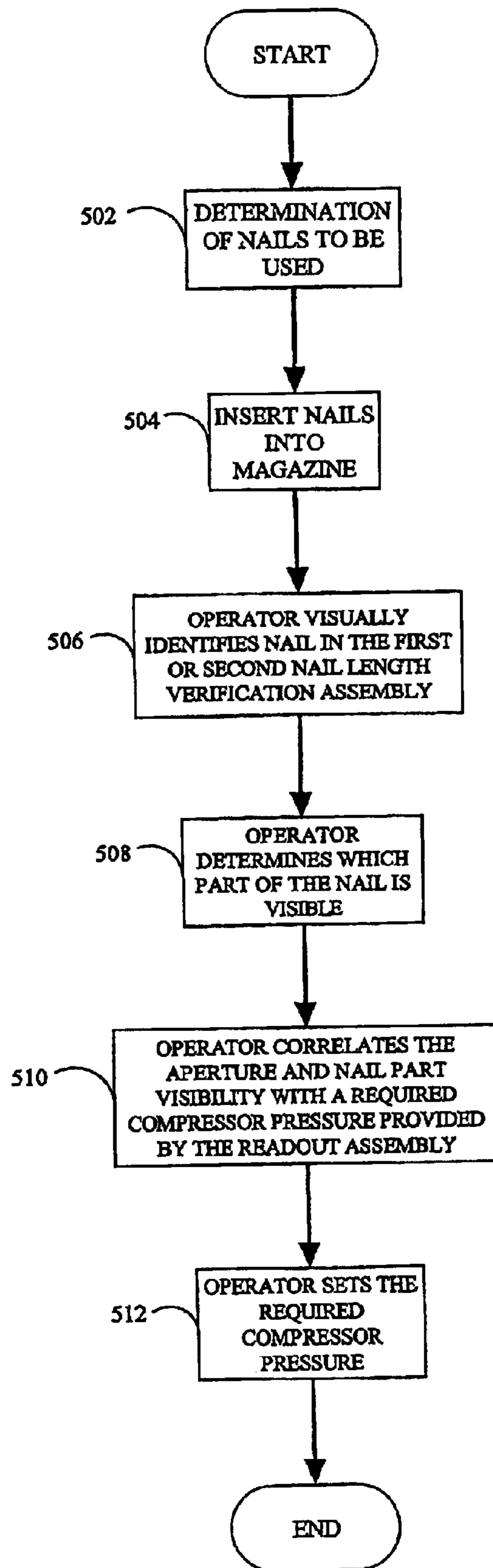
FIG. 5
