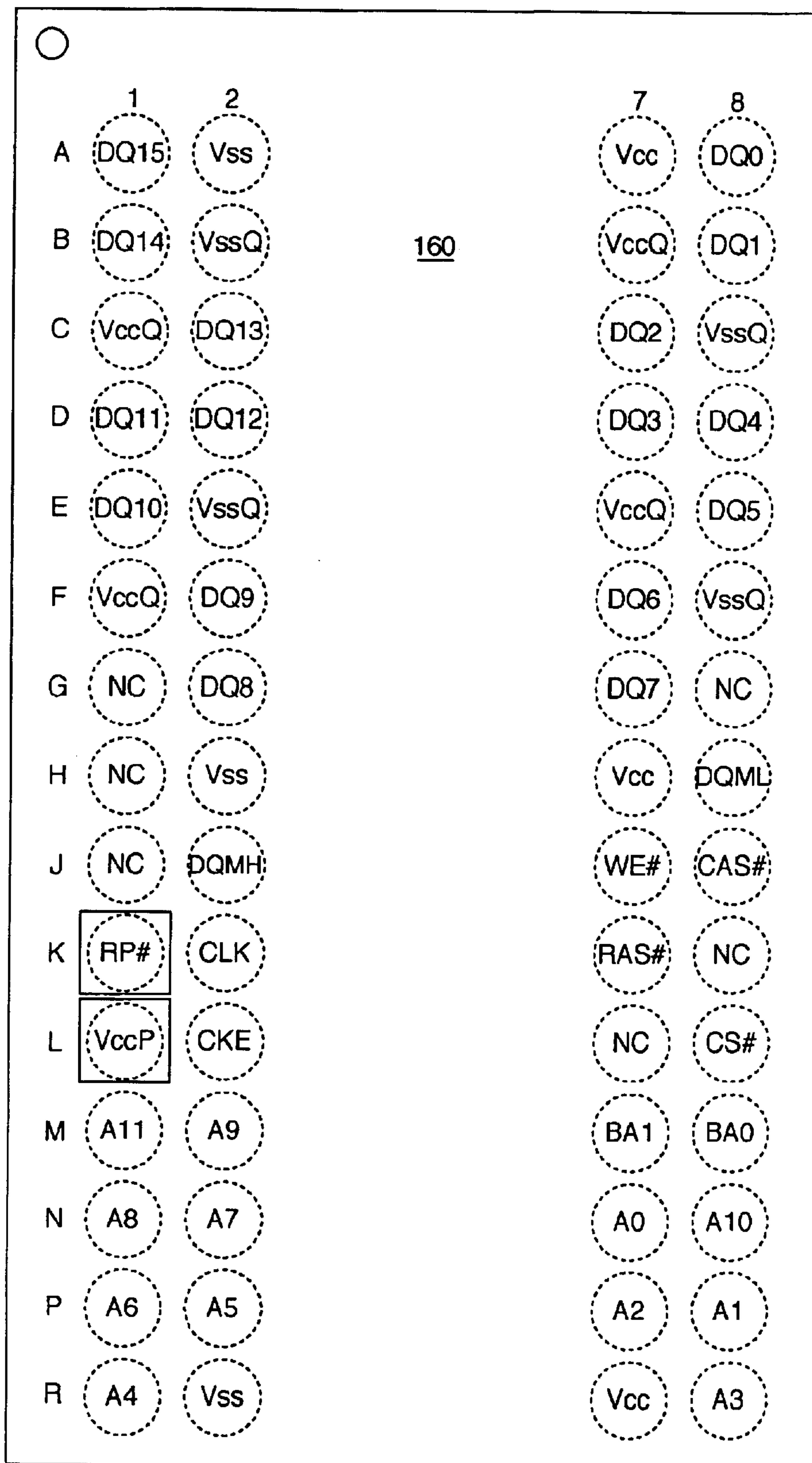
FIG. 1C
