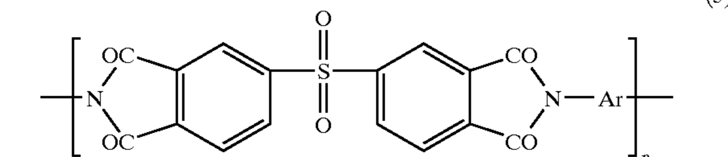
(DSDA polyimide)
