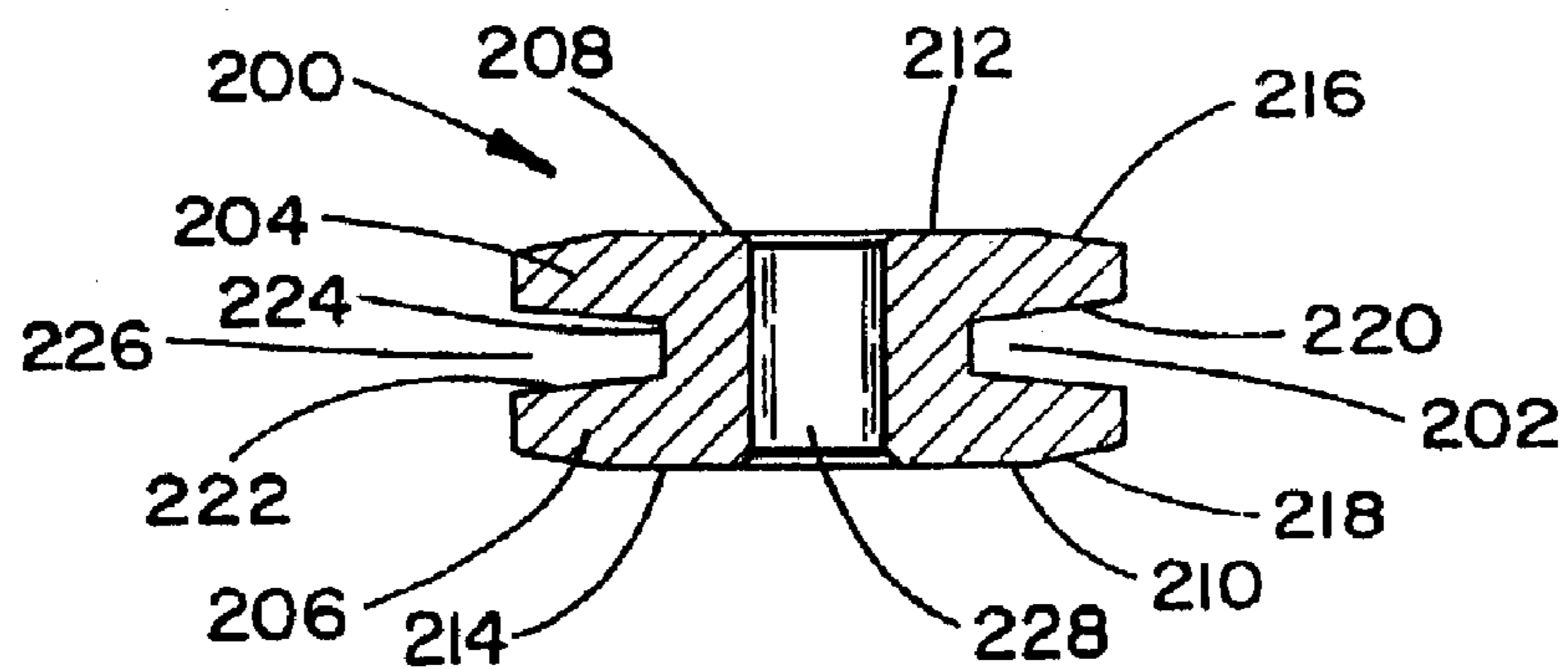
Section A-A
