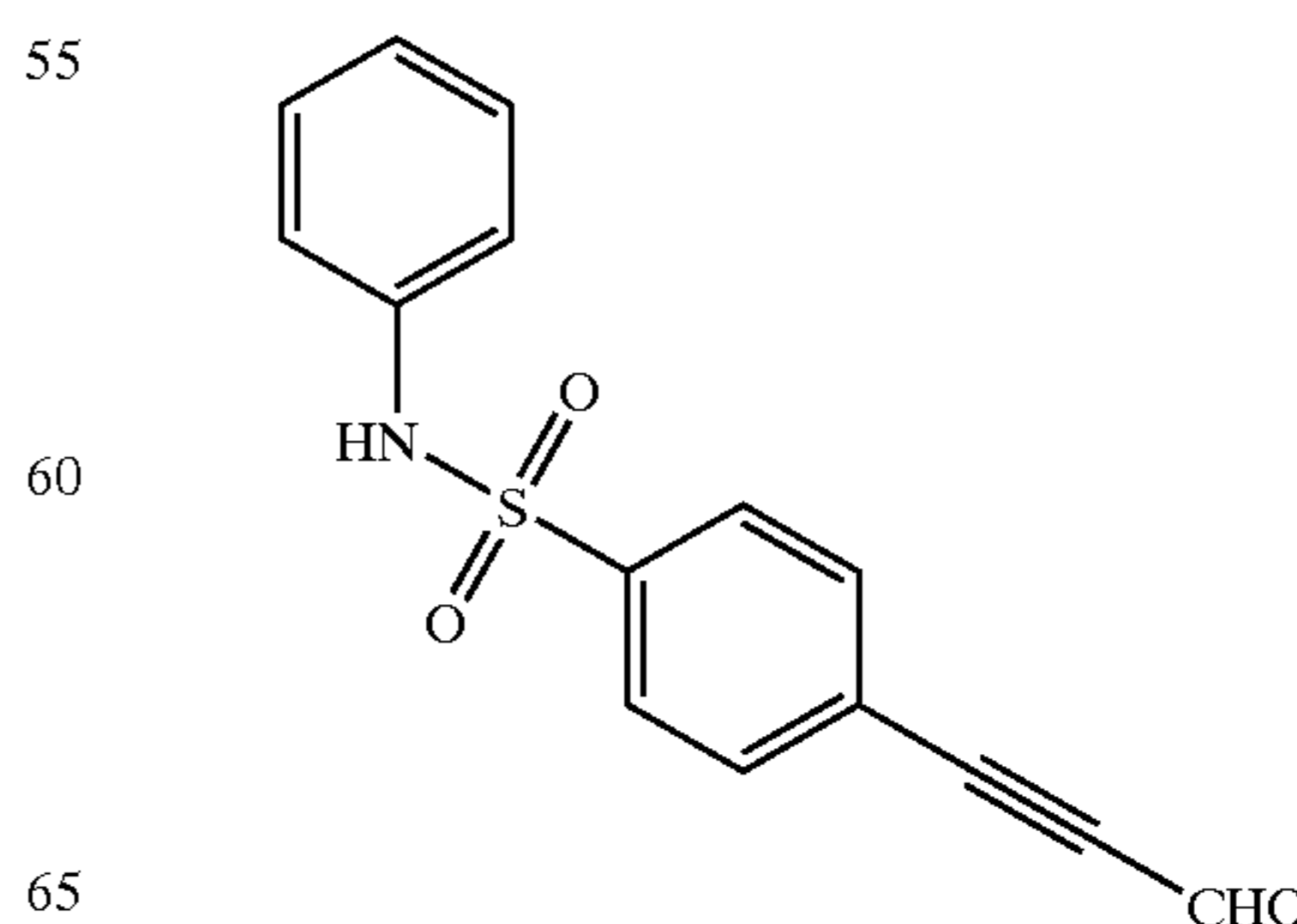
4-(3-Oxoprop-1-ynyl)-N-phenylbenzenesulfonamide (54b)
