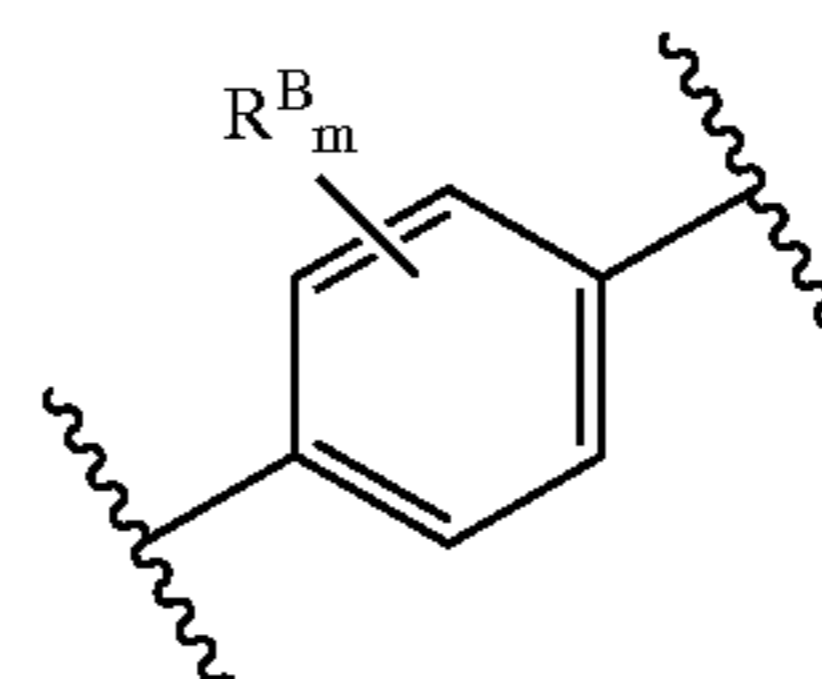
para
